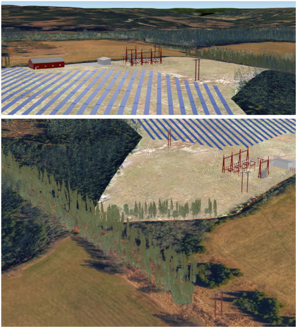
Figur 1: Illustrasjon av koblingsanlegg i Seval Skog transformatorstasjon. Kilde: Energeia og Elvias søknad av 18.04.2025.
