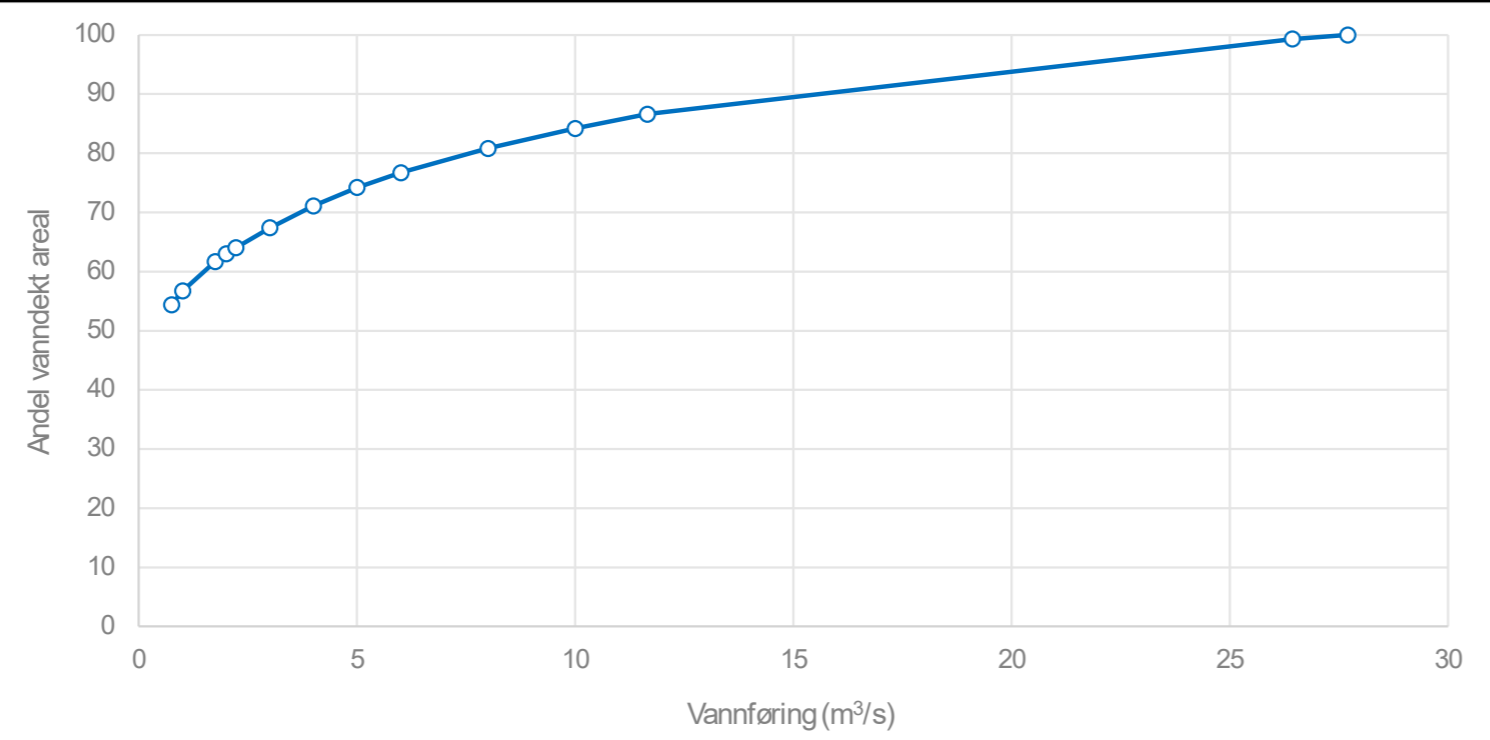
Restareal (%) etter utbygging, sett ift. totalt areal på strekningen Breimsvatnet - Teitafossen
