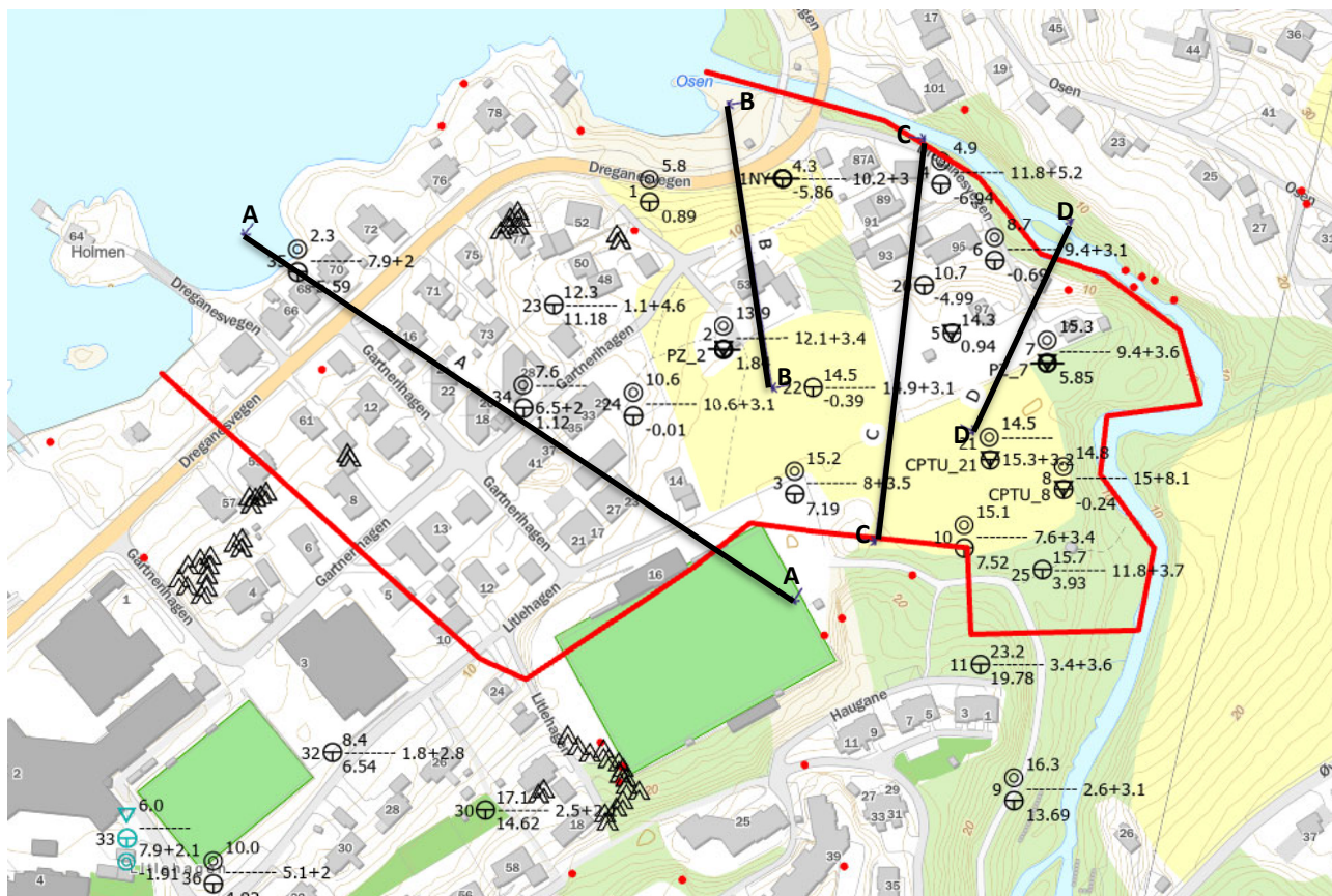
Figur 7-4: Mulig løsnakeområde (markert med rødt) basert på 15 \times skråningshøyden H . Innmålt berg i dagen er markert med \blacktriangle . Rosa prikker viser ca plassering av berg i dagen. Vurderte kritiske snitt innenfor mulig løsnakeområde er markert.
