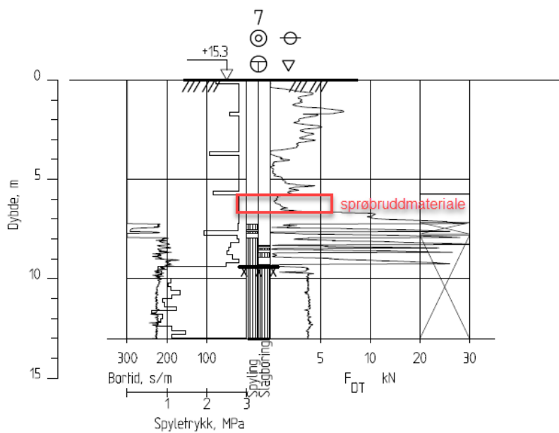
Figur 7-7: Totalsondering i BP 7. Prøvetaking viser at det er et lag med sprøbruddmateriale fra 6,0-6,5 m dybde.
