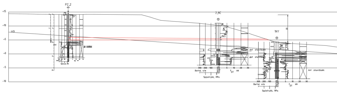
Figur 7-6: Profil B-B med totalsonderinger. Tolkning av laget med sprøbruddmateriale er markert med rødt. Linje med helning 1:15 som starter 0,25 \cdot H under skråningsfot, er vist på tegningen.
