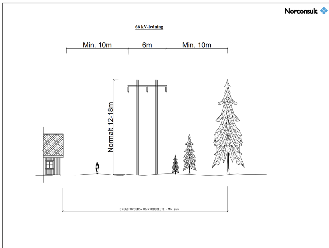
Figur 2: Mastene som planlegges brukt på strekningen Vrangfoss-Holla er i aluminium, har en høyde på 12-18 meter og krever et ryddebelt på 26 meter. Kilde: Lede sin konsesjonssøknad av januar 2026.
