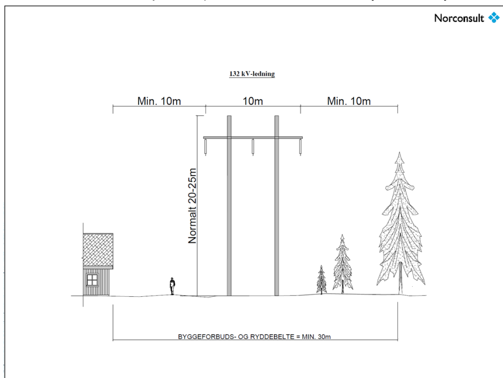
Figur 3: Mastene som planlegges brukt på strekningen Vrangfoss-Gvarv er i aluminium, har en høyde på 20-25 meter og krever et ryddebelt på 30 meter. Kilde: Lede sin konsesjonssøknad av januar 2026
