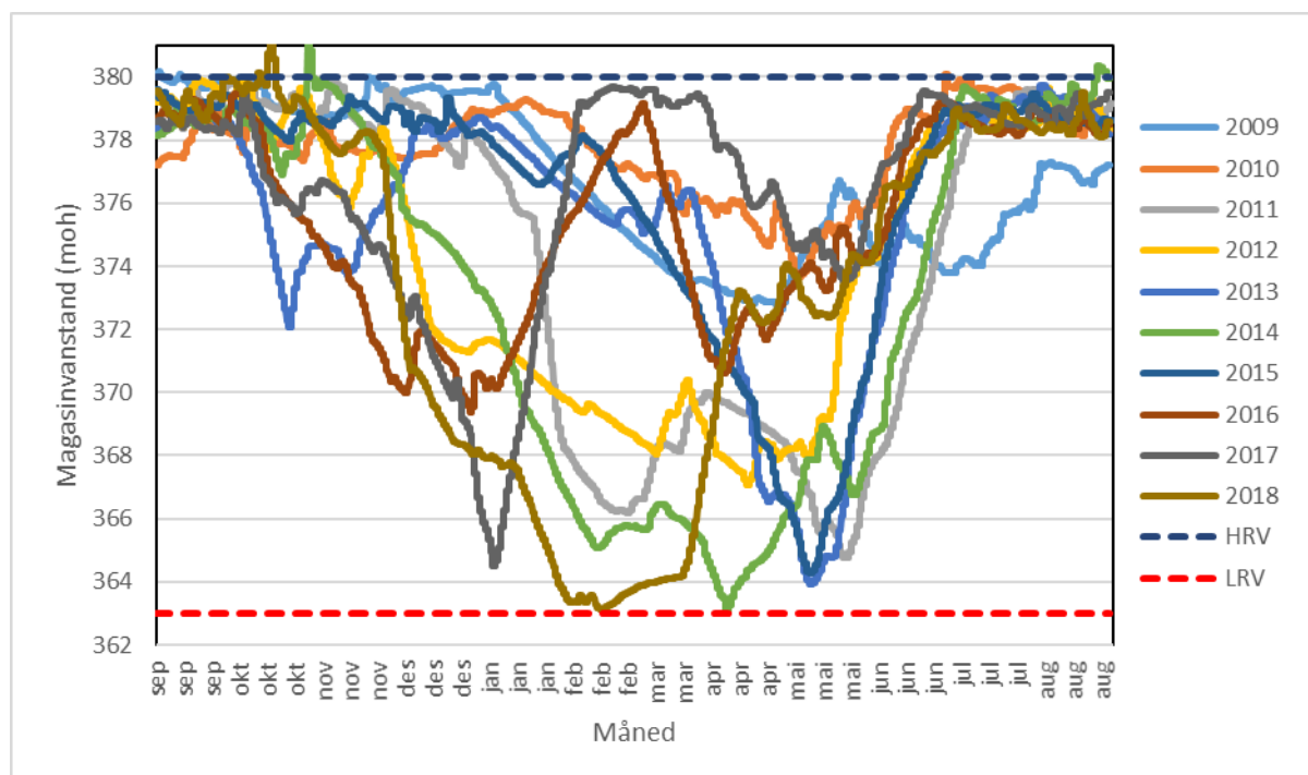
Figur 2-56 Vannstander i Røldalsvatnet over året (september – august) for de siste 10 årene (Figur: Hydro).
