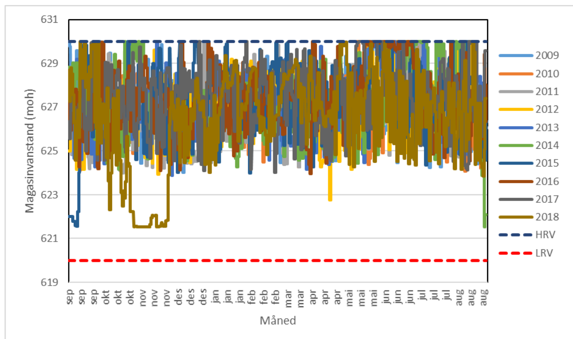
Figur 2-62 Vannstander i Kvanndalsfoss over året (september – august) for de siste 10 årene (Kilde: Hydro). Magasinet er inntaksmagasin for Suldal II kraftverk og kjøringen av kraftverket medfører variasjoner i vannstanden over korte tidsrom.
