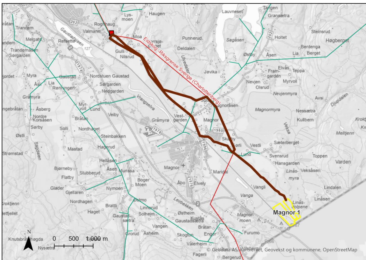
Figur 2-5: Alternative tilknytningstraseer for solkraftverket vist i NVE kart. Forslag til 22 kV tilknytningstraséer er vist med brun linje.
