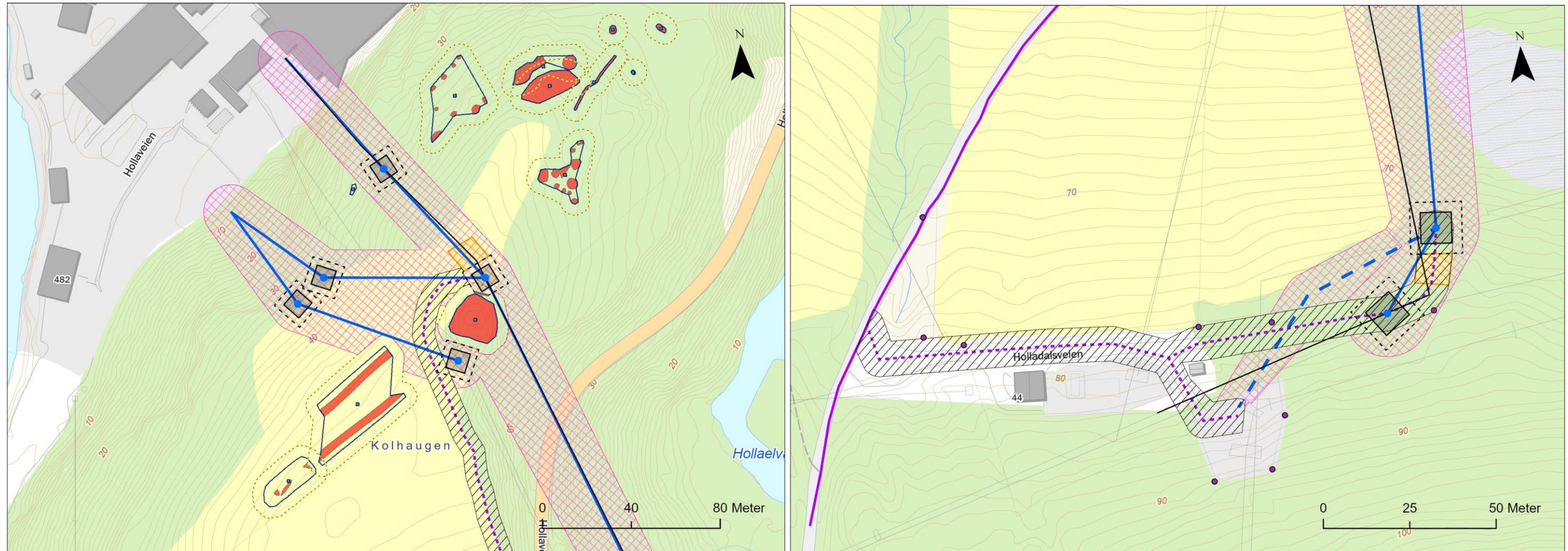
Til venstre: Nærmere kart med oversikt over planlagt inngrep sør i traseen ved Holla transformatorstasjon. Til høyre: Oversikt over inngrepet nord i traseen mot Holla smelteverk.
