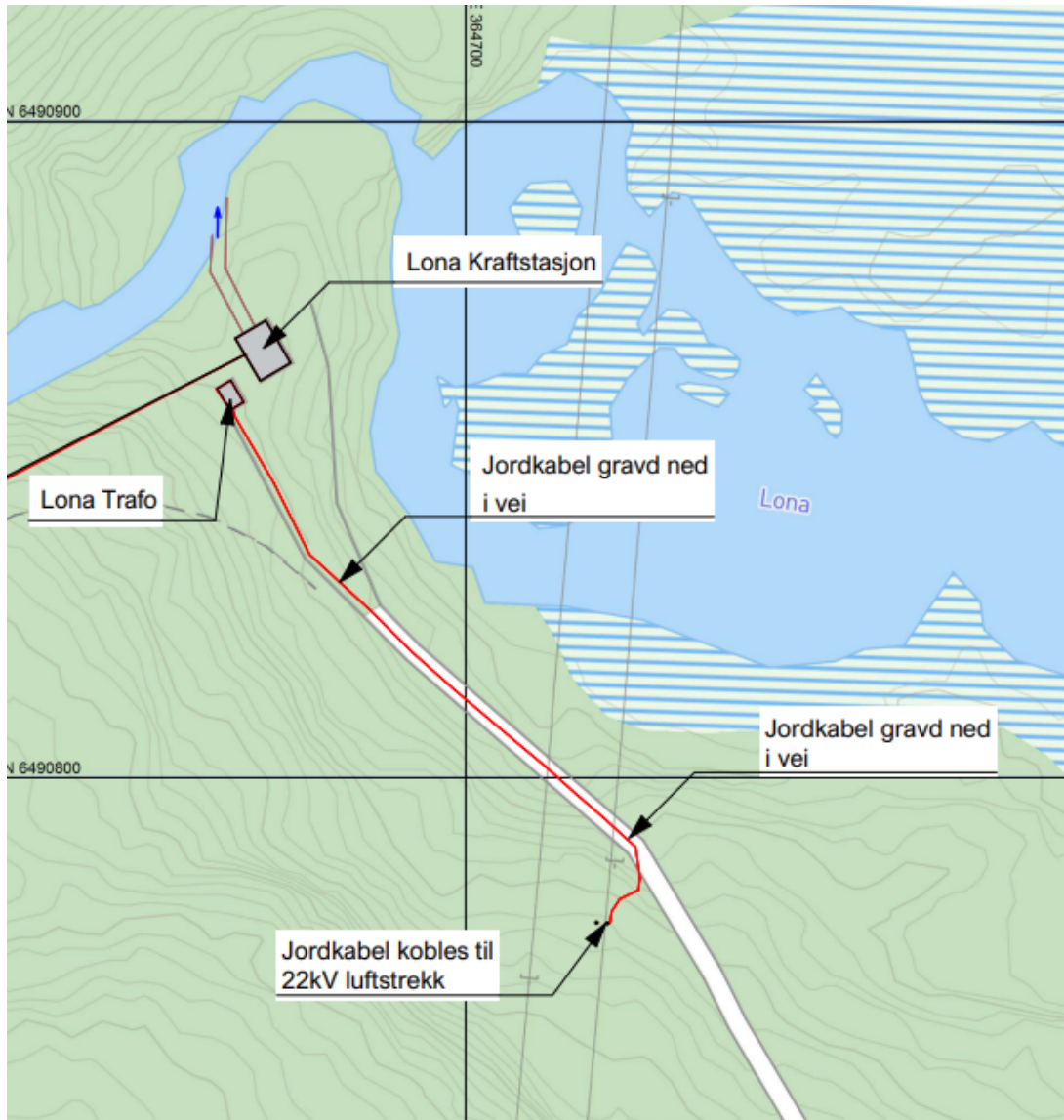
Figur 1: Jordkabelen er markert i rødt. Kilde: Lona kraftverk sin søknad av mars 2025.
