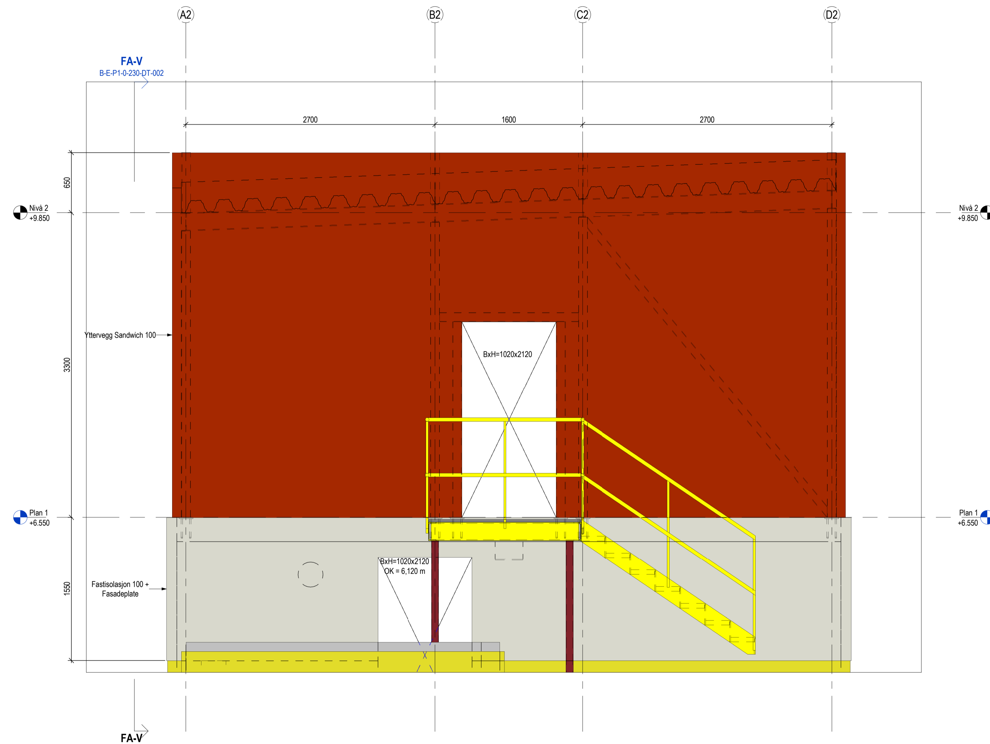
Fasade Sør 1:25
