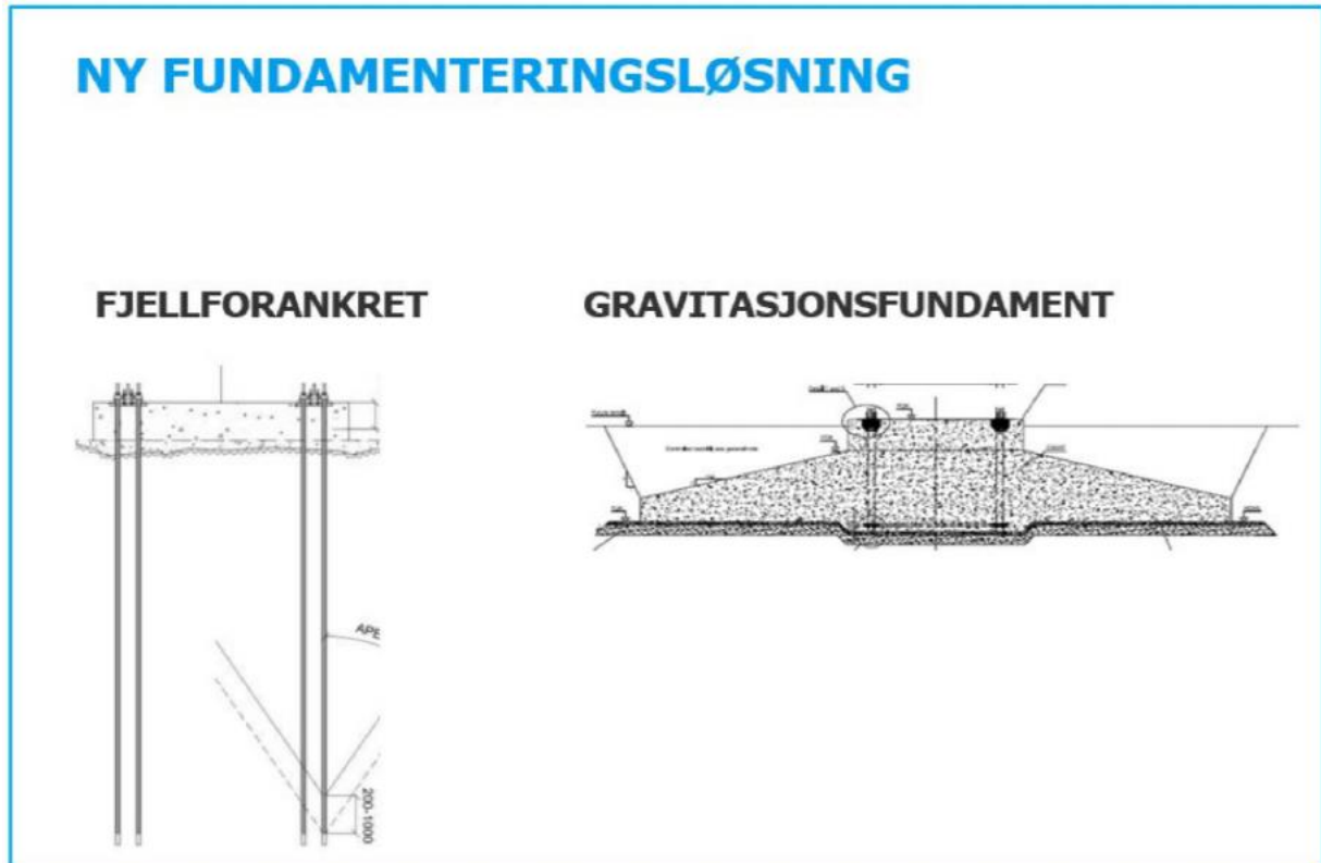
Figur 2: Tverrprofil av fjellforankra fundament og gravitasjonsfundament.
