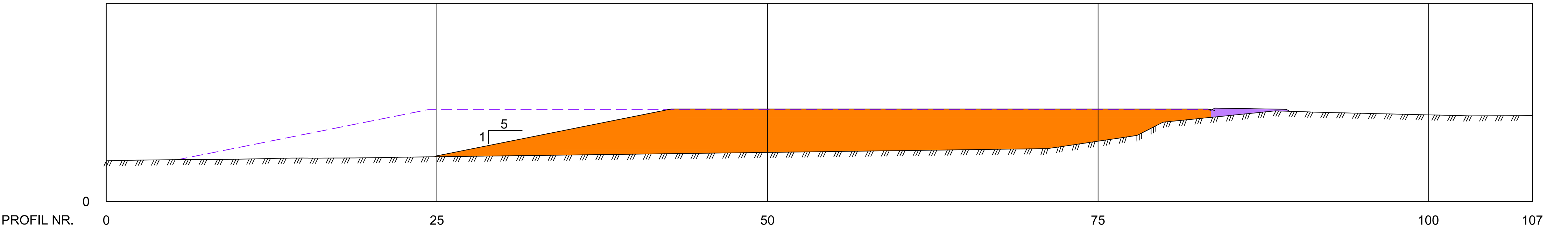
SNITT A-A 1:200
