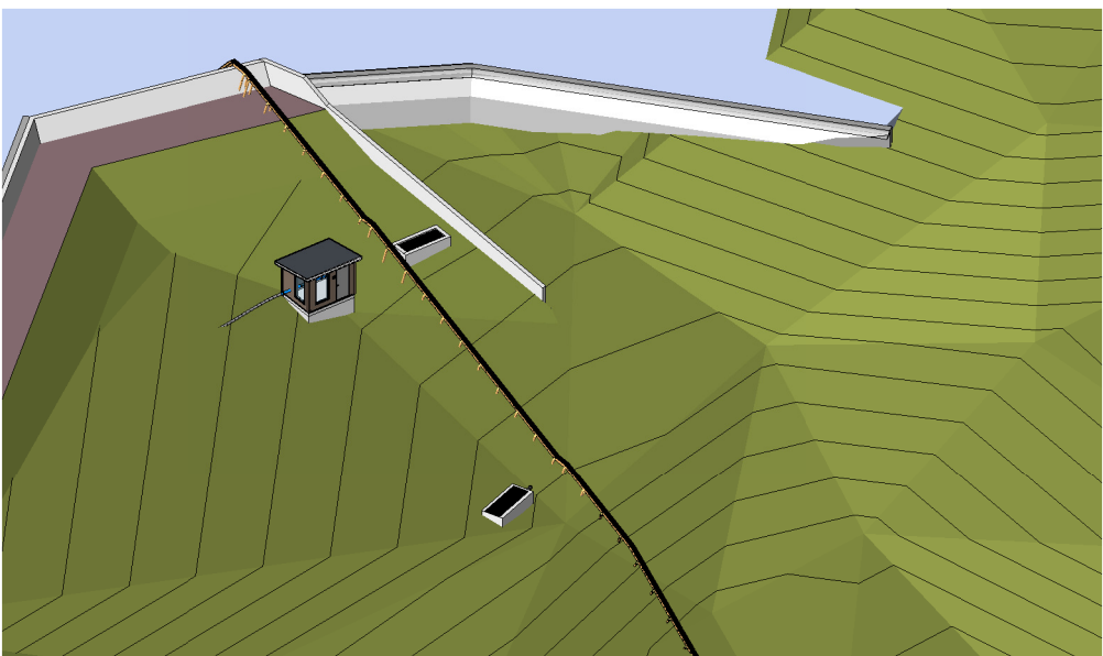
3D overløp, lukehus og ål arrangement
