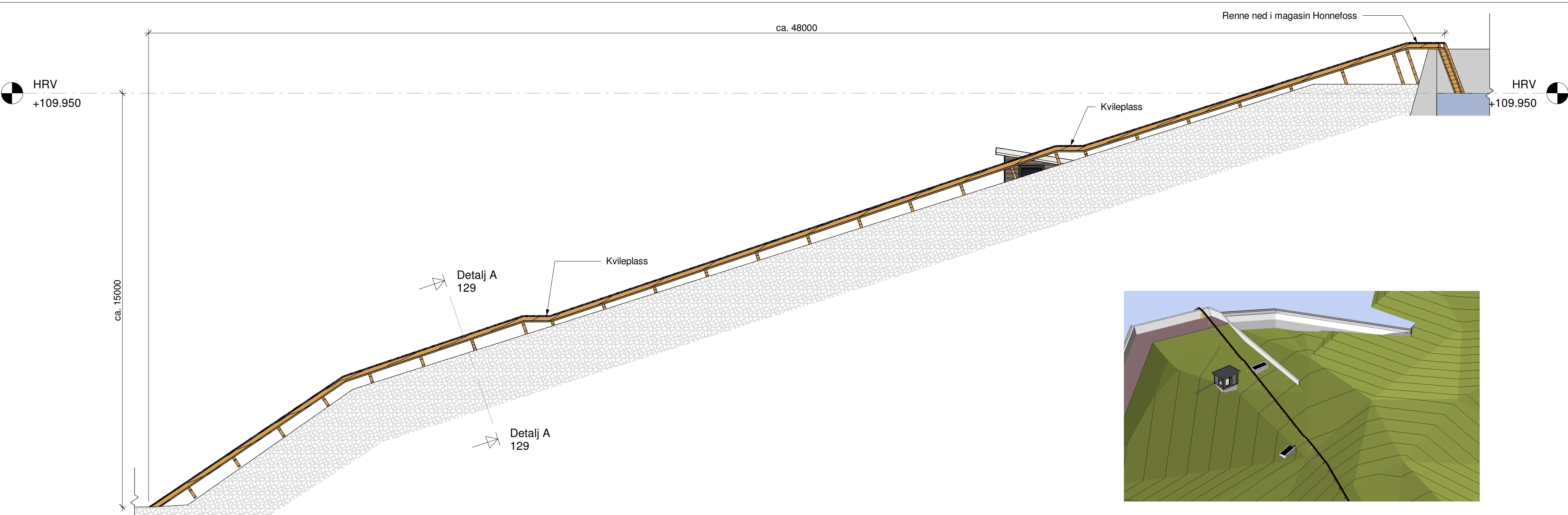
Snitt Ål renne 1 : 100
