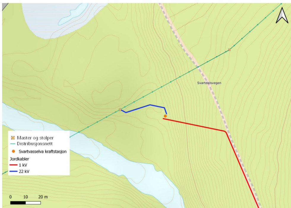
Figur 2: Jordkabeltraseer for Svartvassselva kraftverk. 22 kV-jordkabelen er markert i blått og 1 kV-jordkabelen er markert i rødt. Svartvassselva kraftstasjon er markert som oransje prikk. Kilde: Småkraft sin søknad av mars 2025.
