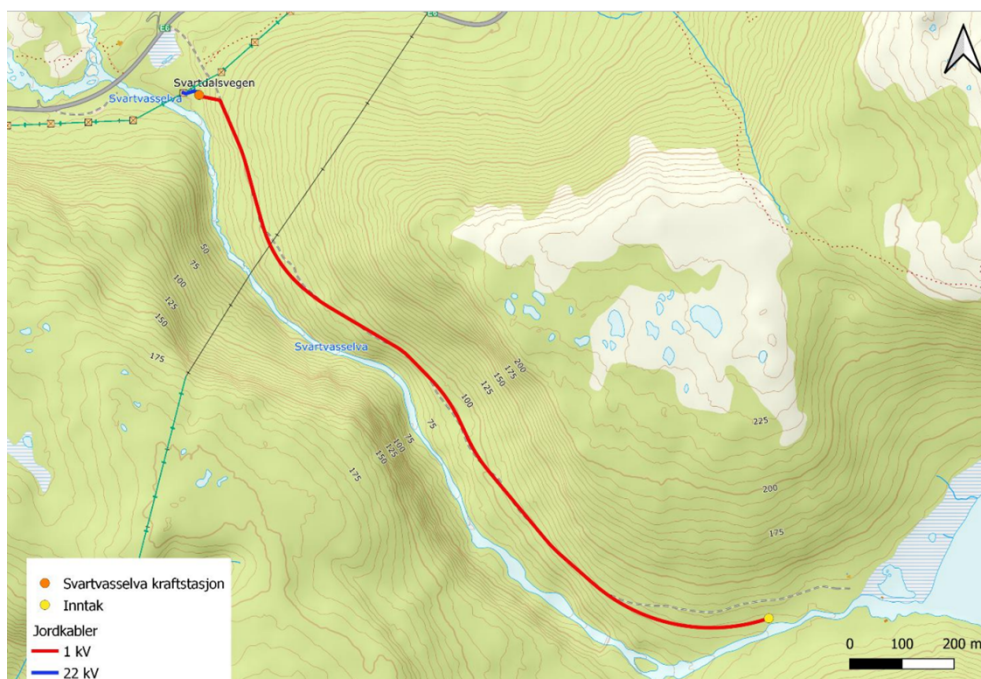
Figur 1: Kabeltraseer for Svartvassselva kraftverk. 22 kV jordkabel er markert i blått, mens 1 kV trasé er markert i rødt. Kilde: Småkraft sin søknad av mars 2025
