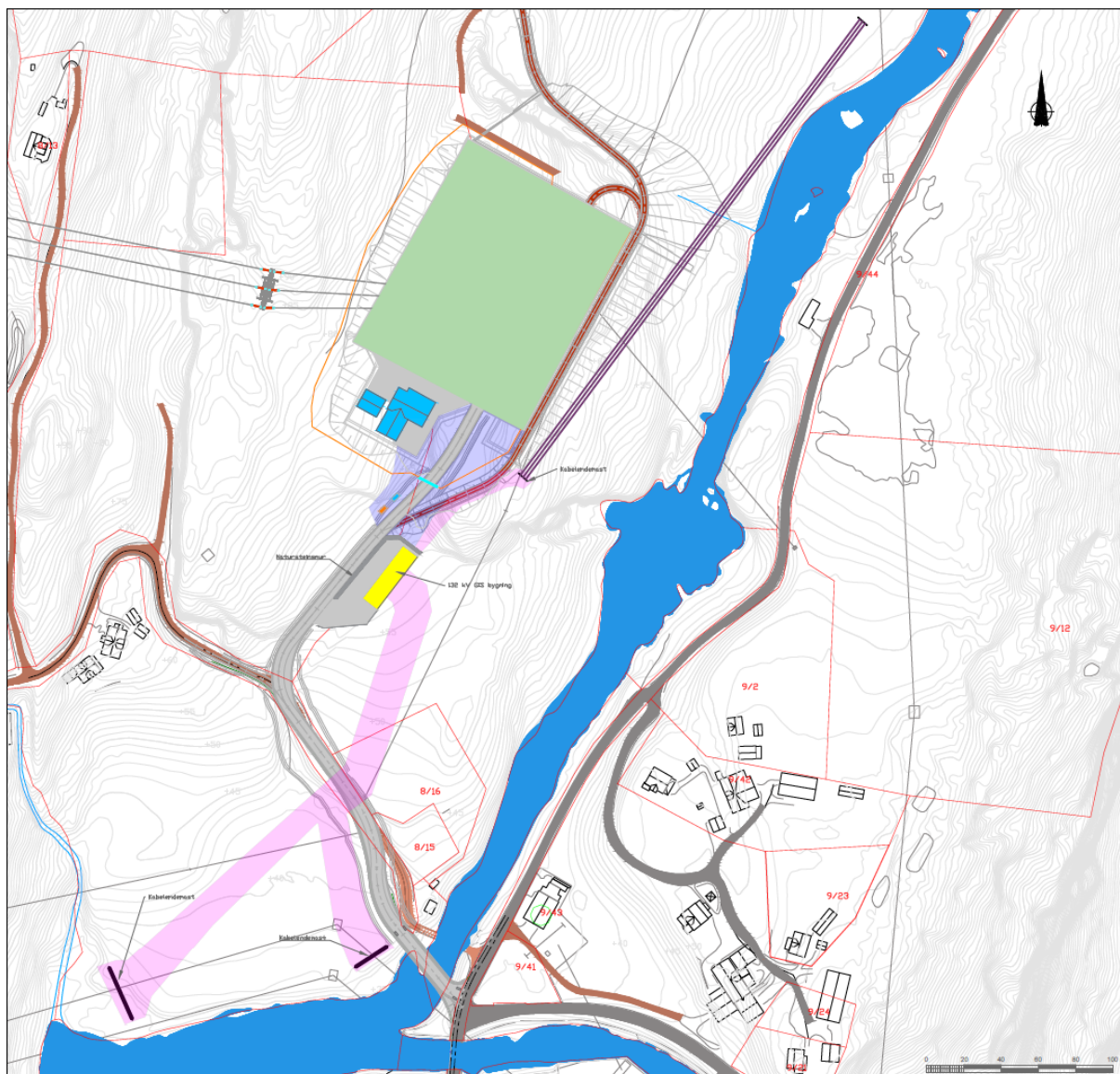
Kart 1: 132 kV jordkabel fra kabelendemast mot Fortun transformatorstasjon ved brua i sør, til Jamnene koblingsstasjon, vist med rosa felt.
