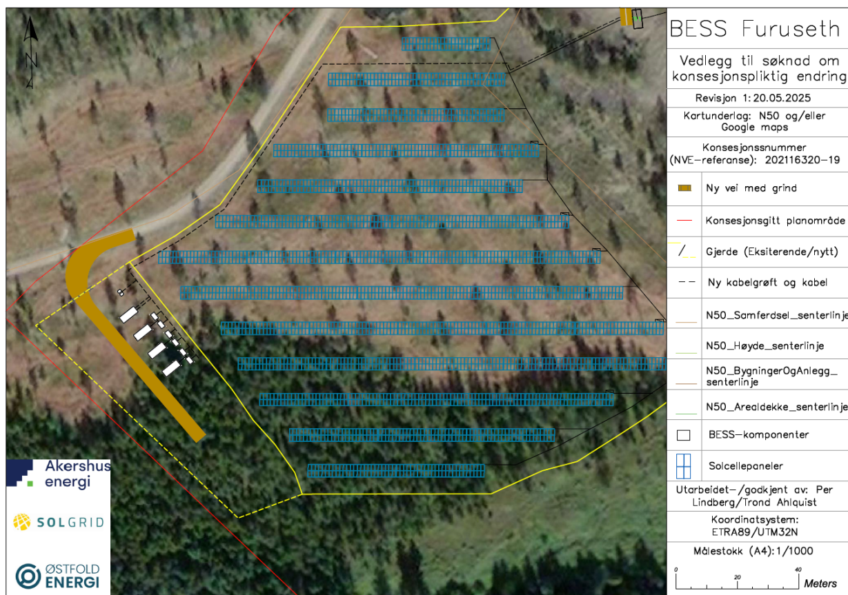
Figur 1: Kartet viser plassering av batterianlegg og anleggsvei i planområdet for Furuseth solkraftverk.
