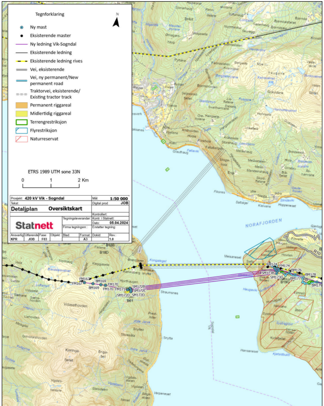
Figur 1: Utsnitt av Statnetts oversiktskart av 5. april 2024. Eksisterende fjordspenn som skal rives vises med gul og sort stiptet linje, mens nytt vises med lilla linjer.
