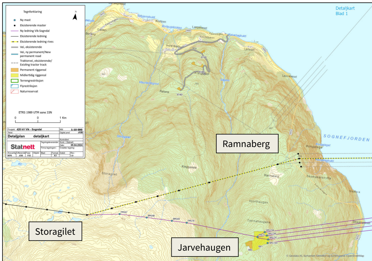
Figur 2: Statnetts detaljplankart av 5. april 2024. Kartet viser riggareal for bygging av det nye fjodspennet på Jarvehaugen, ny trasé i lilla opp mot Storagilet. Eksisterende ledning og master på Ramnaberget og mot Storagilet skal rives når den nye ledningen er bygget.
