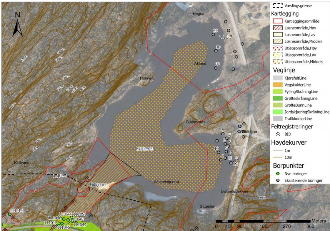
Figur 6-11: Opptegnet løsne- og utløpsområde for faresonen Eidskjerrret.
