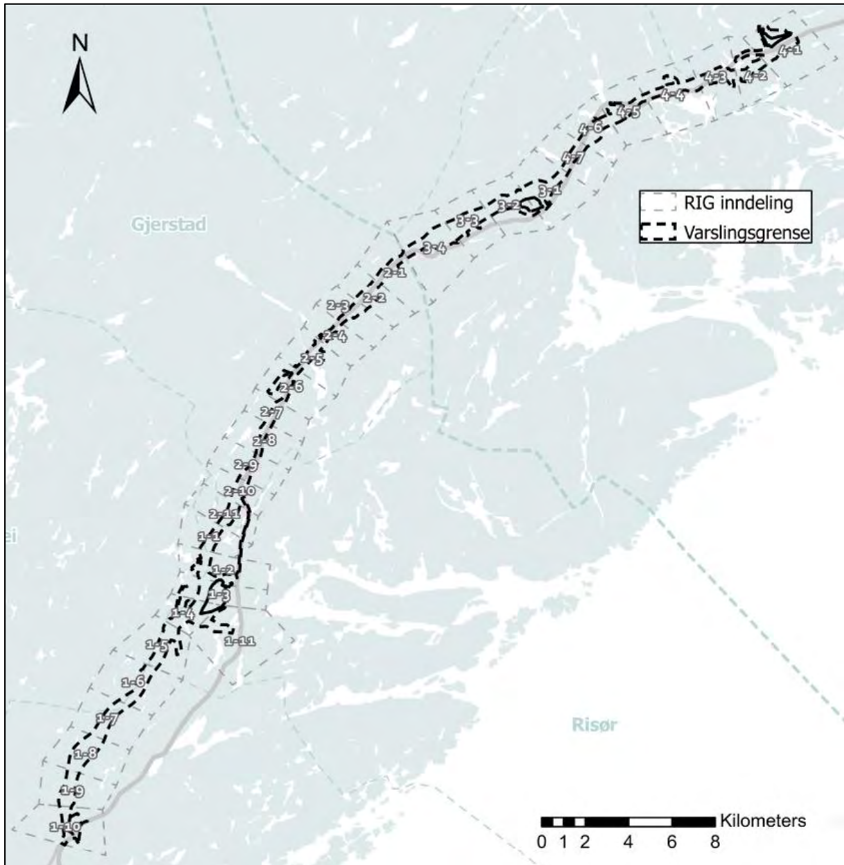
Figur 3-1: Oversiktskart som viser den geotekniske inndelingen (RIG-inndeling) av varslingsområdet.
