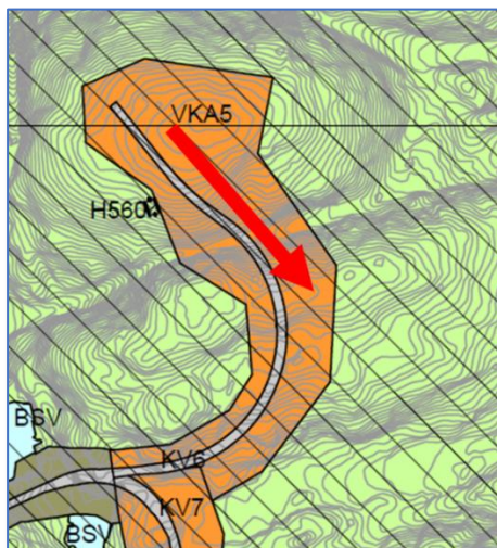
Figur 3 Altrnativ plassering av mølle VKA5
