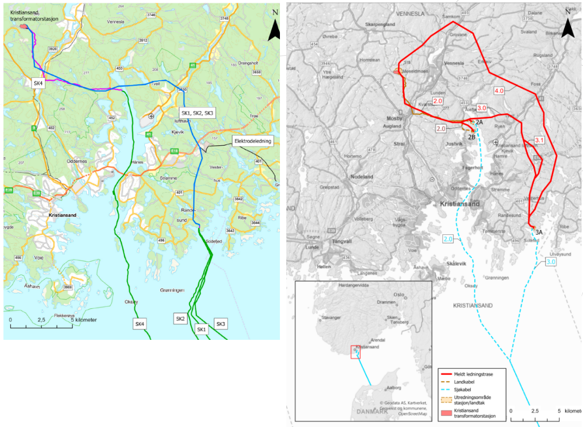
Figur 1: Kart som viser eksisterende strømkabler til Danmark (til venstre) og kart som viser traseer som Statnett foreslår å utrede. Kilder: www.kystinfo.no og Statnett
