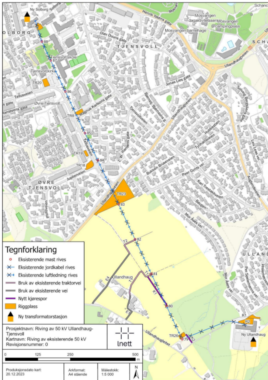
Figur 4: Oversikt over tiltaksområdet med riggplasser og anleggsveier for riving av Tjensvoll - Ullandhaug 1 og 2. Kilde: Lnett sin konsesjonssøknad av desember 2023.
