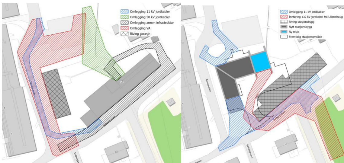
Figur 2: Utsnitt av kart som viser forberedende anleggsarbeid med omlegging av infrastruktur til venstre, og permanent kabelforlegning til høyre. Kilde: Lnett sin konsesjonssøknad av desember 2023.
