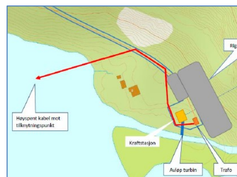
Figur 3: Kabeltrasé fra kraftverket til Sildhopvatnet.
