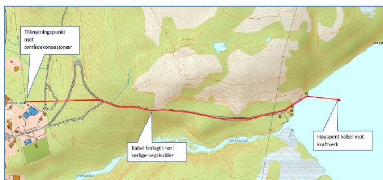
Figur 2: Kabeltrasé fra Sildhopvatnet til tilknytningspunkt ved Mørsvik skole.
