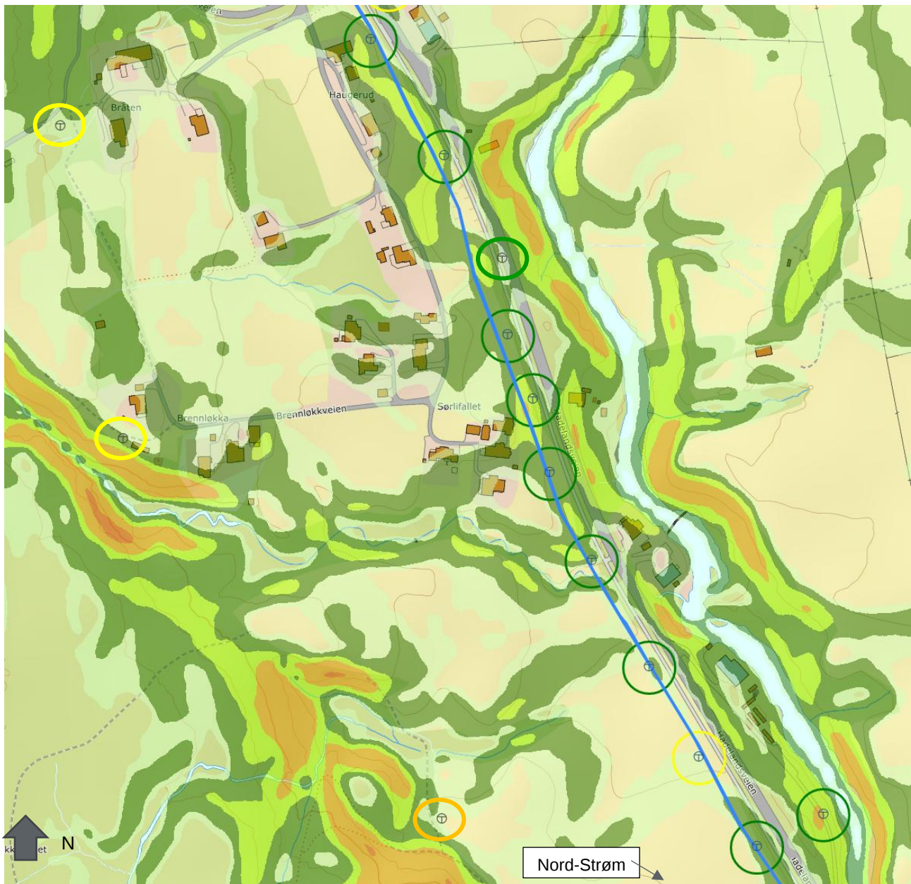
Figur 8 Oversiktsbilde med terrenghelning, borpunkt med tolket kvikkleire og skissert va-trase. Gul sirkel indikerer leire, oransje sirkel er antatt sprøbrudd og rød er påvist sprøbrudd. Grønn er enten påvist ikke sprøbrudd eller tolket å ikke inneholde leire..
