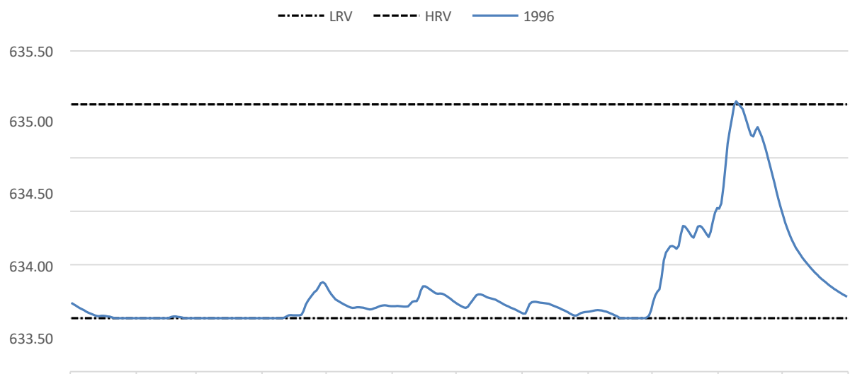
Fyllingskurve for Bjørnestadvatn (Tørt år 1996)
