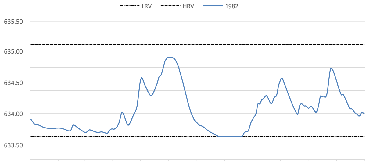
Fyllingskurve for Bjørnestadvatn (Middels år 1982)
