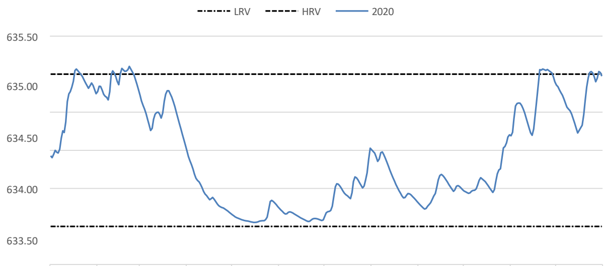
Fyllingskurve for Bjørnestadvatn (Vått år 2020)
