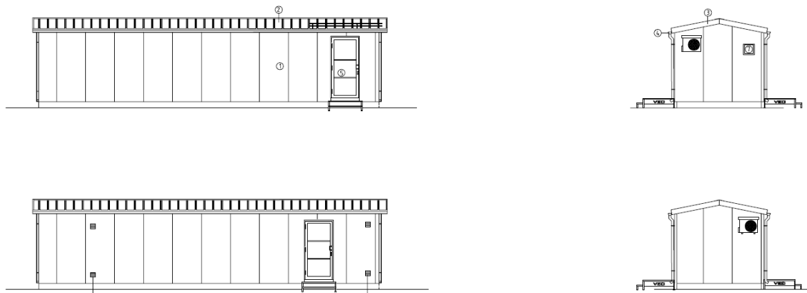
Figur 2: Utklipp fra fasadetegninger for transformatorstasjon. Komplet versjon er vedlagt.
