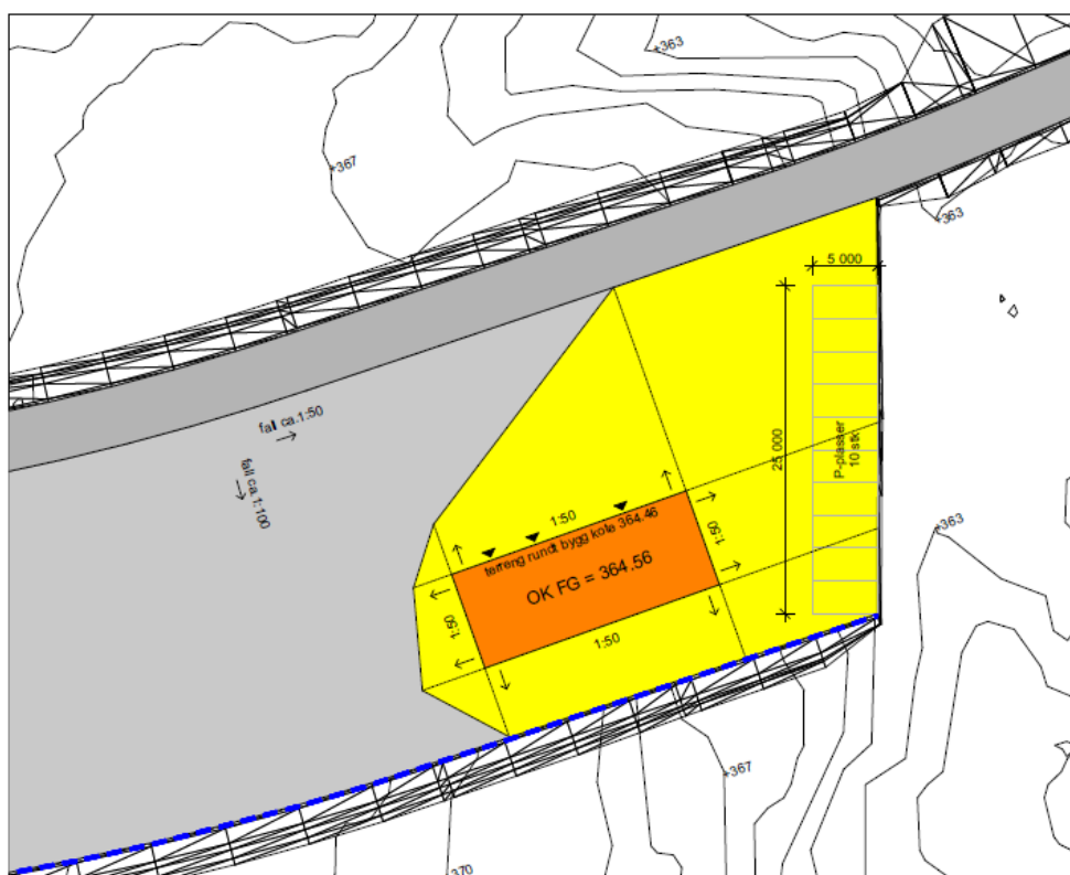
Figur 5: Utklipp fra søknad: utomhusplan for driftsbygg. Oransje: driftsbygg, gult: opparbeidet areal rundt bygg, grått: vei og istandsatt massetak. På sørsiden av bygget er det en skjæring i fjellet.
