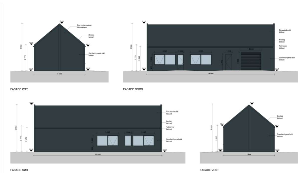
Figur 1: Utklipp fra fasadetegninger for driftsbygg. Komplet versjon er vedlagt.
