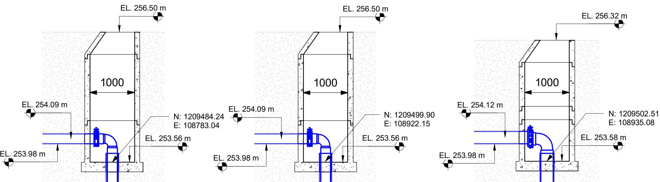
SECTION TB1 1 : 50
