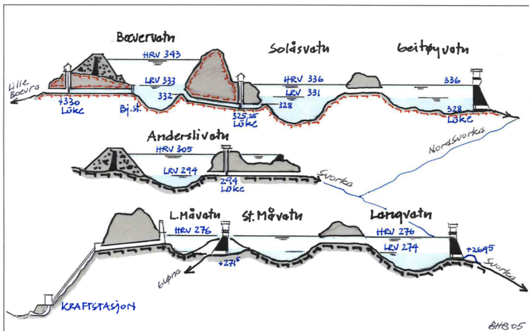
Figur 1. Revurdering 2005 Svorka kraftverk – skjematisk snitt vannveier. Referanse: Statkraft Energi
