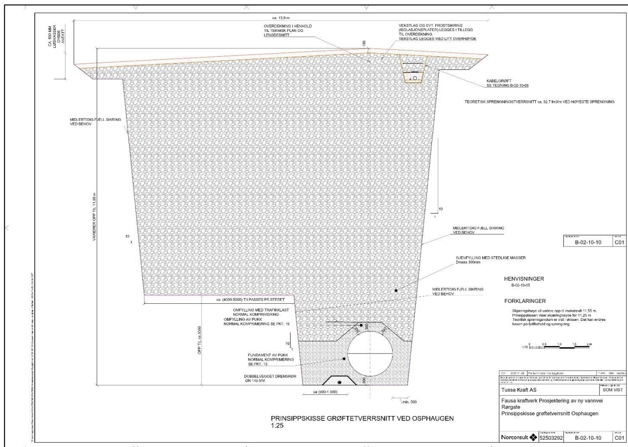
Figur 3-19: Skisse, grøftetverrsnitt ved Osphaugane.
