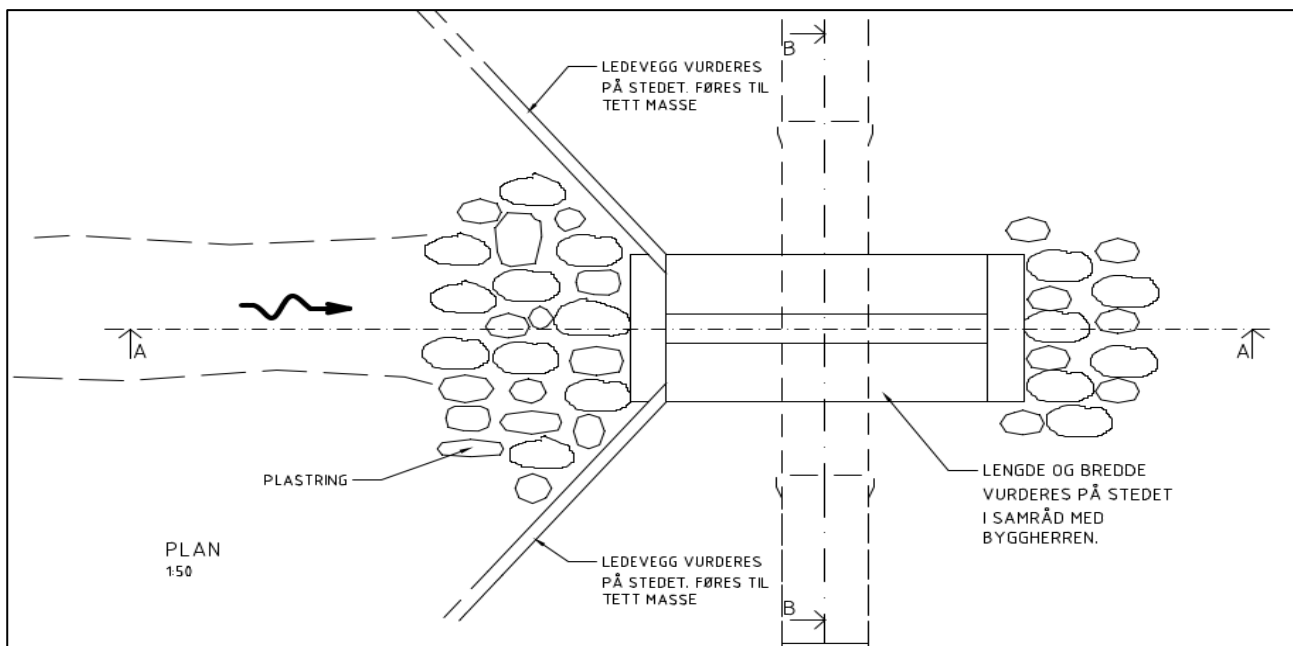
Figur 3-24: Plantegning av planlagte bekkekryssninger.
