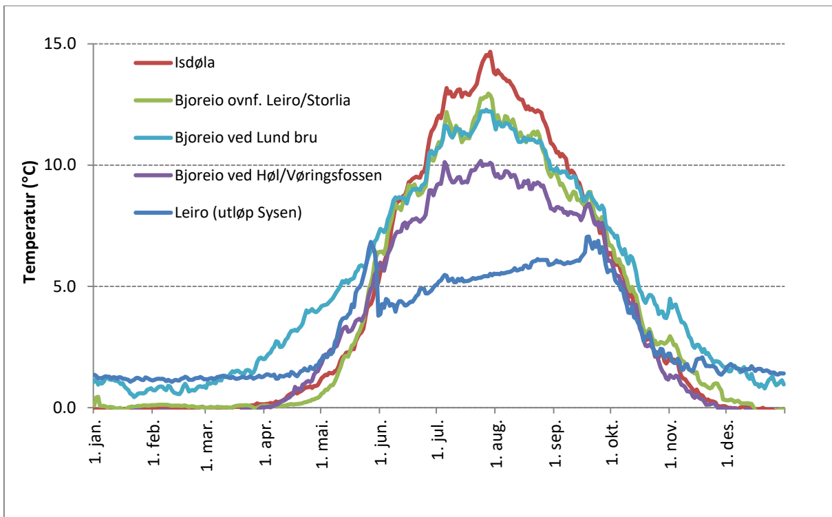
Figur 2. Vanntemperatur (døgnmiddel) for perioden 2001-2019 med tilgjengelige data fra Isdøla, Bjoreio ovenfor Leiro (utløp Sysendammen), Leiro like nedstrøms tappeventilen i Sysendammen og Bjoreio ved Høl (Vøringsfossen) og Lund Bru.
