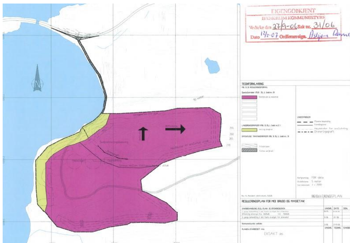
Figur 4. Utsnitt fra reguleringsplankart for Moi brudd og massetak. Store deler av arealet er regulert til steinbrudd og massetak (lilla farge), deler til jord og skogbruk (gulgrønn farge), og vei er regulert til felles avkjørsel (grått med skravur). Kilde: Bjerkreim kommunes planregister.
