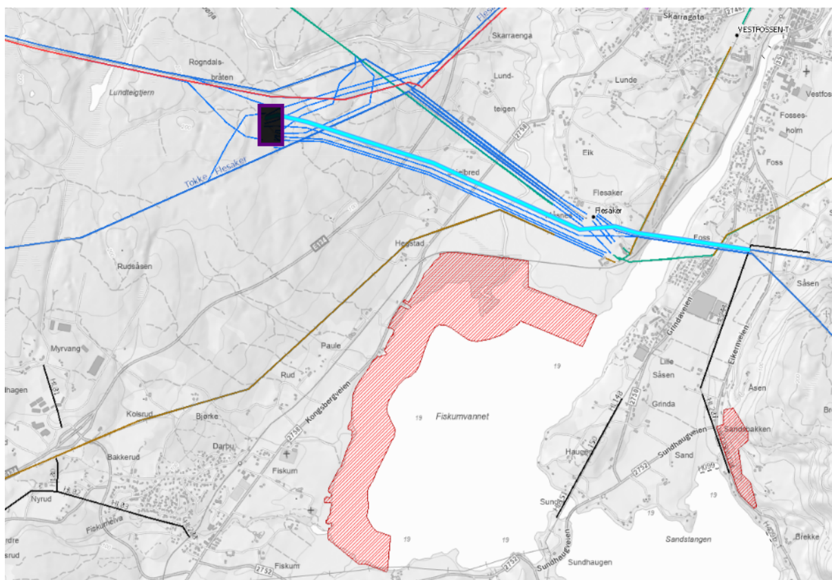
Figur 1 Eiker transformatorstasjon vist med svart firkant, 420 og 132 kV ledninger vist med blå streker, hvor de nye er lengst sør, og Fiskumvannet naturreservat med rødt skravert felt. Kilde: NVE Atlas.
