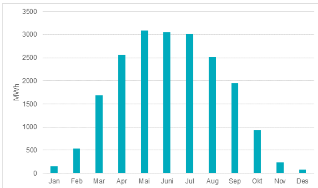
Figur 3-5: Estimert månedlig energiproduksjon
