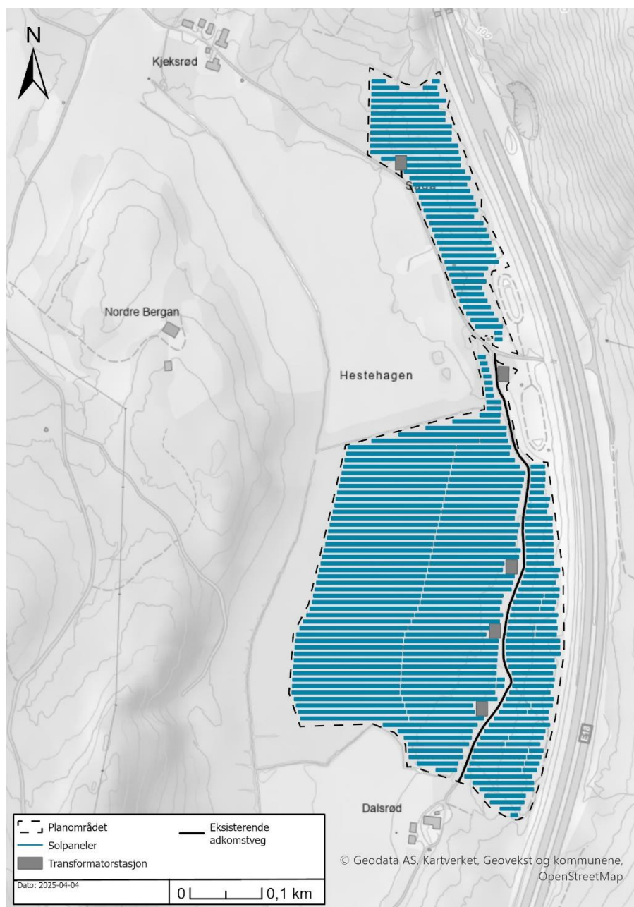
Figur 3-4: Foreløpig layout av Hestehagen solkraftverk.
