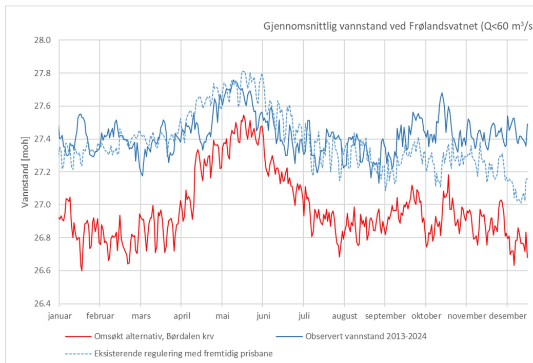
Figur 5-43 Gjennomsnittlig vannstand i Frølandsvatnet (ved vannføringer under 60 m 3 /s)
