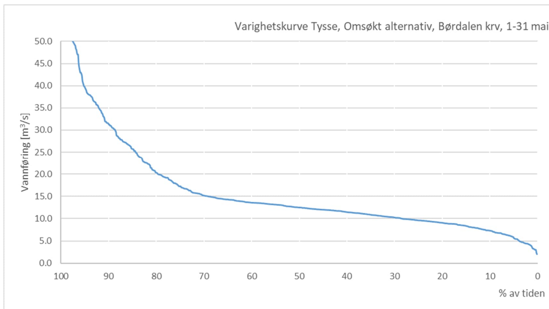
Figur 8-14 Varighetskurve etter omsøkt kraftverk
