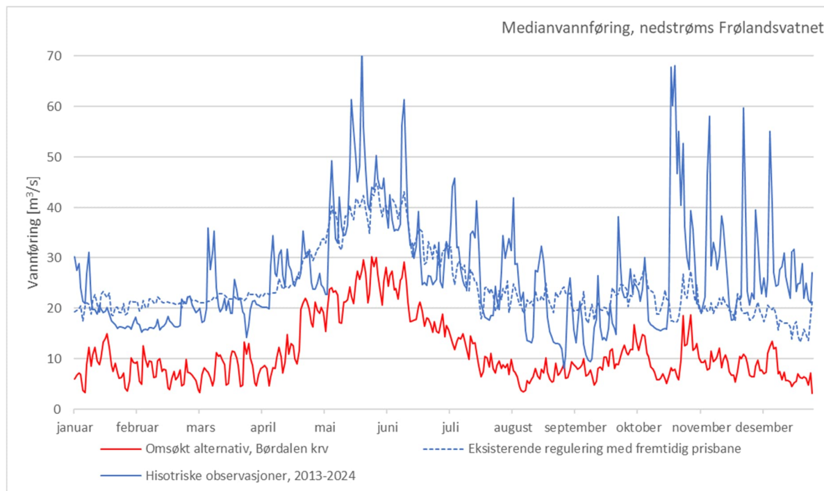
Figur 5-47 Observert medianvannføring for perioden 2013-2024 vist sammen med medianvannføring for eksisterende regulering gitt fremtidig prisbane og omsøkt alternativ (1988-2015).
