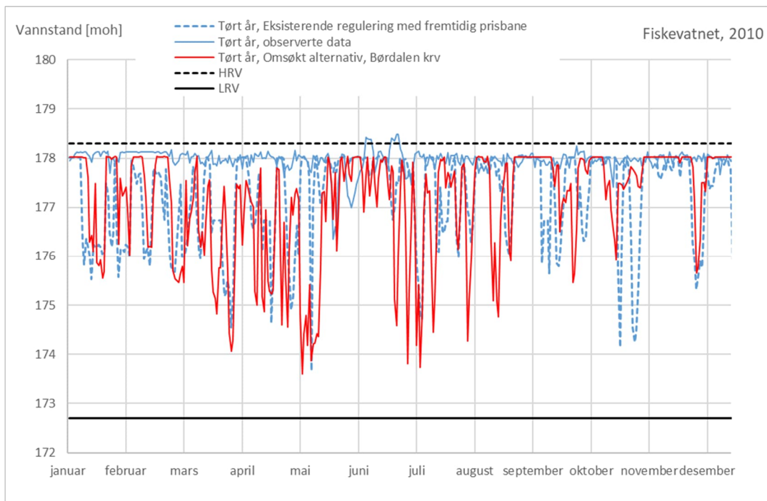
Figur 5-23 Vannstandsvariasjon i et tørt år ved eksisterende regulering og ved omsøkt alternativ (2010)
