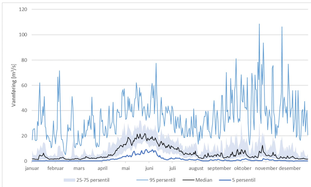
Figur 5-41 Persentilkurver ved innløp Frølandsvatnet for tilsig fra Frølandselva
