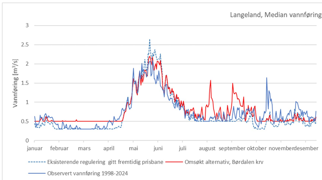
Figur 5-32 Medianvannføring før og etter omsøkt alternativ
