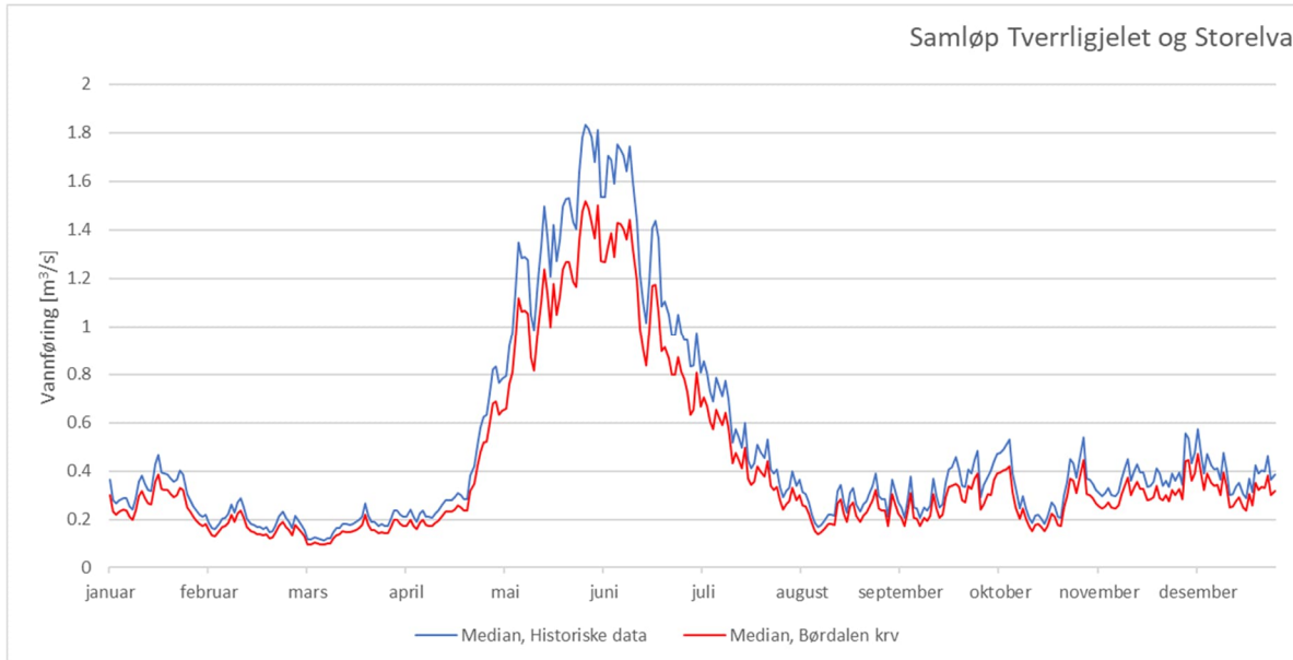
Figur 5-12 Medianvannføring før og etter overføring av felt til bekkeinntak, omsøkt alternativ Børdalen kraftverk
