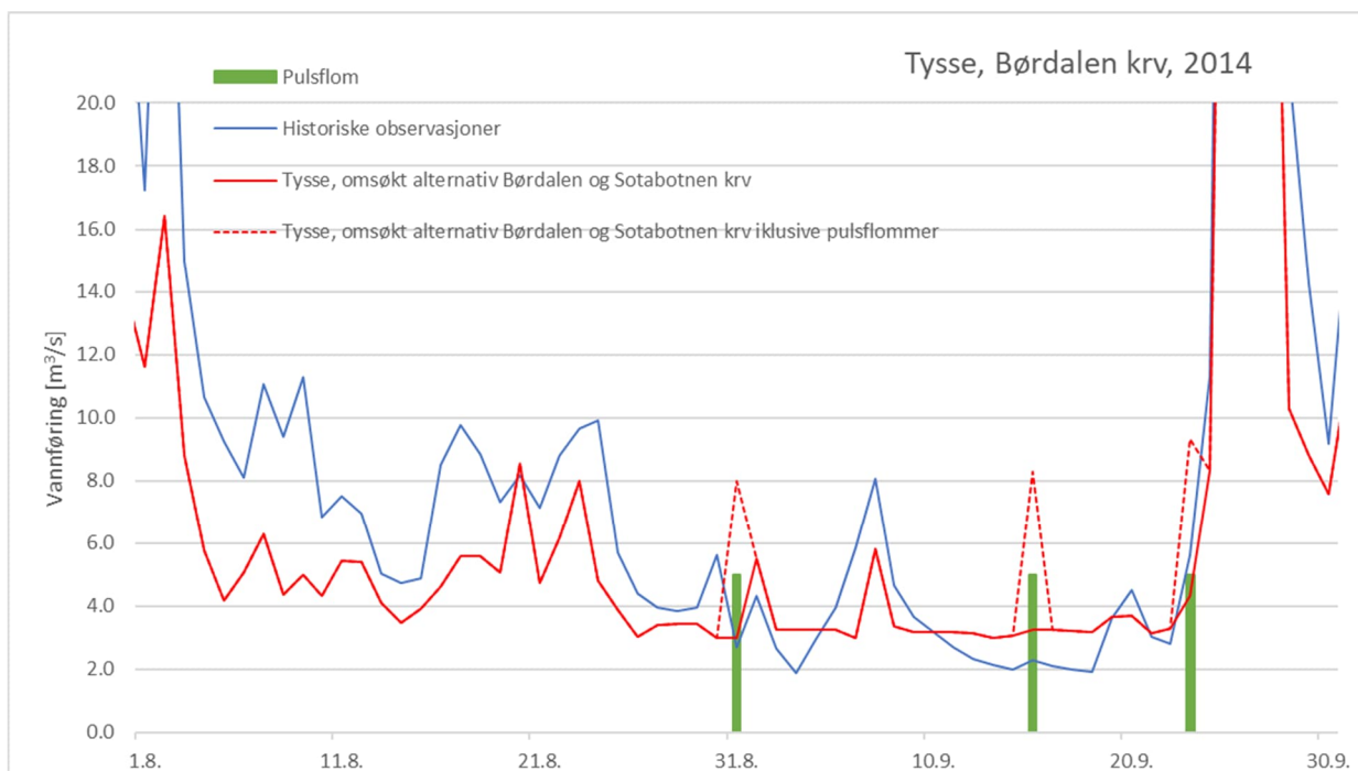
Figur 5-60 Pulsflommer ved Tysse, omsøkt alternativ Børdalen kraftverk, 2014, august og september
