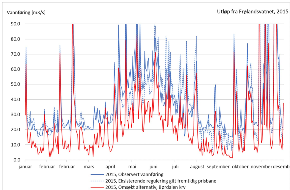
Figur 5-50 Observert vannføring, vannføring ved eksisterende regulering gitt fremtidig prisbane og ved omsøkt alternativ for 2015
