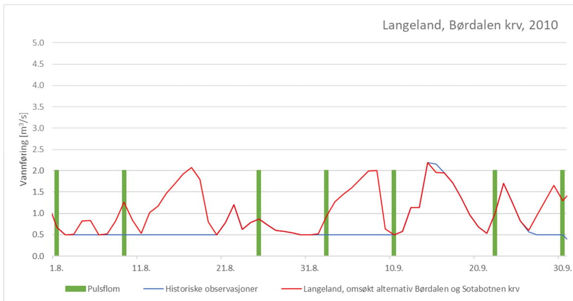
Figur 5-38 Pulsflommer (august og september) ved Langeland for 2010, omsøkt alternativ Børdalen kraftverk
