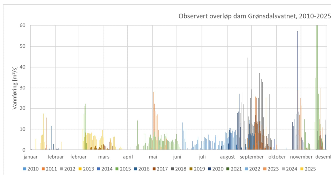
Figur 5-18 Historiske overløpsepisoder, dam Grønsdalsvatn
