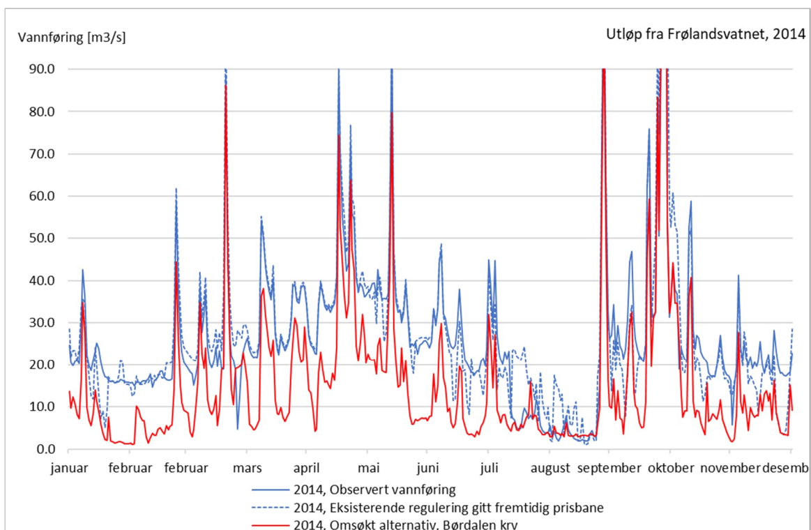
Figur 5-49 Observert vannføring, vannføring ved eksisterende regulering gitt fremtidig prisbane og ved omsøkt alternativ for 2014
