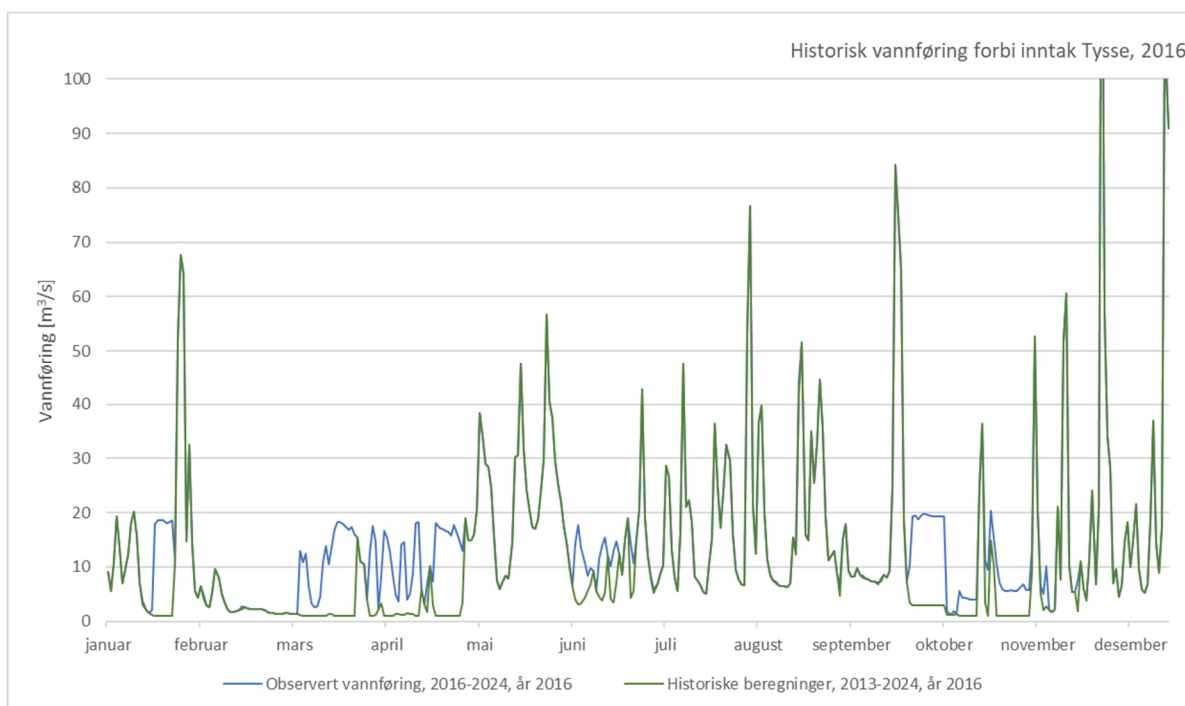
Figur 5-51 Vannføring forbi Tysse kraftverk, observert vannføring og beregnet historisk vannføring for 2016
