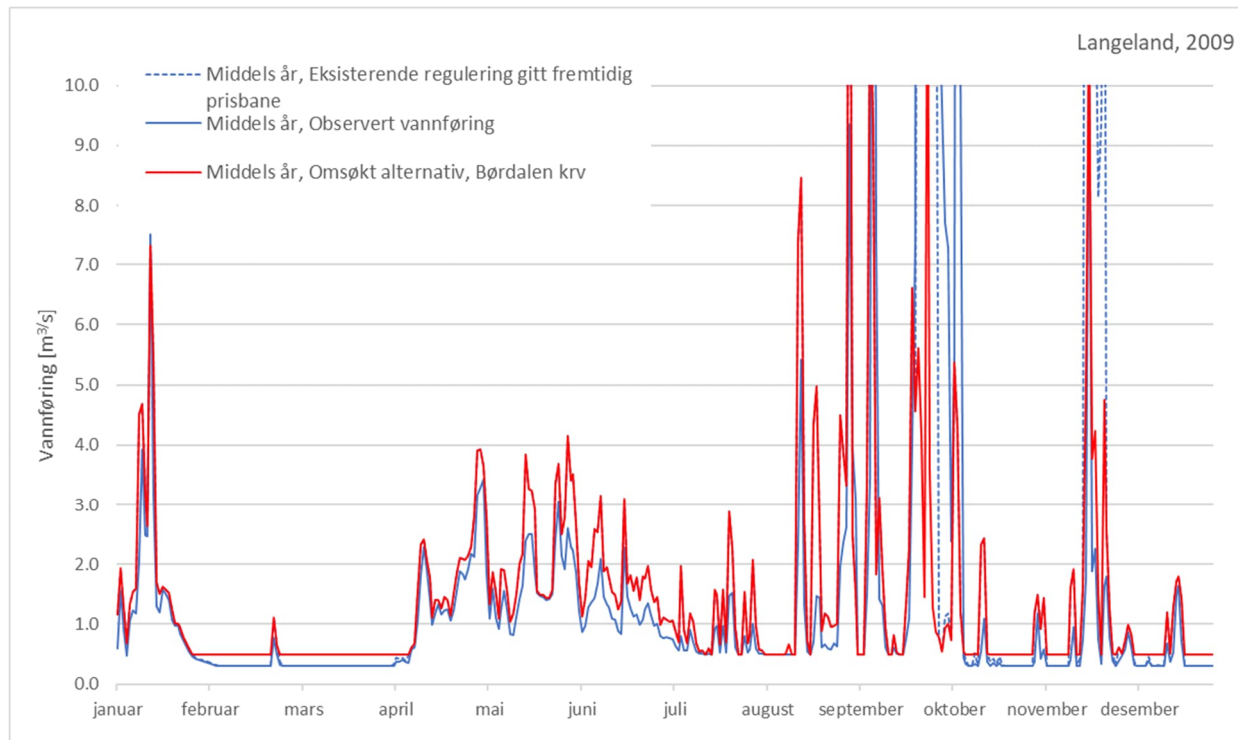
Figur 5-34 Vannføring ved Langeland, middels år (2009), eksisterende regulering gitt fremtidig prisbane, observert vannføring og omsøkt alternativ
