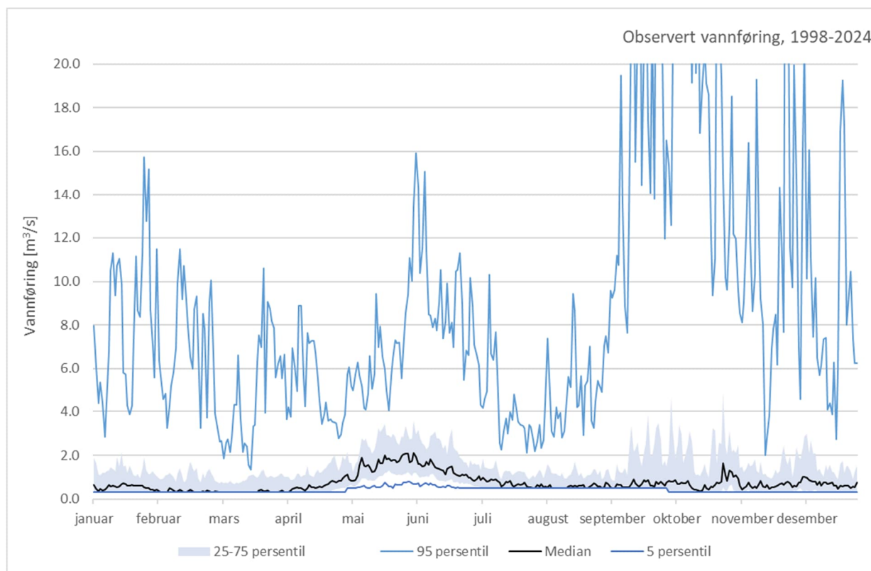
Figur 5-31 Persentilcurver for observert serie ved Langeland, 1998-2024
