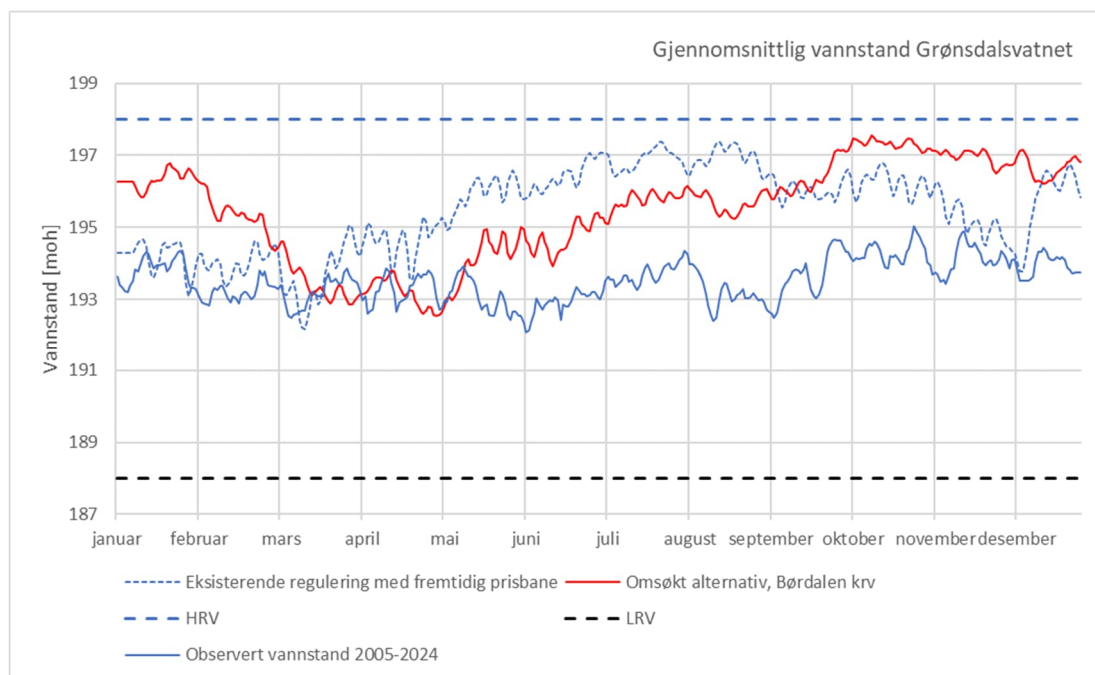
Figur 5-17 Gjennomsnittlig vannstand i Grønsdalsvatnet, observert vannstand, vannstand ved omsøkt alternativ og ved eksisterende regulering gitt fremtidig prisbane
