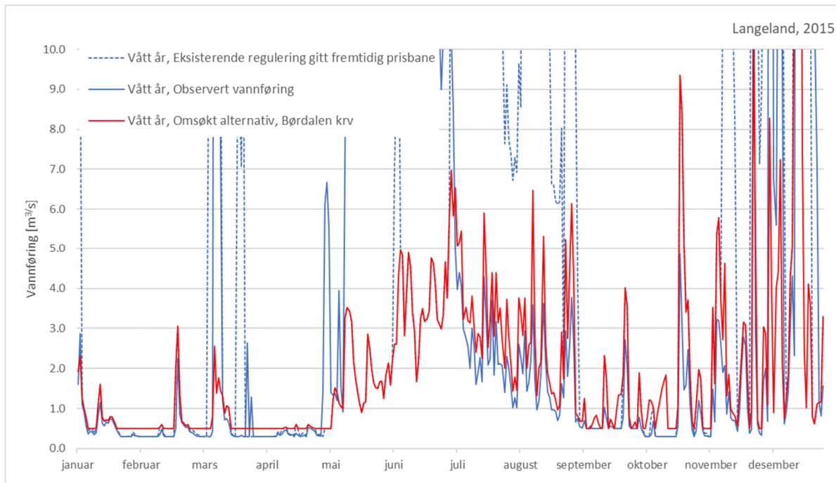
Figur 5-36 Vannføring ved Langeland, vått år (2015), eksisterende regulering gitt fremtidig prisbane, observert vannføring og omsøkt alternativ
