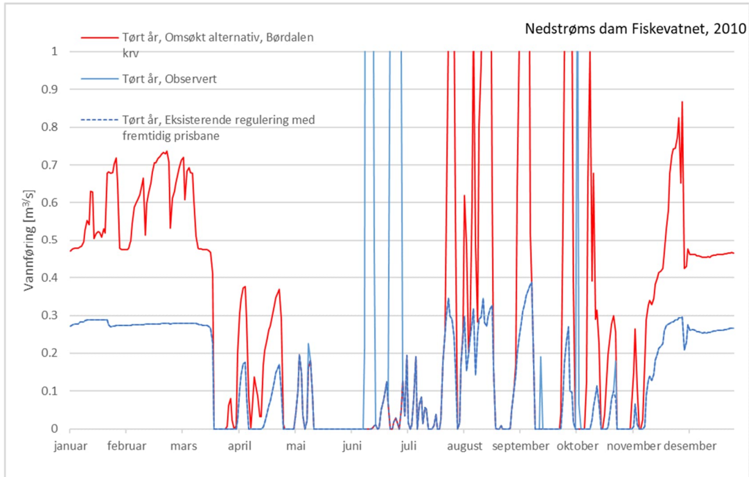
Figur 5-28 Vannføring nedstrøms Fiskevatnet, tørt år. (2010)
