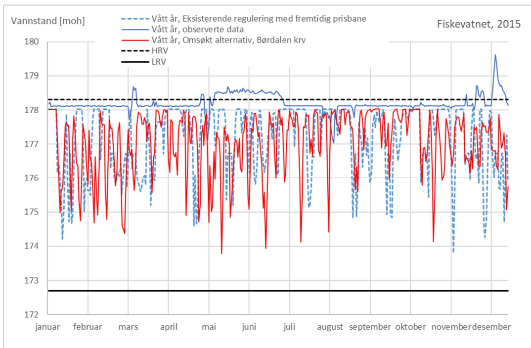
Figur 5-24 Vannstandsvariasjon i et vått år ved eksisterende regulering og ved omsøkt alternativ (2015)
