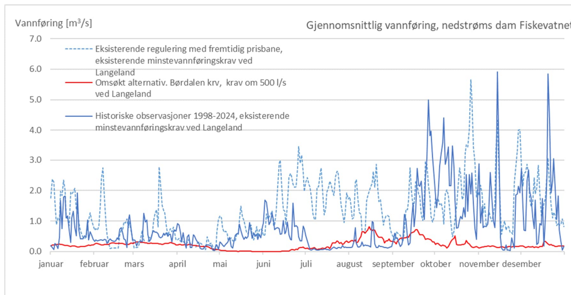
Figur 5-25 Gjennomsnittlig vannføring nedstrøms dam Fiskevatnet
