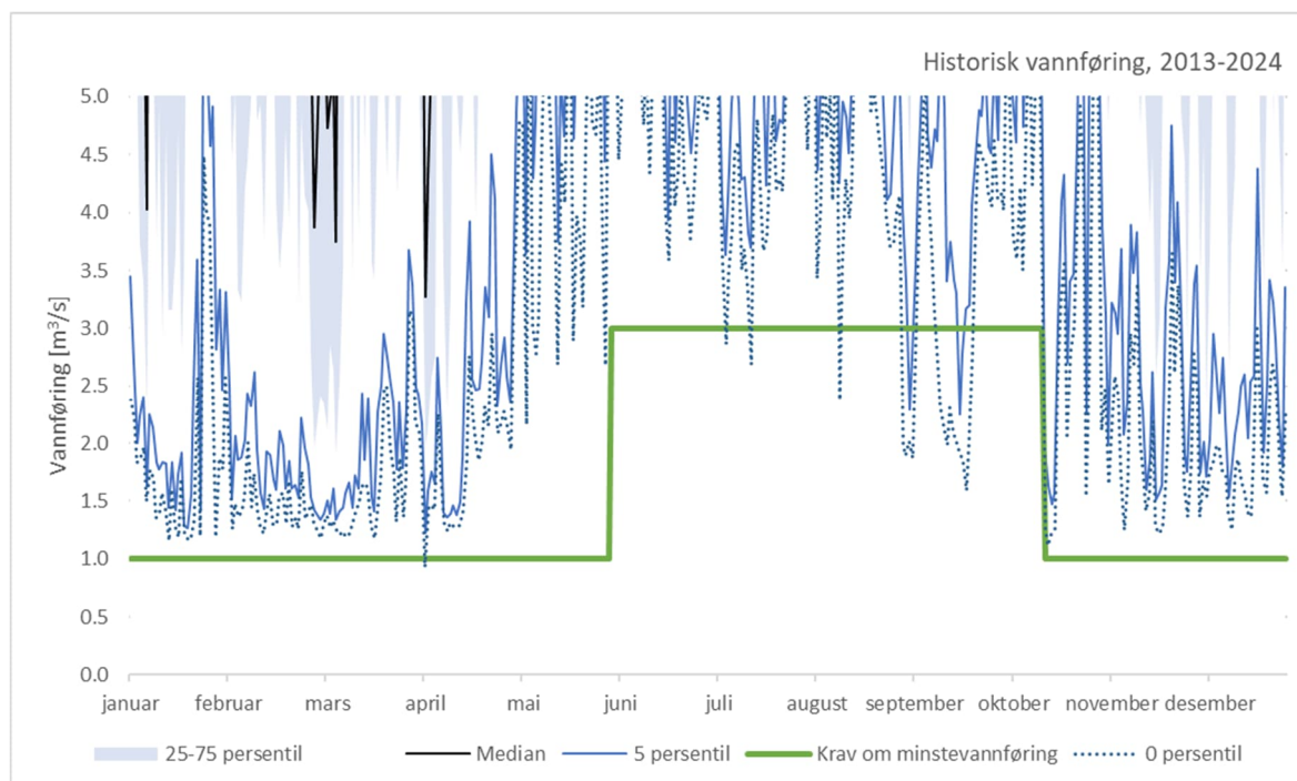
Figur 5-52 Persentilkurver for historisk vannføring forbi inntak Tysse med fokus på minstevannføringskrav og episoder med lav vannføring. NB kraftverket står ved lavere vannføring enn minstevannføringskravet gitt gjeldende vilkår.
