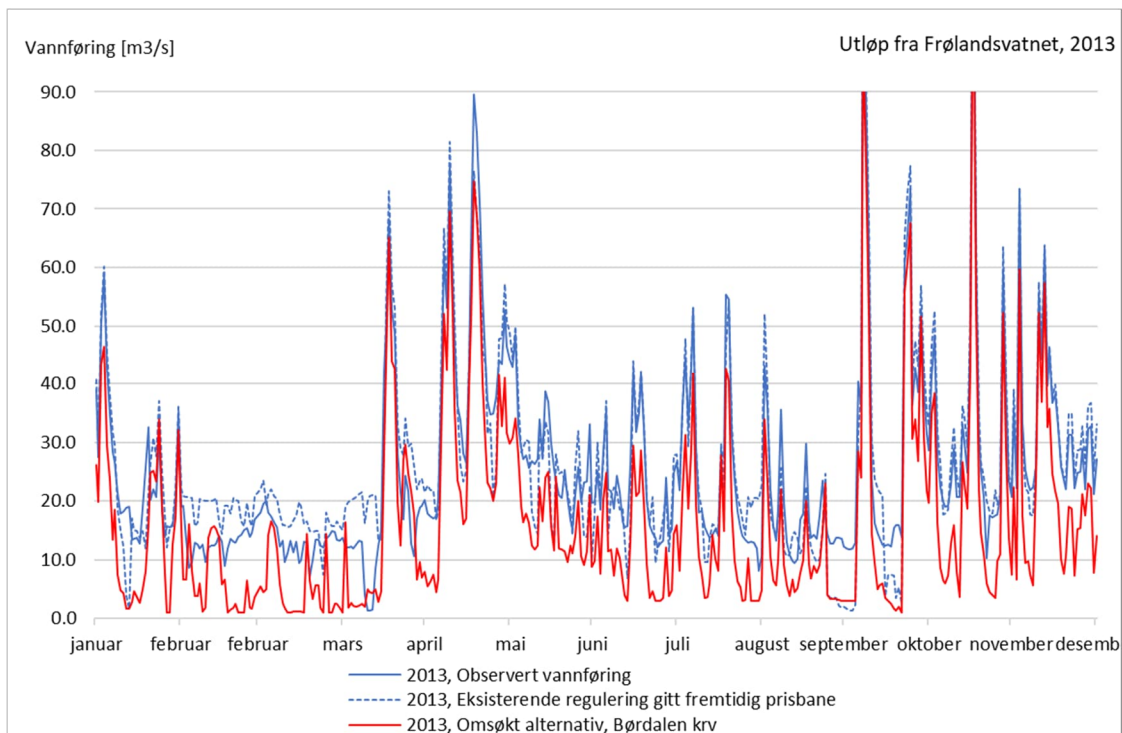
Figur 5-48 Observert vannføring, vannføring ved eksisterende regulering gitt fremtidig prisbane og ved omsøkt alternativ for 2013.
