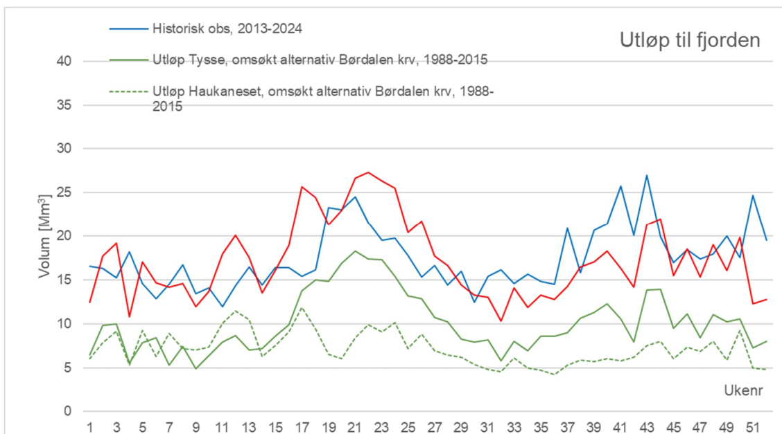
Figur 5-62 Utløp til fjorden, Gjennomsnittlig volum vann pr uke, rød kurve viser eksisterende kraftverk med framtidige priser.
