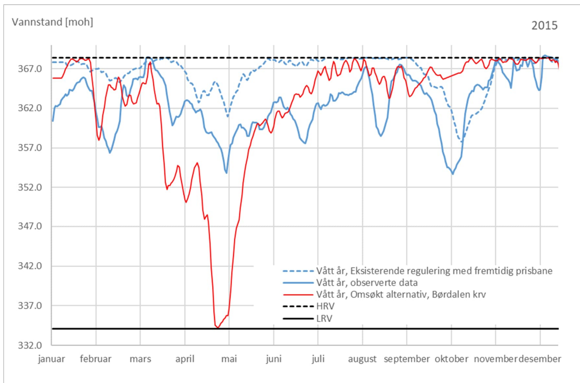
Figur 5-7 Vannstandsvariasjon i Kvitingvatnet i et typisk vått år (2015)
