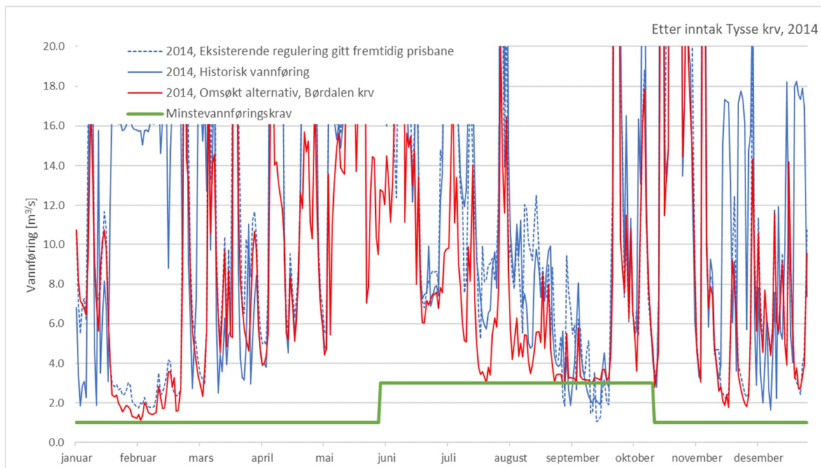
Figur 5-57 Vannføring 2014 for omsøkt alternativ, eksisterende regulering gitt fremtidig prisbane og historisk vannføring, detaljer
