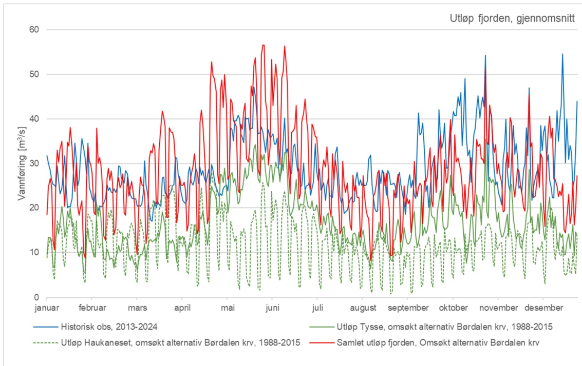
Figur 5-61 Gjennomsnittlig utløp til fjorden ved omsøkt alternativ Børdalen krv (1988-2015) sammen med historisk utløp (2013-2024)
