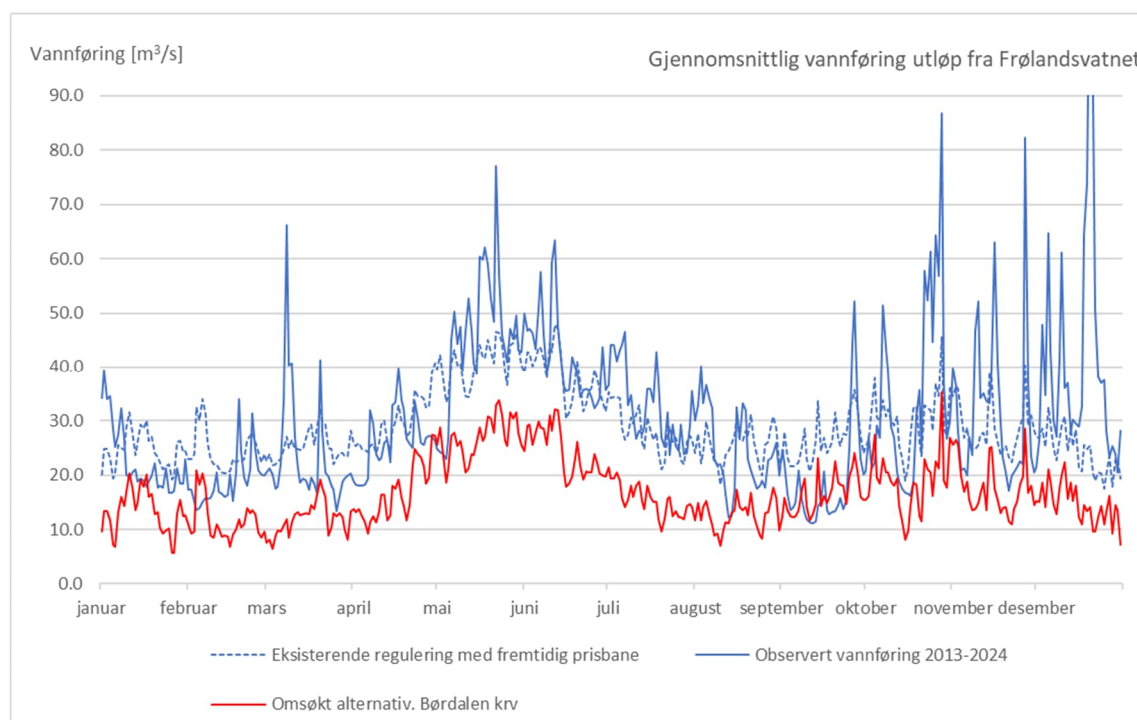
Figur 5-46 Observert gjennomsnittlig vannføring for perioden 2013-2024 vist sammen med gjennomsnittlig vannføring for eksisterende regulering gitt fremtidig prisbane og omsøkt alternativ (1988-2015)
