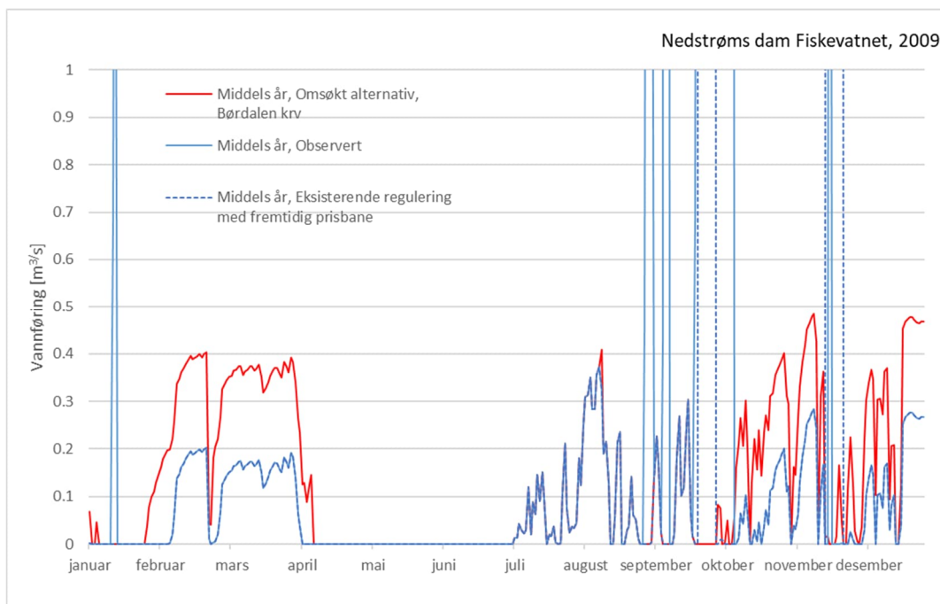
Figur 5-27 Vannføring nedstrøms Fiskevatnet, middels år (2009).
