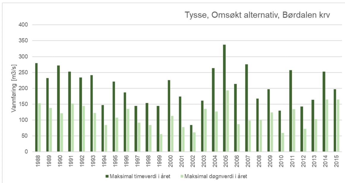
Figur 9-9 Maksimal døgnvannføring og timesvannføring pr år, Børdalen krv
