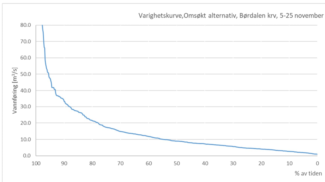
Figur 7-10 Varighetskurve for Frølandsvatnet etter omsøkt alternativ
