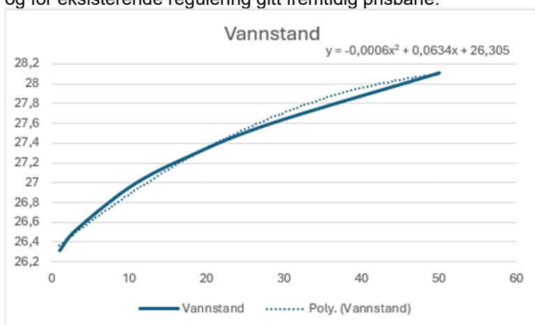
Figur 5-42 Vannføringskurve Frølandsvatnet (kilde LFI, 2025)
