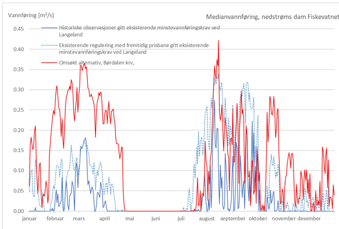
Figur 5-26 Medianvannføring nedstrøms dam Fiskevatnet
