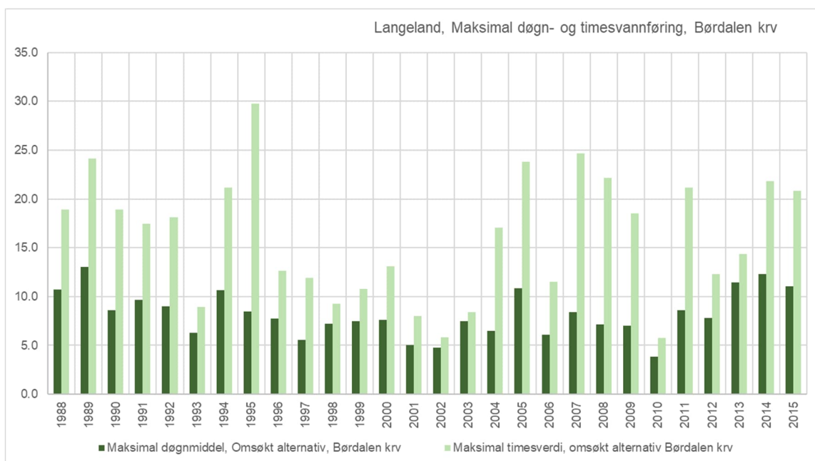
Figur 9-3 Flomvannføring Langeland etter omsøkt alternativ, Børdalen krv
