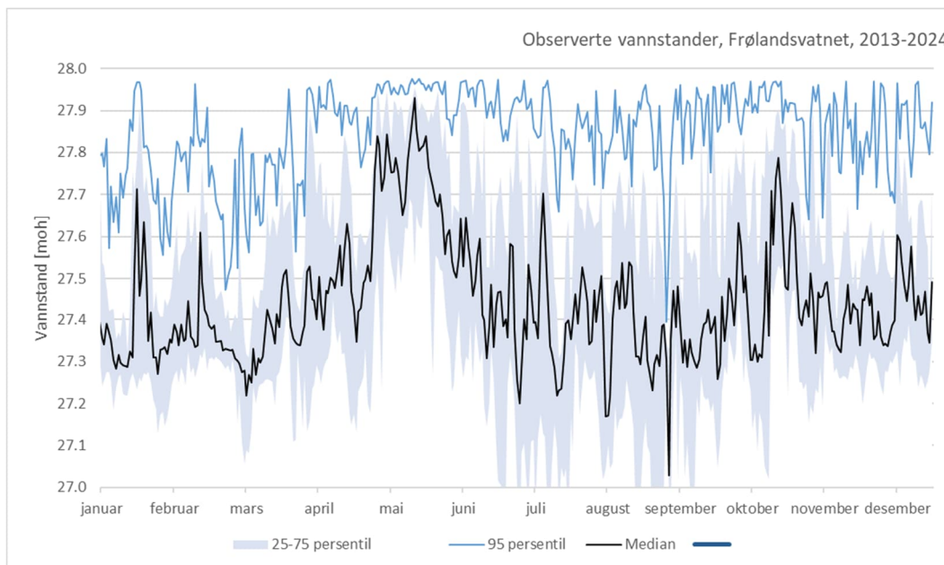
Figur 5-44 Persentilkurver for observert vannstand i Frølandsvatnet for perioden 2013-2024
