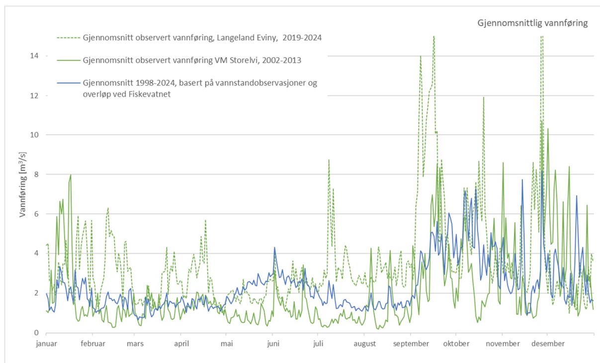
Figur 5-30 Gjennomsnittlig vannføring for årene 1998-2024 ved Langeland (Storelvi)
