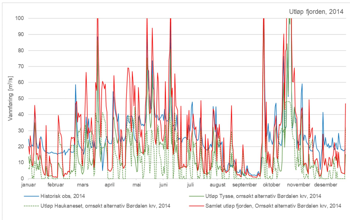
Figur 5-65 Vannføring til fjorden, døgngjennomsnitt, 2014.
