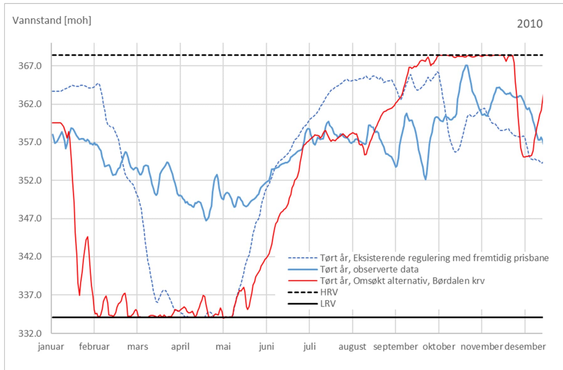
Figur 5-6 Vannstandsvariasjon i Kvitingvatnet i et typisk tørt år (2010)
