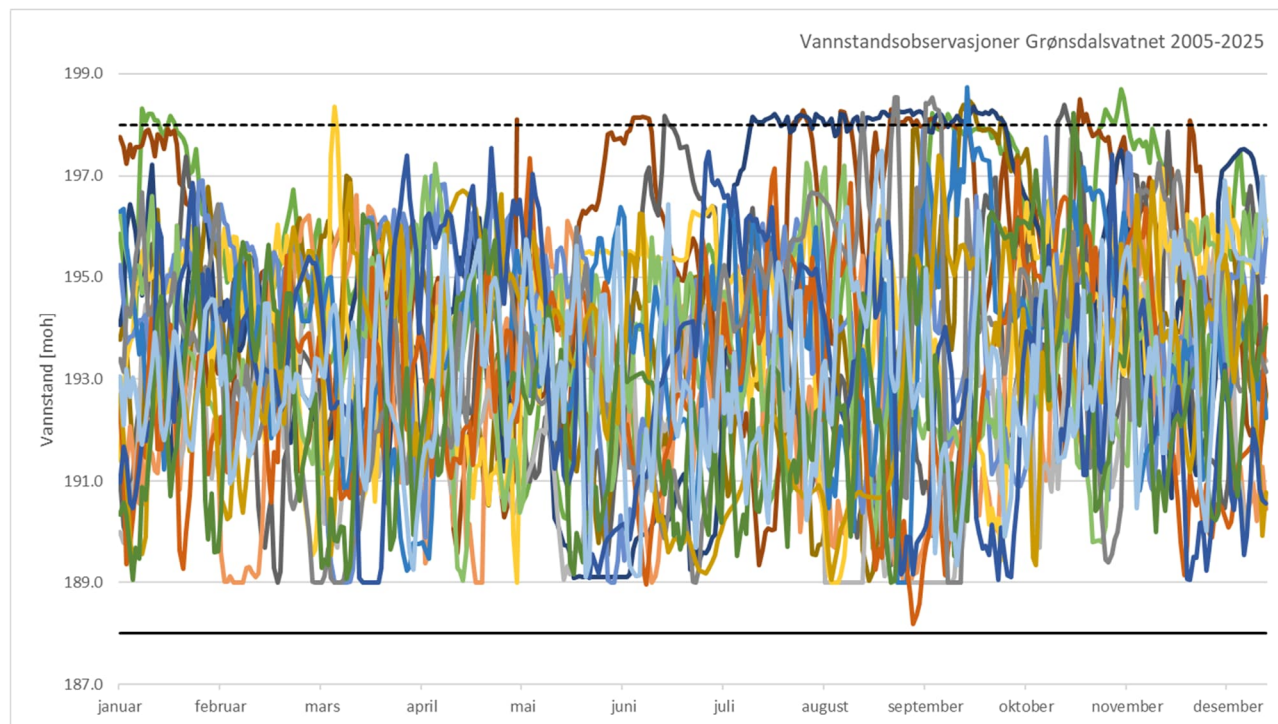
Figur 5-16 Observerte vannstander i Grønsdalsvatnet mellom 2005-2024
