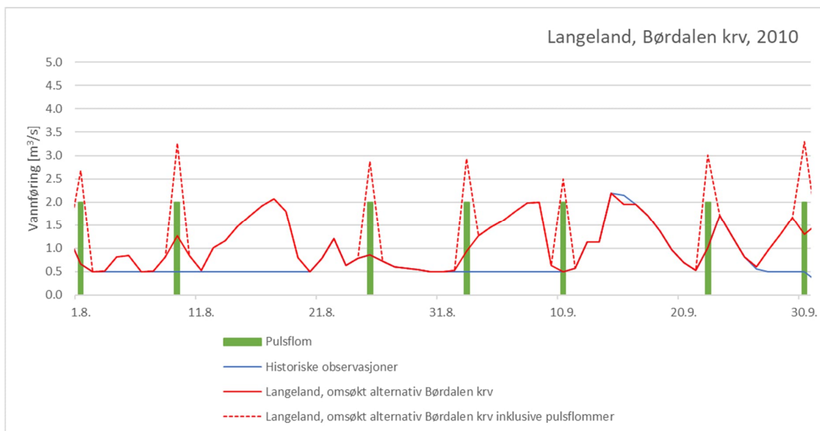
Figur 5-39 Pulsflommer (august og september) ved Langeland for 2010, omsøkt alternativ Børdalen kraftverk
