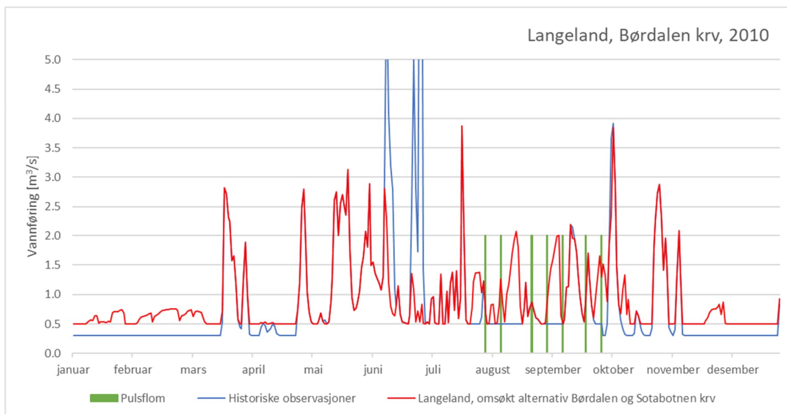
Figur 5-37 Pulsflommer ved Langeland for 2010, omsøkt alternativ Børdalen kraftverk.
