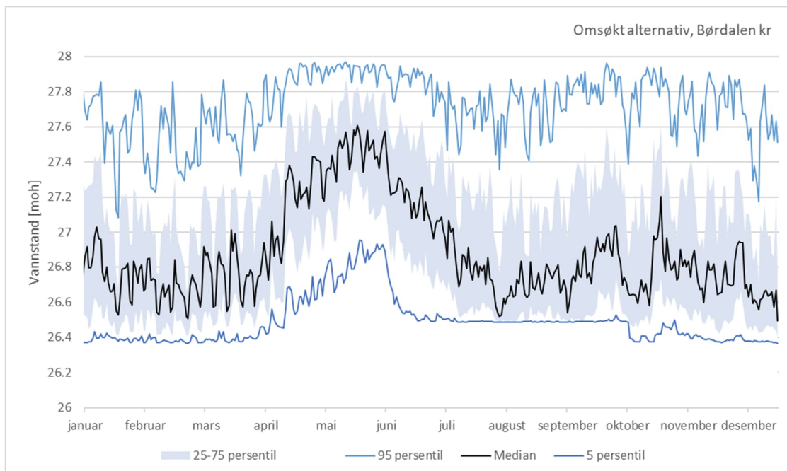
Figur 5-45 Persentilkurver for vannstand i Frølandsvatnet for omsøkt alternativ
