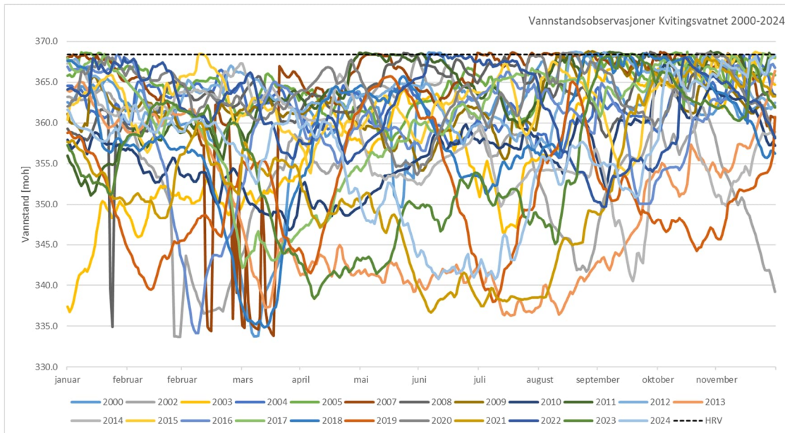
Figur 5-1 Observert magasin vannstand for årene 2000-2024 i Kvittingsvatnet, med unntak av 2001 og 2006,
