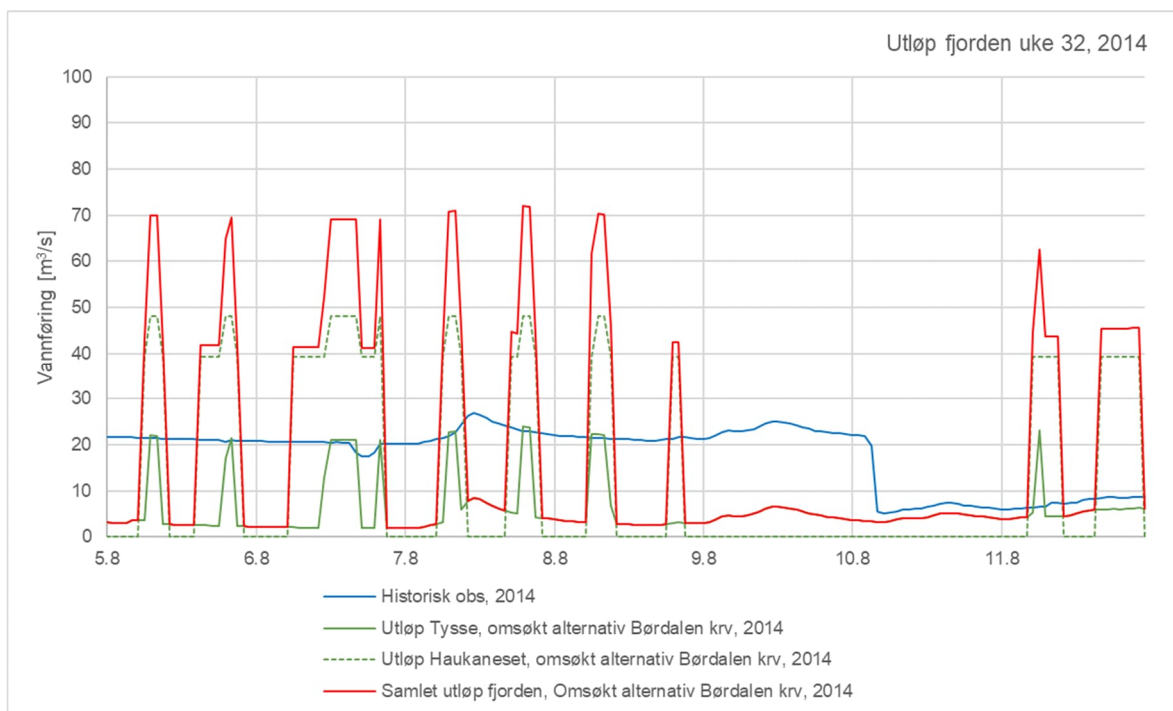
Figur 5-64 Vannføring til fjorden, uke i oktober, 2014
