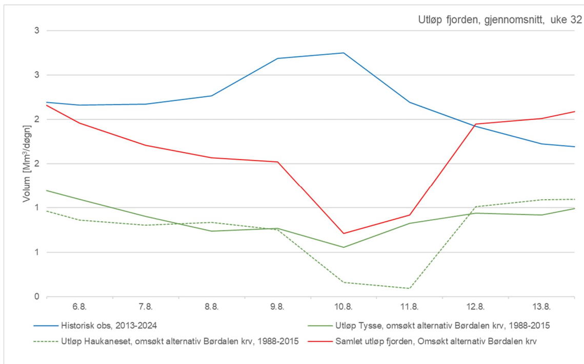
Figur 5-63 Gjennomsnittlig tilførsel til fjorden i volum/døgn for uke 32
