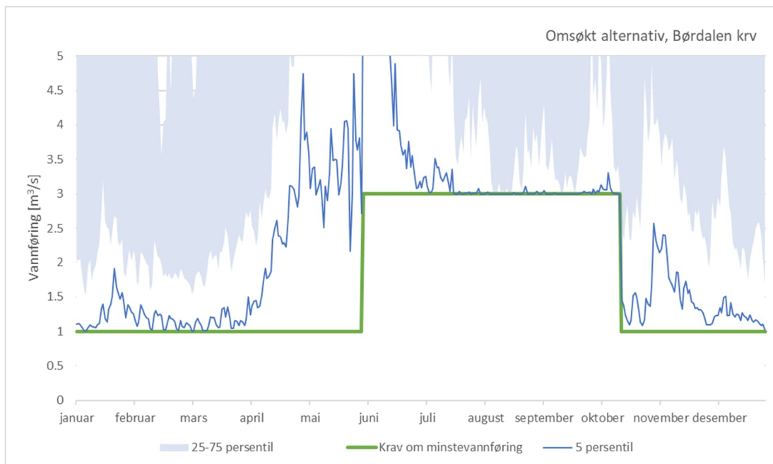
Figur 5-55 Persentilkurver for omsøkt alternativ
