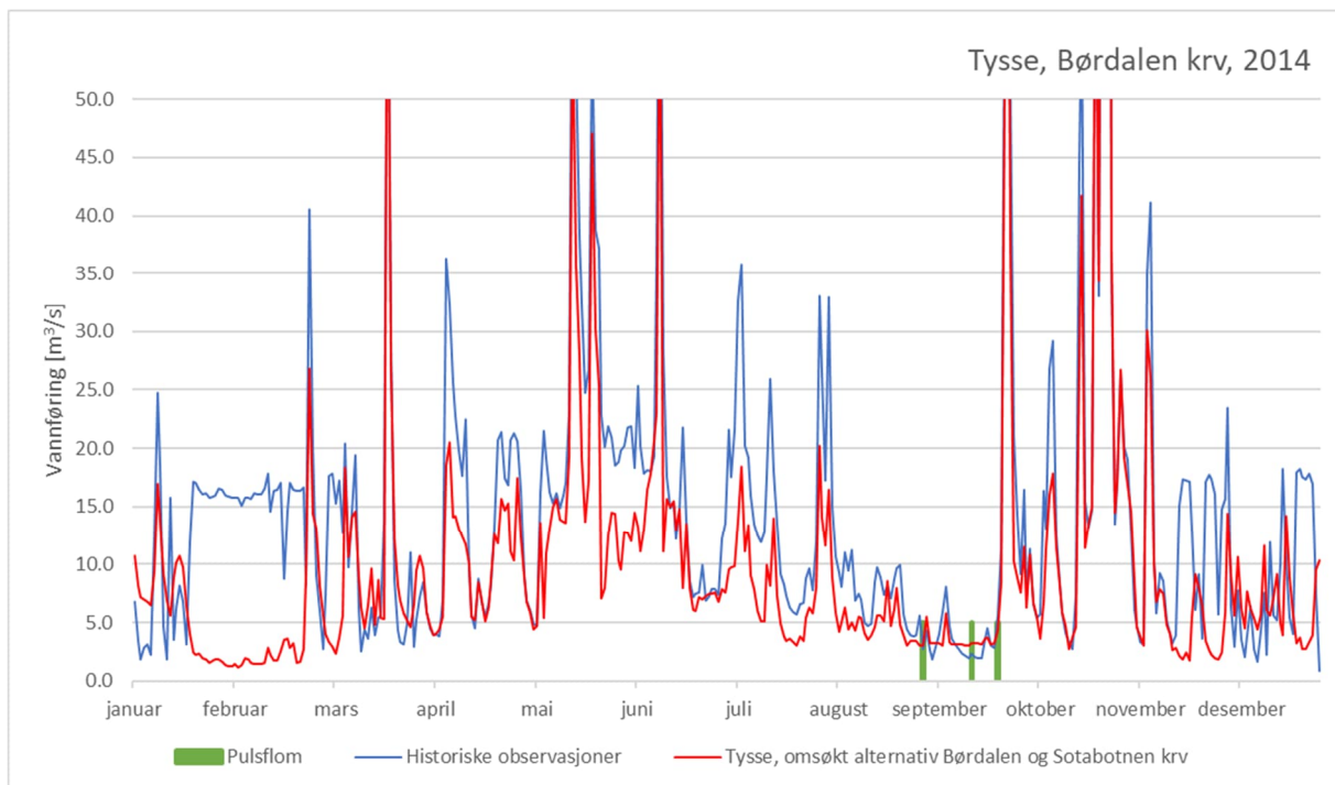
Figur 5-59 Pulsflommer ved Tysse, omsøkt alternativ Børdalen kraftverk, 2014
