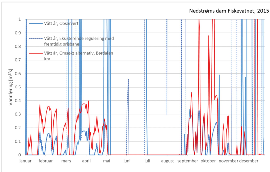
Figur 5-29 Vannføring nedstrøms Fiskevatnet, vått år (2015)
