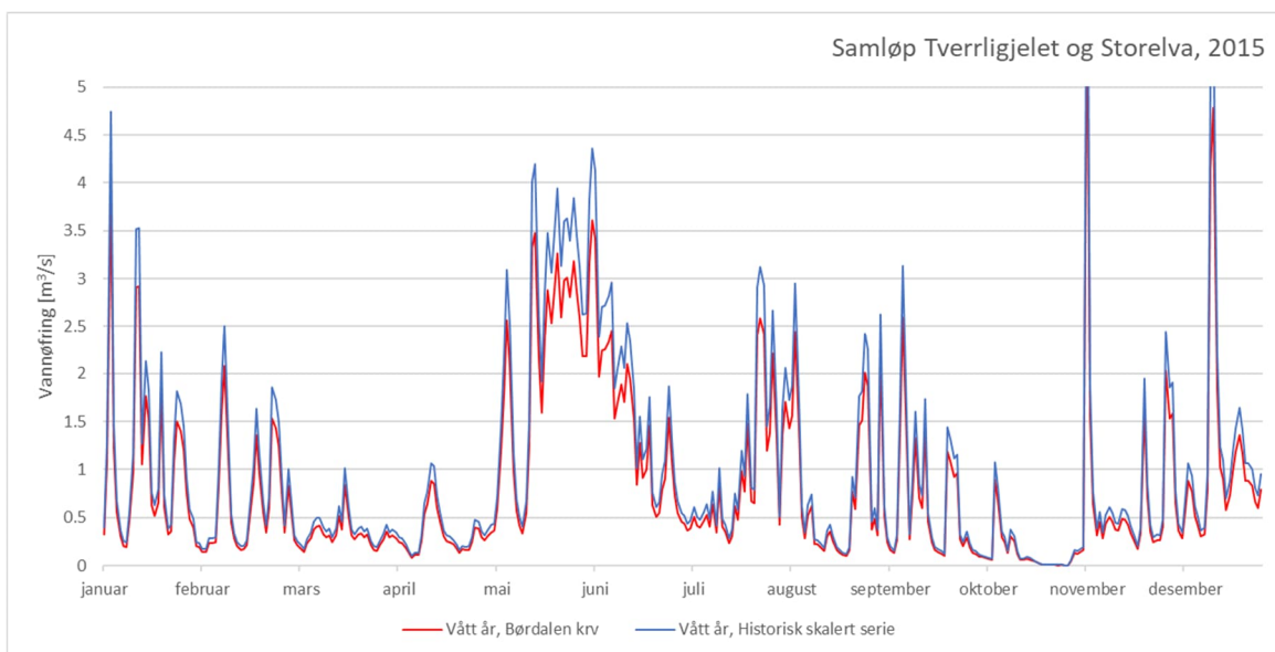
Figur 5-15 Vannføring i et vått år ved samløp Tverrligjelet og Storelva (2015)
