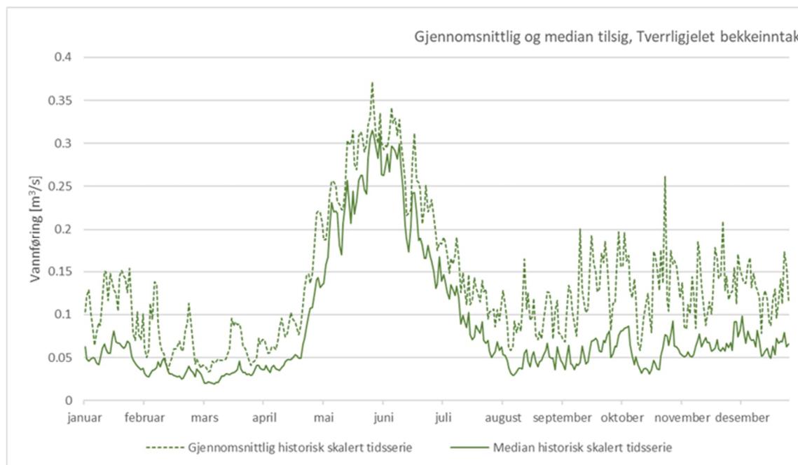
Figur 5-9 Gjennomsnittlig og median vannføring i Tverrligjelet for omsøkt alternativ
