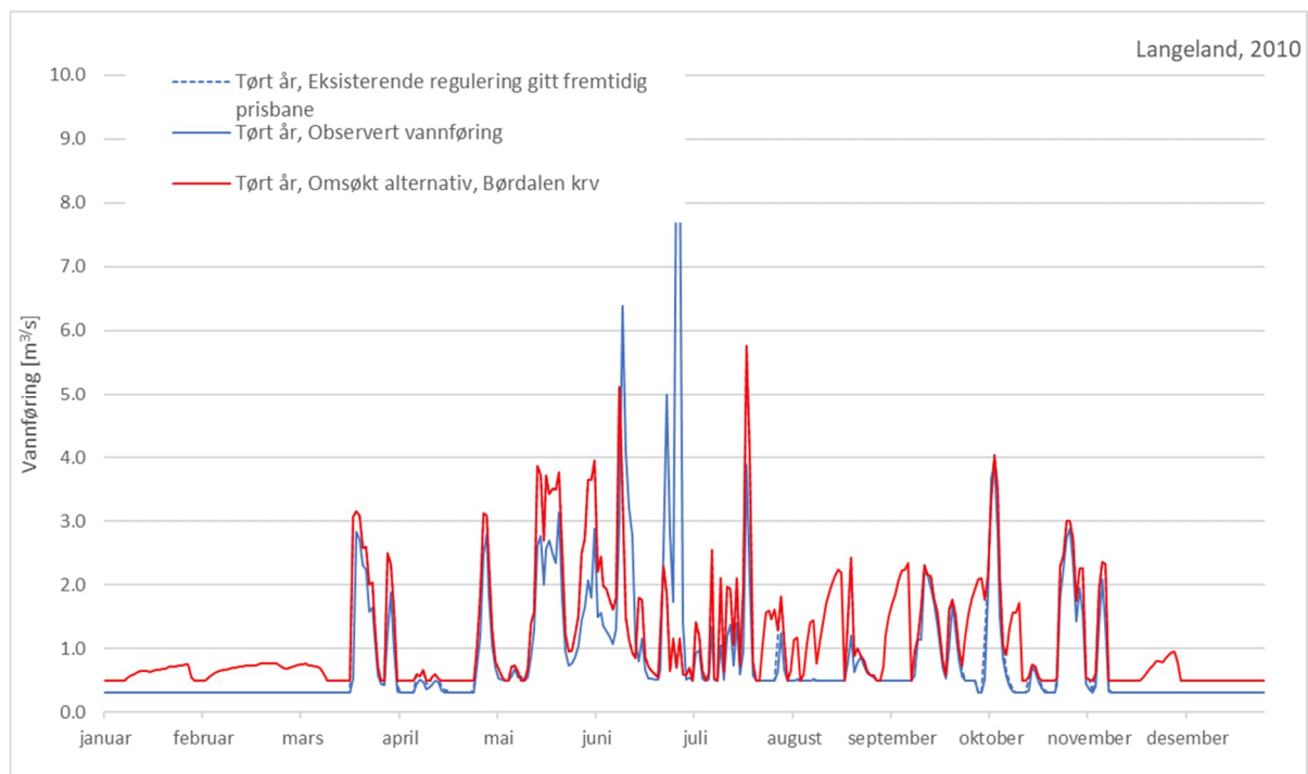
Figur 5-35 Vannføring ved Langeland, tørt år (2010), eksisterende regulering gitt fremtidig prisbane, observert vannføring og omsøkt alternativ
