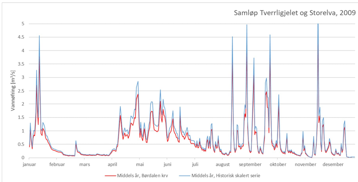
Figur 5-13 Vannføring i et middels år ved samløp Tverrligjelet og Storelva (2009)
