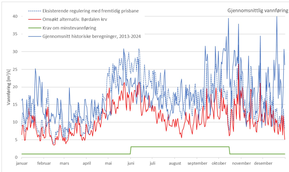
Figur 5-53 Gjennomsnittlig vannføring etter inntak Tyssefossen kraftverk.
