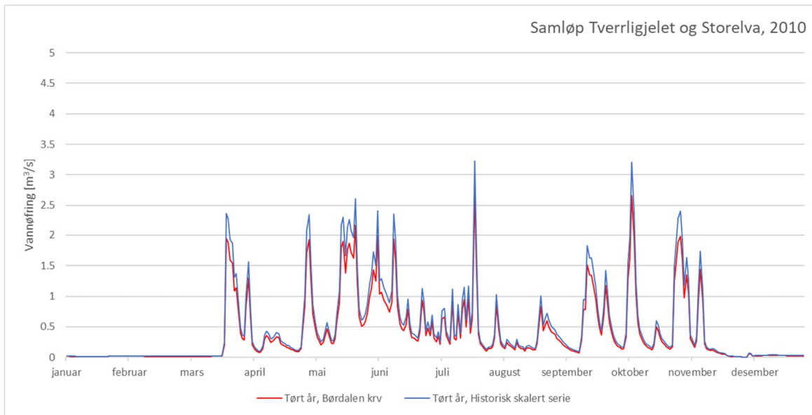
Figur 5-14 Vannføring i et tørt år ved samløp Tverrligjelet og Storelva (2010)
