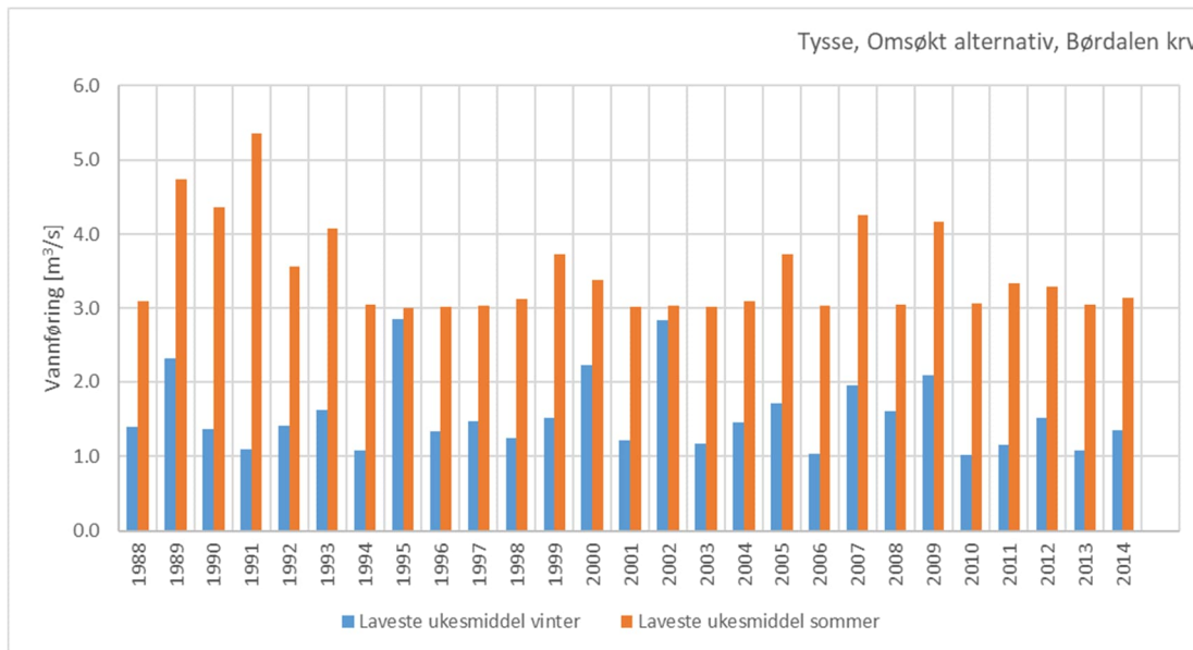
Figur 6-8 Lavvannføring sommer og vinter etter omsøkt alternativ
