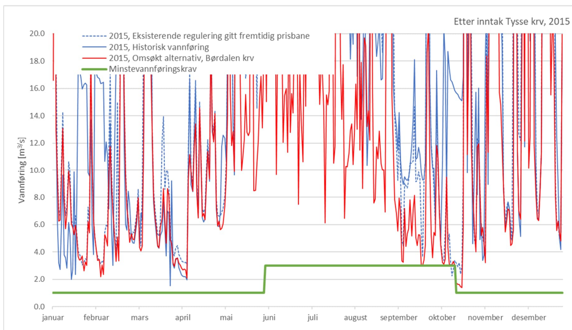
Figur 5-58 Vannføring 2015 for omsøkt alternativ, eksisterende regulering gitt fremtidig prisbane og historisk vannføring, detaljer
