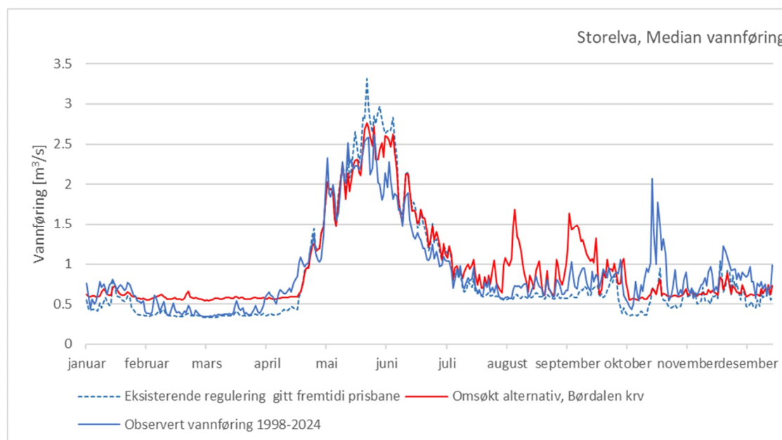
Figur 5-40 Medianvannføring ved utløp av Storelva i Frølandsvatnet, observert vannføring, eksisterende regulering gitt fremtidig prisbane og etter omsøkt alternativ
