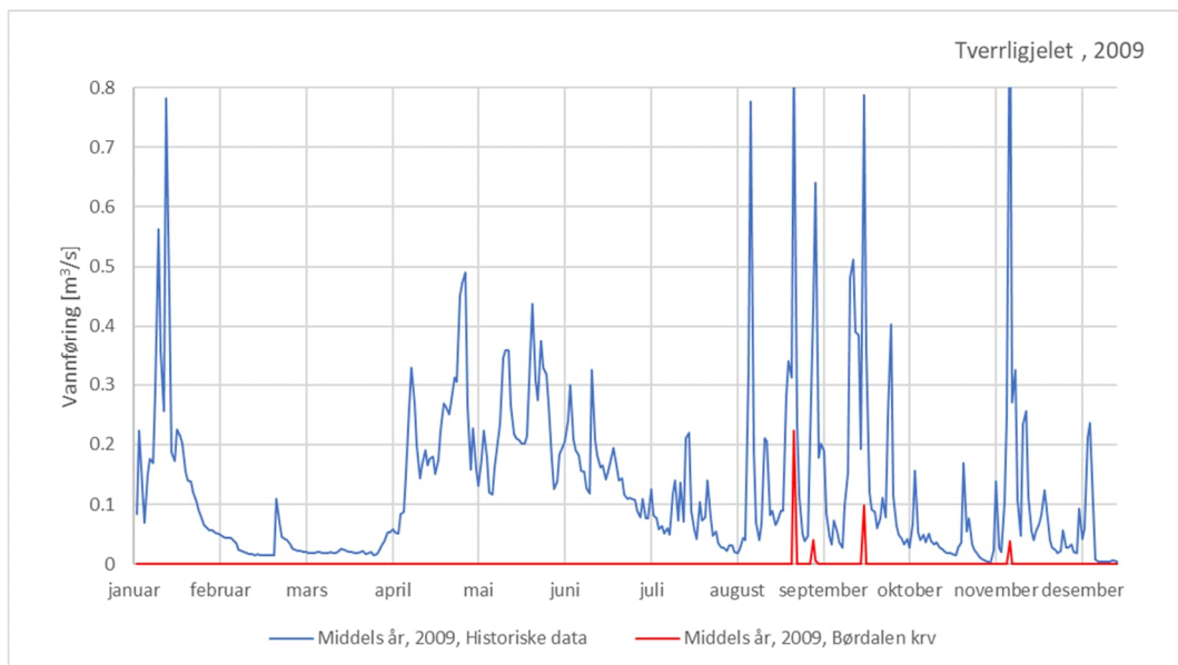
Figur 5-11 Vannføring i et middels år (2009), før og etter omsøkt alternativ med Børdalen krv
