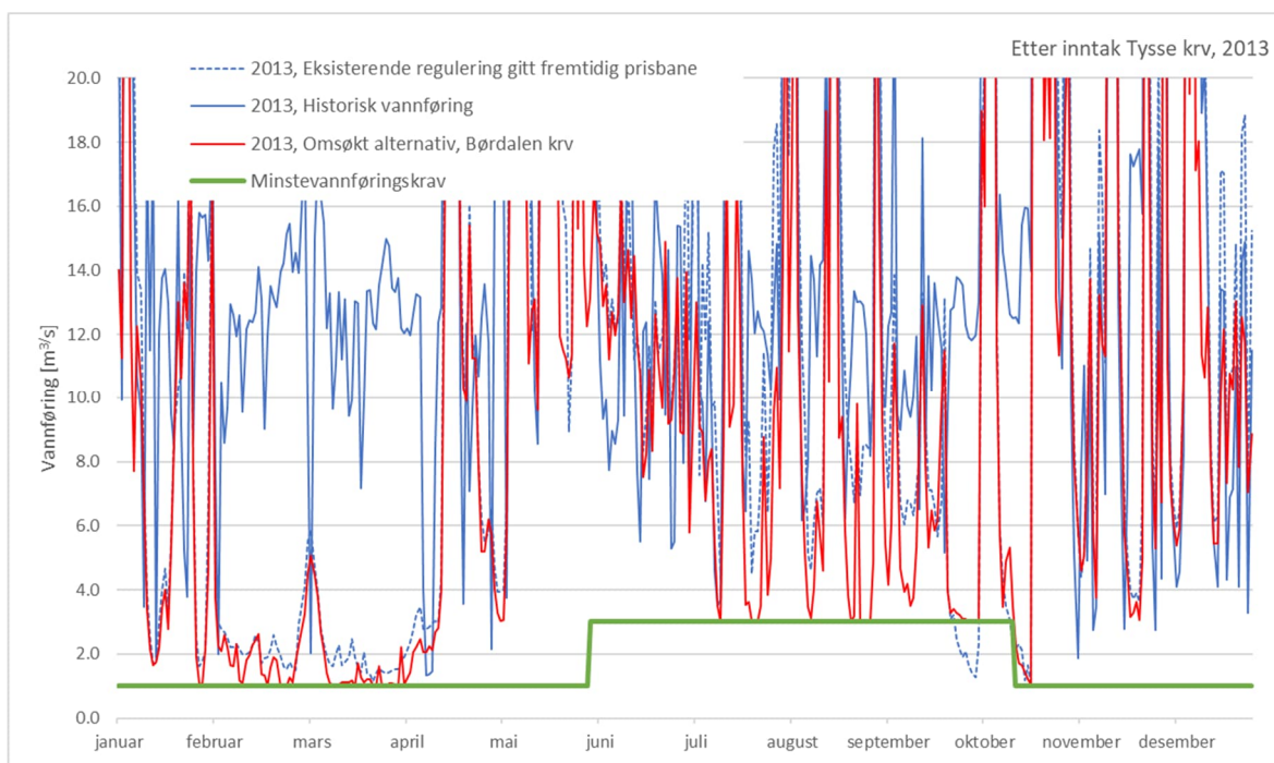
Figur 5-56 Vannføring 2013 for omsøkt alternativ, eksisterende regulering gitt fremtidig prisbane og historisk vannføring
