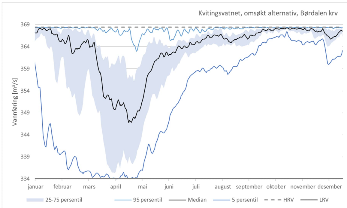
Figur 5-4 Persentilkurver for vannstand i Kvitingvatnet gitt omsøkt alternativ
