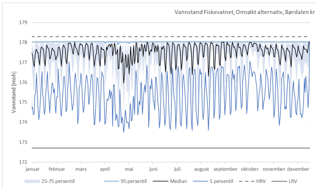
Figur 5-21 Persentilkurver for vannstand i Fiskevatnet ved omsøkt alternativ
