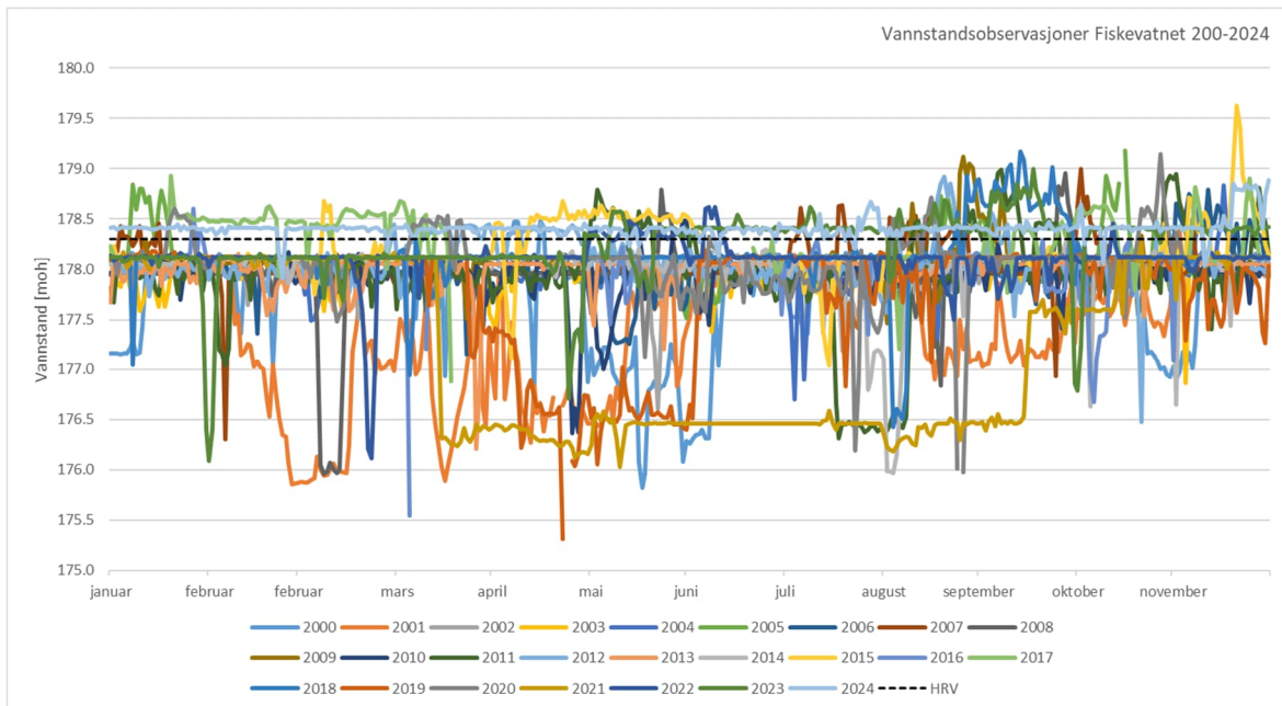
Figur 5-19 Vannstandsobservasjoner i Fiskevatn, 2000-2024
