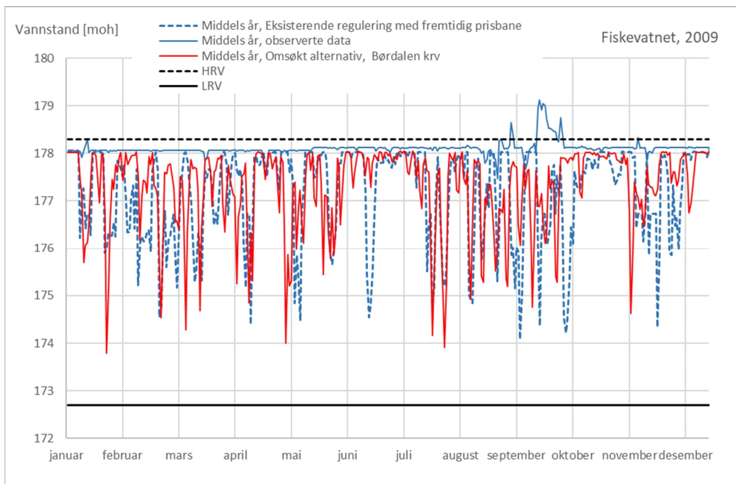
Figur 5-22 Vannstandsvariasjon i et middels år ved eksisterende regulering og ved omsøkt alternativ (2009)
