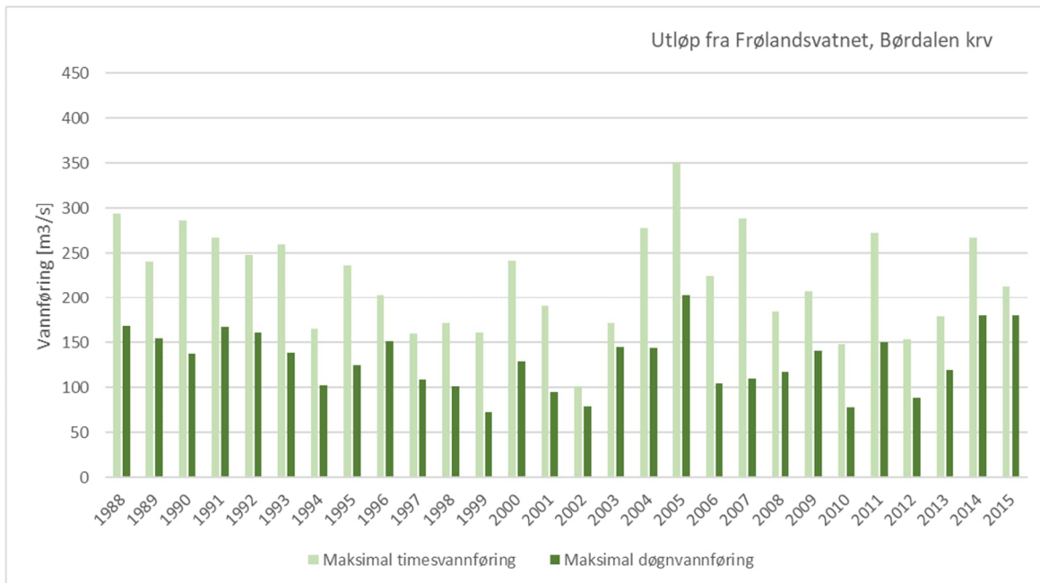
Figur 9-7 Maksimal flomstørrelse pr år etter omsøkt alternativ, Børdalen kr.
