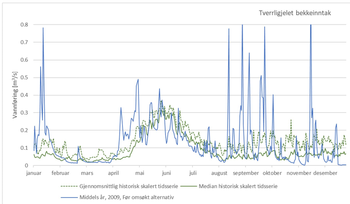
Figur 5-10 Gjennomsnittlig vannføring, medianvannføring og eksempelåret 2009 for Tverrligjelet.
