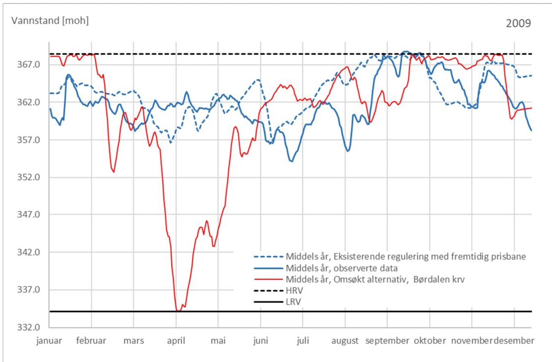
Figur 5-5 Vannstandsvariasjon i et typisk middels år for Kvitingvatnet, 2009
