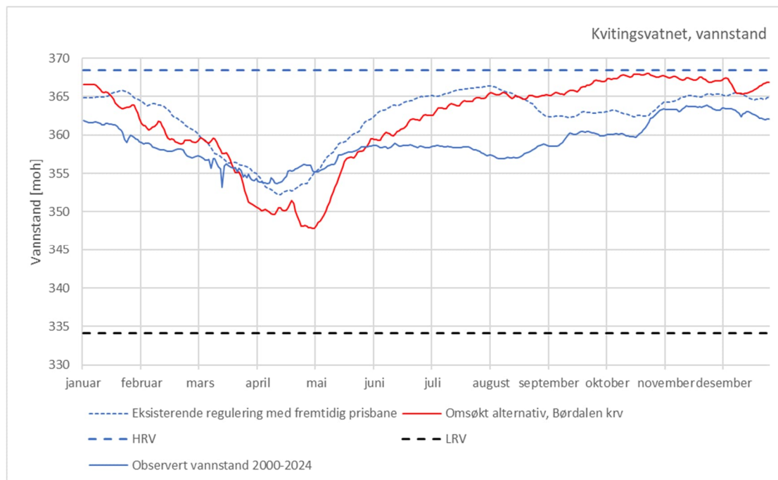
Figur 5-3 Gjennomsnittlig vannstandsvariasjon over året, Kvitingsvatnet
