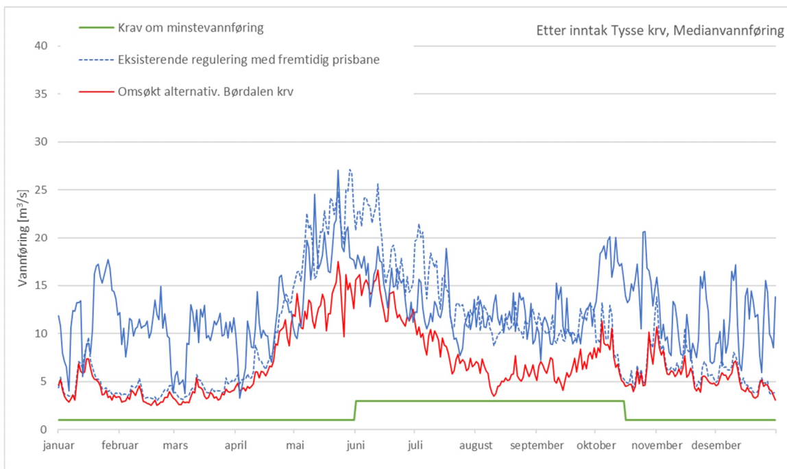
Figur 5-54 Medianvannføring etter inntak Tyssefossen kraftverk.
