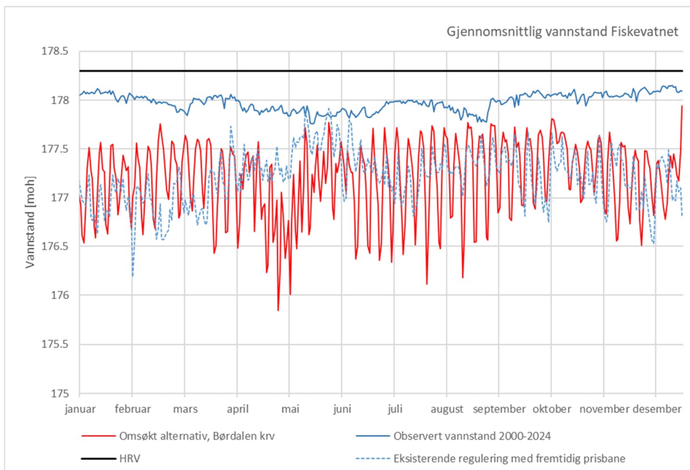
Figur 5-20 Middelvannstand for observert serie, eksisterende regulering med fremtidig prisbane og ved omsøkt alternativ.
