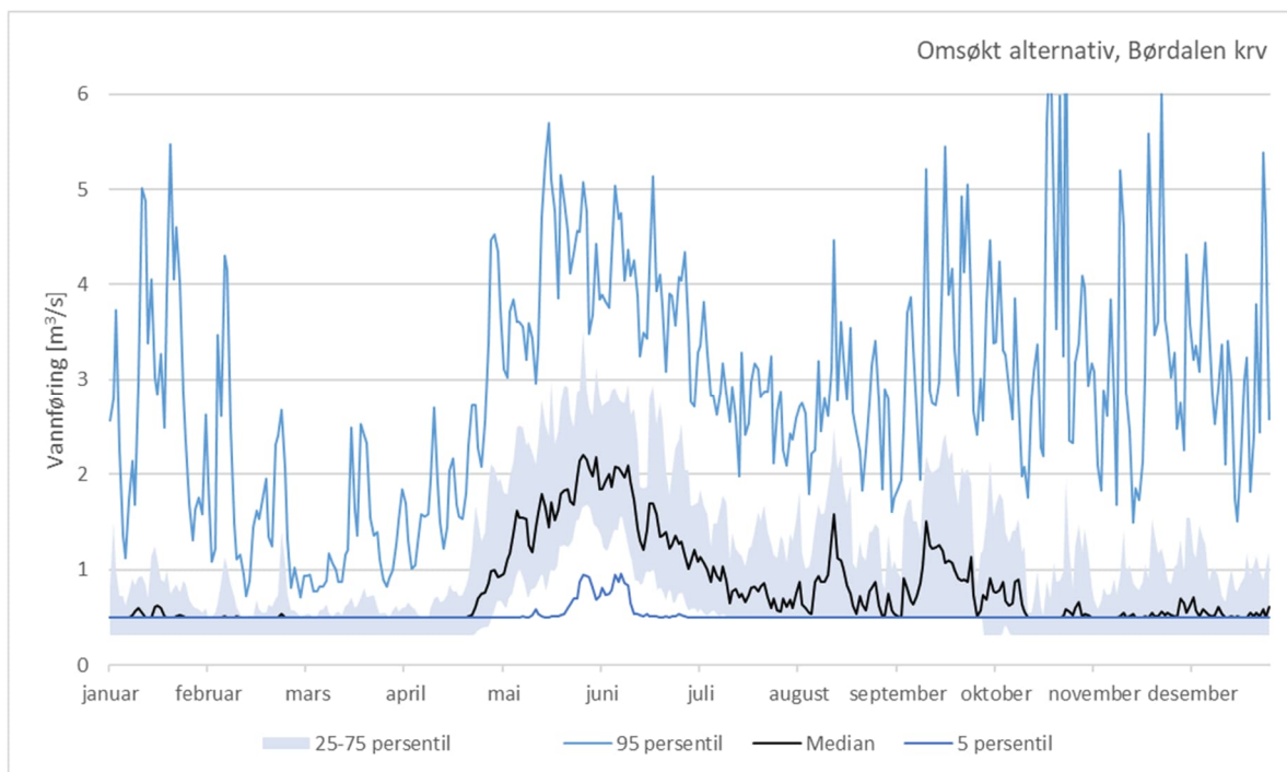
Figur 5-33 Persentilkurver ved Langeland, omsøkt alternativ
