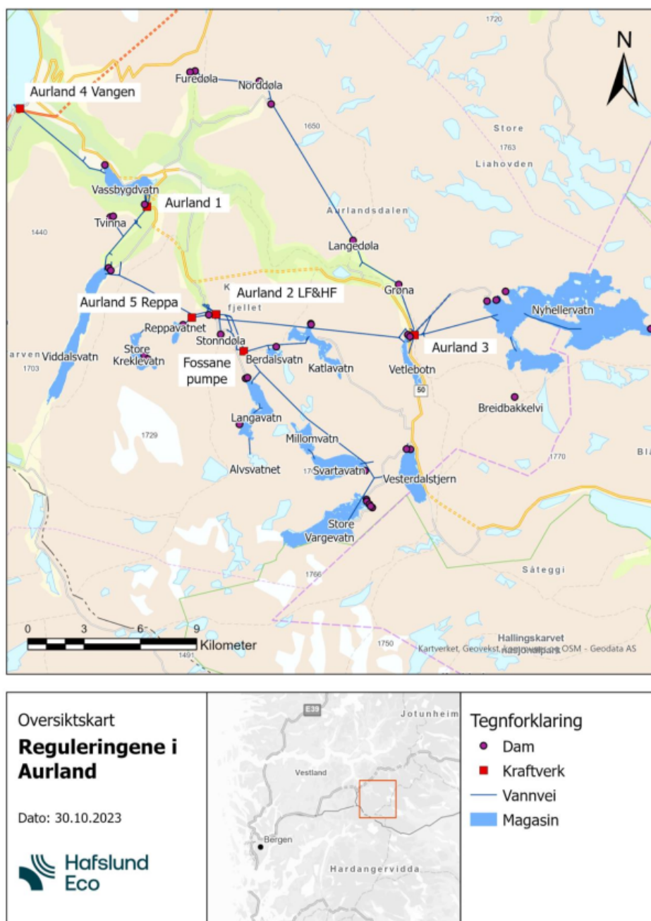
Fig.1. Oversiktskart over kraftverk, magasin, dammar og vatnvegar i reguleringssystemet i Aurland. (Henta frå revisjonsdokumentet)
