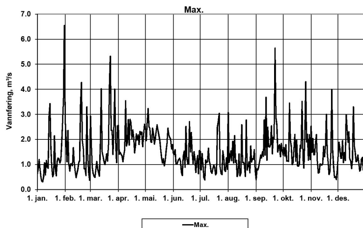
Figur 4. Plott som viser maksimumsvannføringer (døgndata). 14
