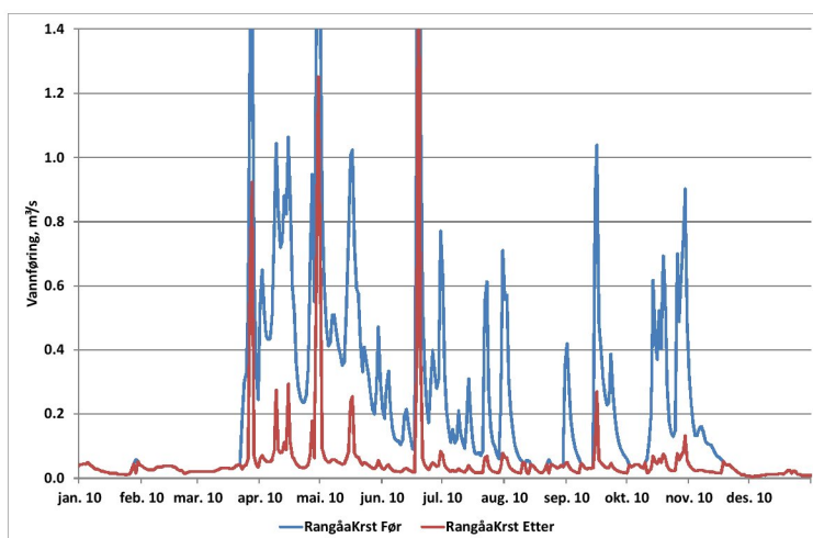
Figur 8. Plott som viser vannføringsvariasjoner i et tørt år like oppstrøms kraftstasjonen (før og etter utbygging). 18
