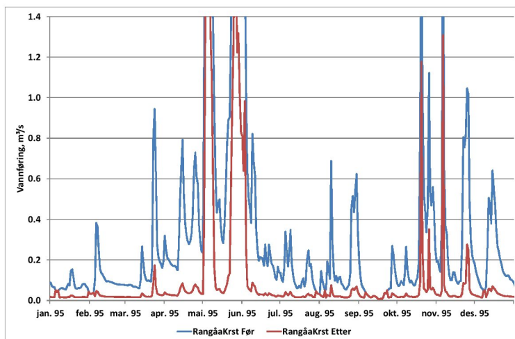
Figur 7. Plott som viser vannføringsvariasjoner i et middels år like oppstrøms kraftstasjonen (før og etter utbygging). 17
