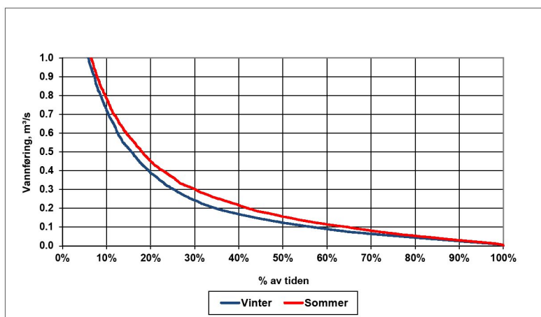
Figur 9. Varighetskurve for sommer- og vintersesongen (1/5 – 30/9).
