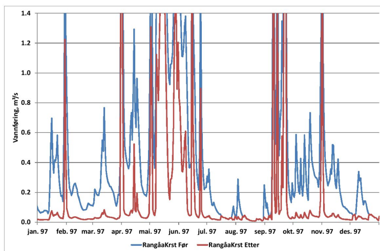
Figur 6. Plott som viser vannføringsvariasjoner i et fuktig år like oppstrøms kraftstasjonen (før og etter utbygging). 16
