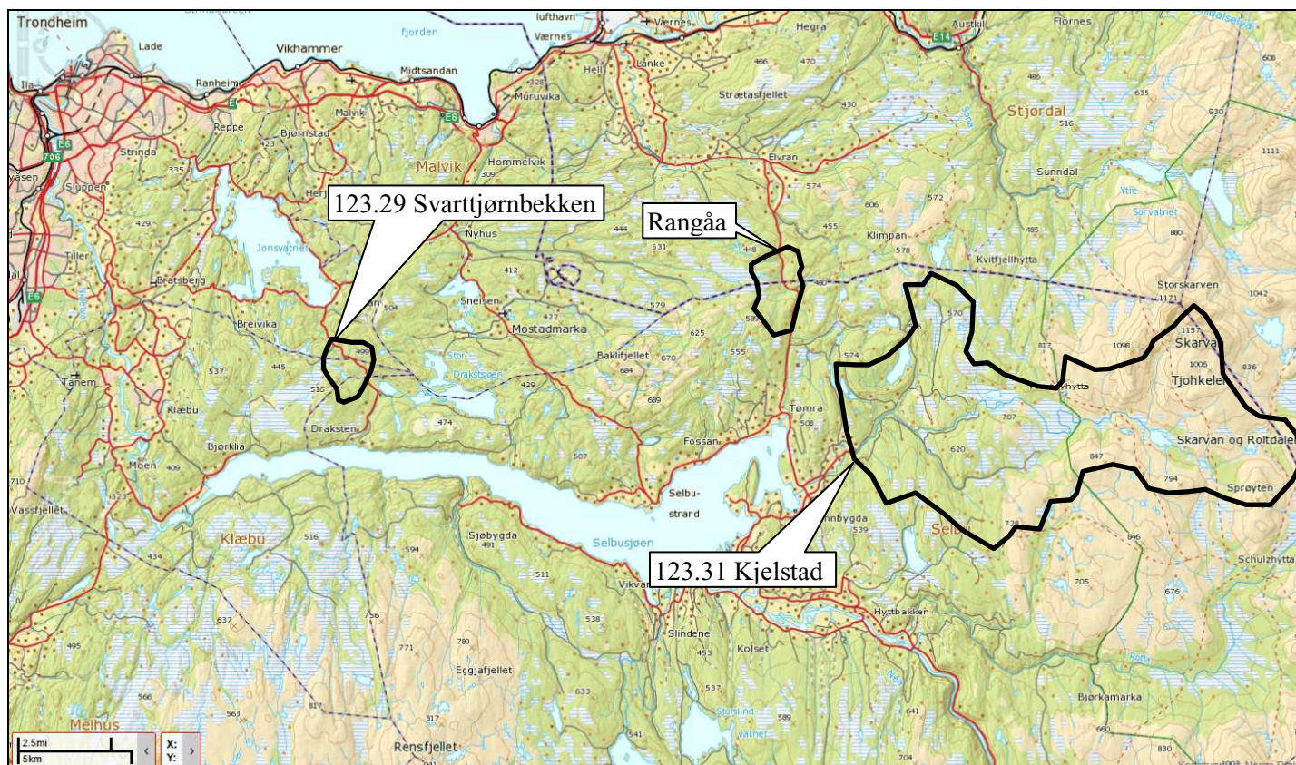
Figur 2. Kart med inntegnet nedbørfelt til kraftverket og til benyttet sammenligningsstasjon. Kommentarer ved behov.
