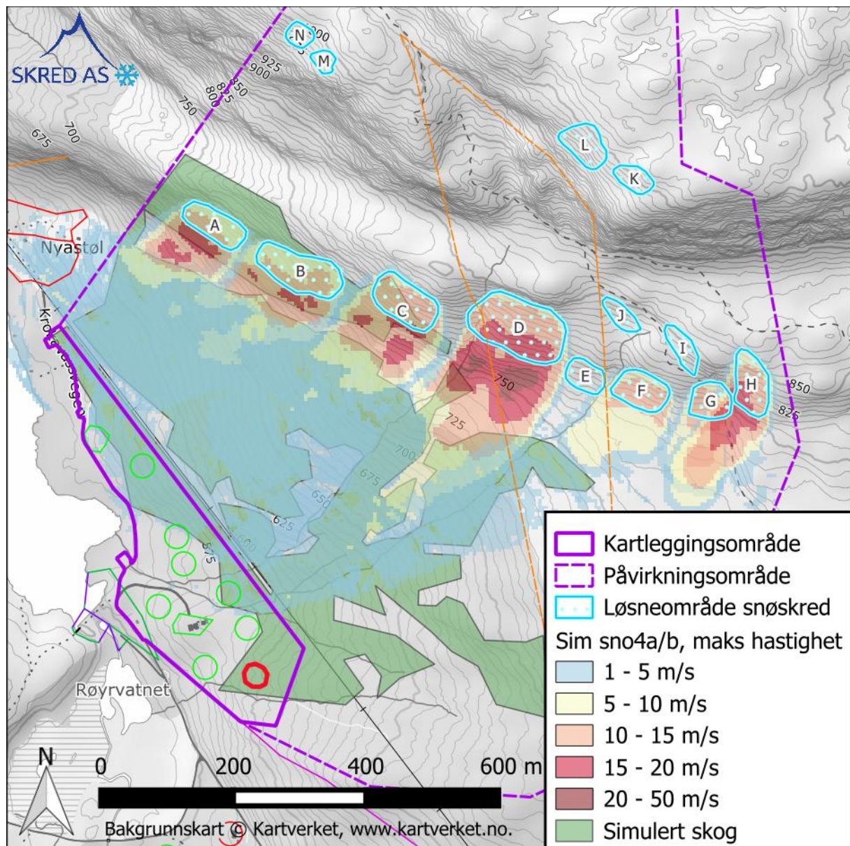
Figur 12: Eksempel på simulering (Sim sno4a/b) med identisk inngangsverdier som i Figur 11, men med skog. Resultatet viser kortere utløp og betraktelig lavere skredhastigheter. Snøen som når tomtene skyldes numerisk sig i simuleringsresultatet og gir urealistisk lange utløp med lave hastigheter over tid etter at snømassene er bremsset opp av skogen. Samtlige tomter ligger dermed trygt nok med tanke på snøskred. Løснеområde A og B er vurdert å ha en årlig løsnestannsynlighet mindre enn 1/1000 med skog, og kan ses vekk ifra.
