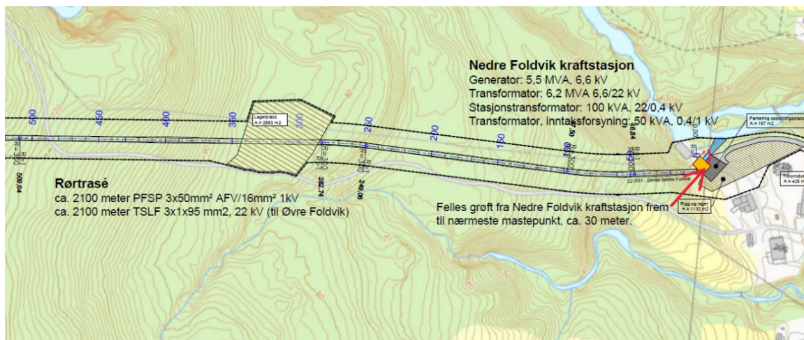
Figur 2: Detaljkart for Nedre Foldvik kraftverk der rød strek angir den ca. 30 meter lange jordkabelen frem til tilknytningspunkt i overliggende nett tilhørende Noranett.
