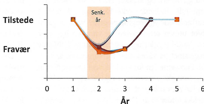
Figur 7. Restitueringsperiode for skjoldkrepsbestandar etter eit spesielt senkingsår i fem høgfjellsmagasin. Skjoldkreps treng 1–2 år med normal fylling før den på ny kan påvisast som næring for aure. (Etter Brabrand 2010.)
