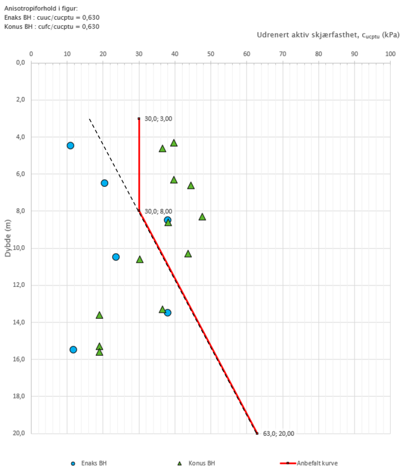
Figur 2 Designprofil for Cu basert på laboratorieundersøkelser i borhull 16230_2. SHANSEP-linjen er illustrert med stiplet linje.
