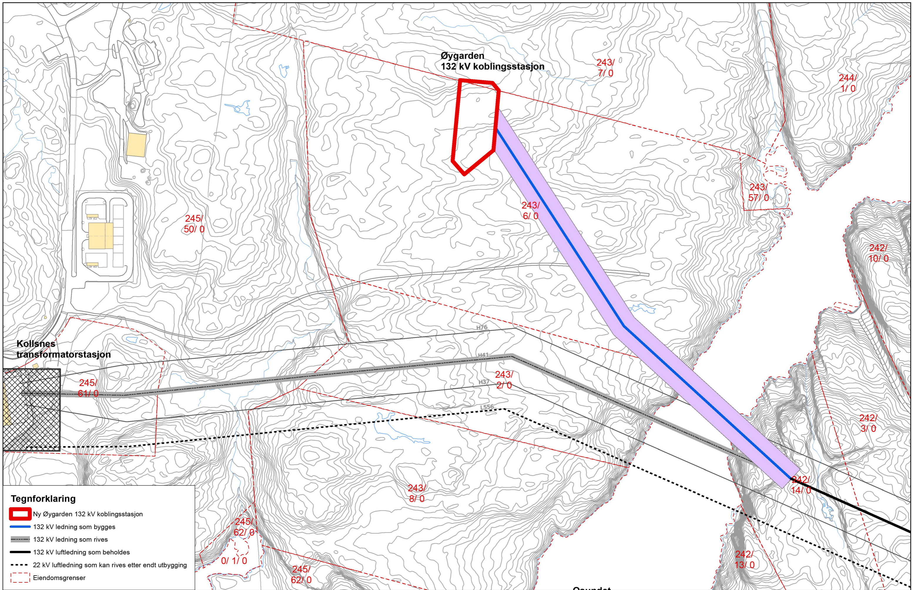
Detaljkart Øygarden 132 kV koblingsstasjon med omlegging av 132 kV luftledninger
