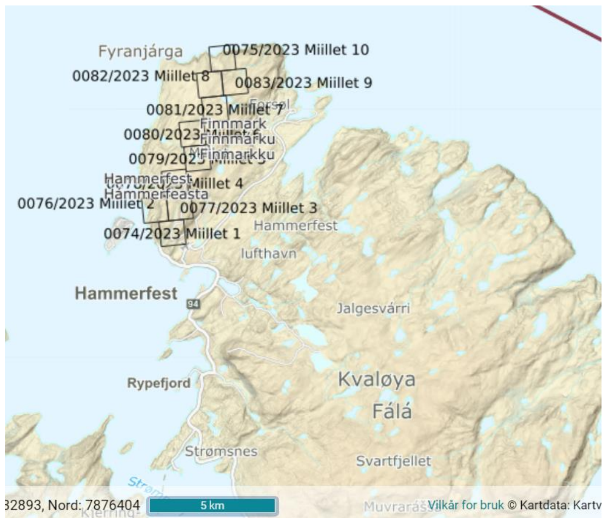
Figur 5-2. Kartutsnittet som viser bergrettigheter (sorte ruter)-. Kilde: DMFs kart.
