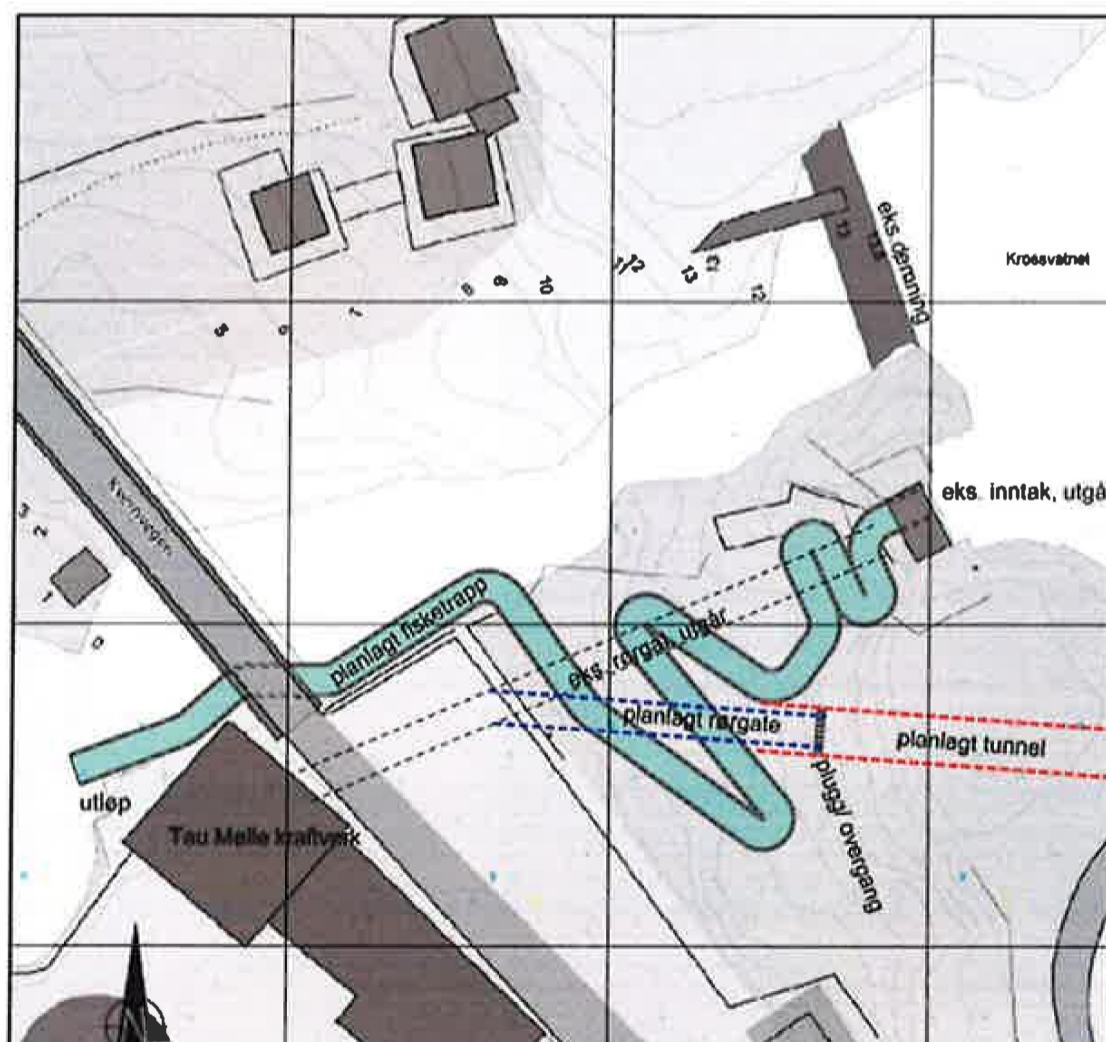
Figur 20: planlagt fisketrapp alternativ 1, helning 1:8
