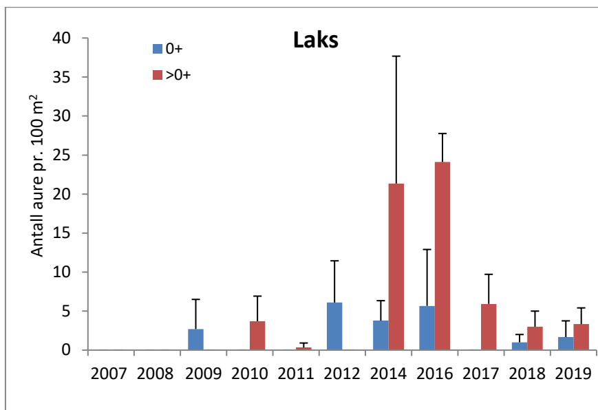
Figur 39. Gjennomsnittlige tettheter av ungfisk av laks i Austrepollelva ved innsamlingene i 2007-2019. Det er skilt mellom årsunger (0+) og eldre ungfisk (> 0+). I 2013 og 2015 ble det ikke utført ungfiskundersøkelser.
