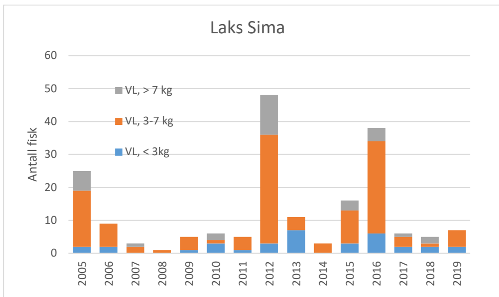
Figur 11. Antall sjøåure (øverst) og laks (nederst) i ulike størrelsesgrupper observert ved drivtelling i Sima i perioden 2005-2019.
