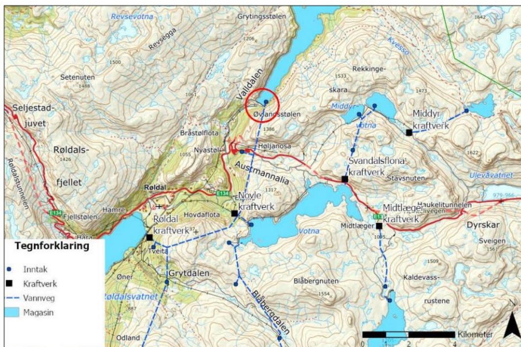
Figur 1. Kart fra detaljplan over dam Valldalens plassering (rød sirkel) nord for E134.
