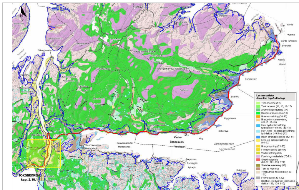
Figur 62: Utlipp av NGUs løsmassekart [5] som viser plasseringen av Karasjok-Bugøfjord, her strekningen Polmak - Vardø på E75. Marin grense er vist med blå stiplet linje. Kartlagt målestokk 1: 500 000.
