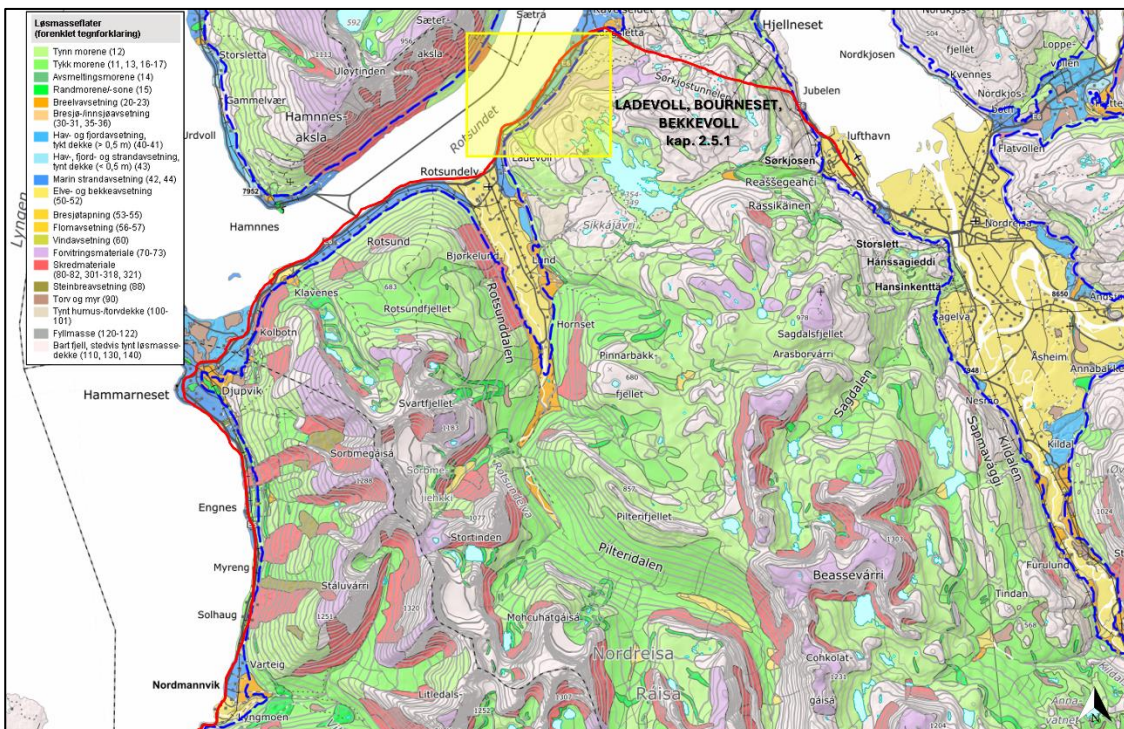
Figur 36: Utklipp av NGUs løsmassekart [5] som viser plasseringen av E6 Nordkjösbotn til Sørkjosen, her strekningen Nordmannvik - Sørkjosen. Marin grense er vist med blå stiplede linje. Kartlagt målestokk 1: 250 000 til 1:500 000. Plassering av Ladevoll, Bourneset og Bekkevoll er angitt med gult rektangel.
