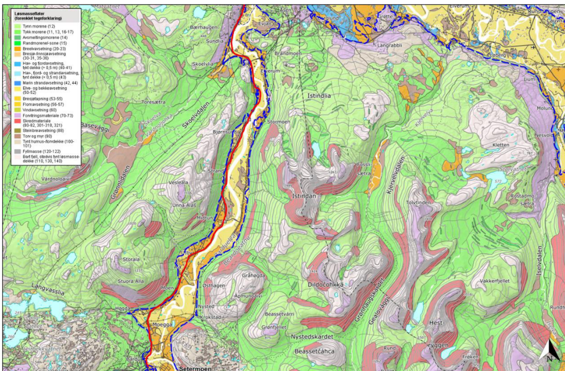
Figur 21: Utklipp av NGUs løsmassekart [5] som viser plasseringen av E6 Narvik til Tromsø, her Setermoen - Brandmoen . Marin grense er vist med blå stiplede linje. Kartlagt målestokk 1: 20 000 til 1:250 000.
