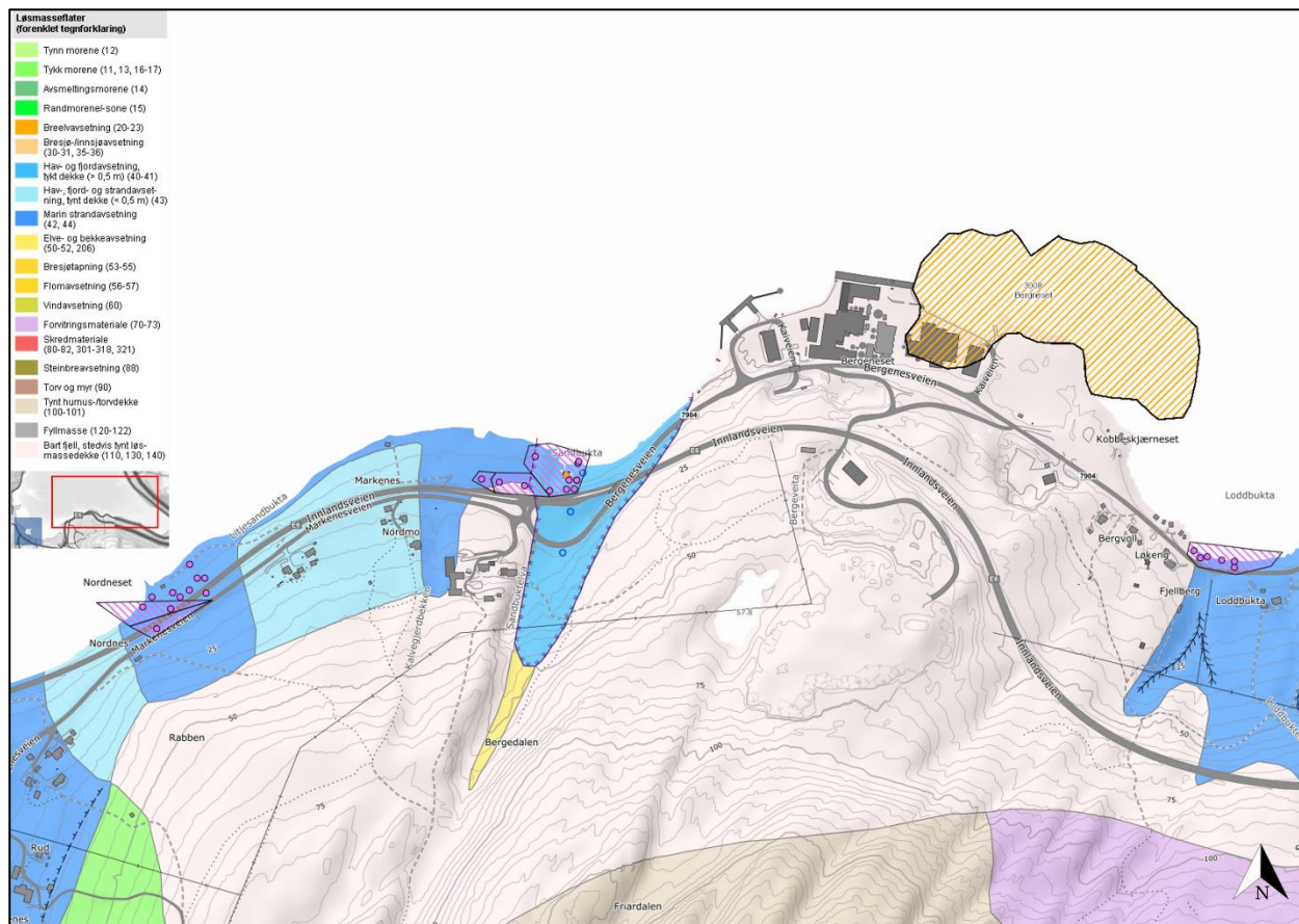
Figur 28: Utklipp fra NGU Løsmasser [5] som viser SVV-kvikkleirepunkter kartlagt ved Marken i Balsfjord kommune. Sandbukt sone og Nordneset sone ligger i et område karakterisert av hav-, fjord- og sandavsetninger (blå farge), før overgang til fjell i sør. Kartlagt målestokk: 1: 20 000.
