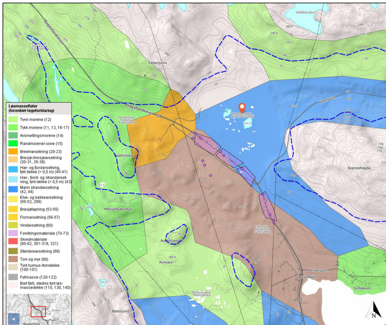
Figur 71: Utklipp fra NGU Løsmasser [5] som viser SVV-kvikkleirepunkter kartlagt ved Sopnesmyra i Sør-Varanger kommune. Sopnesmyra sone, Haukelva vest og øst soner ligger i område karakterisert av hav-, fjord- og sandavsetninger (blå farge), samt myr (brun farge), med en overgang til tynne og tykkere morenelag (henholdsvis lys grønn og grønn farge). Et område er også kartlagt som breelavsetninger. Det er også på begge sider av veien kartlagt områder med bart fjell (lysebrun/beige farge), slik som Sopneshøgda og Balsanjunnas. Marin grense er lagt inn som blå stiplet linje. Kartlagt målestokk: 1: 500 000.
