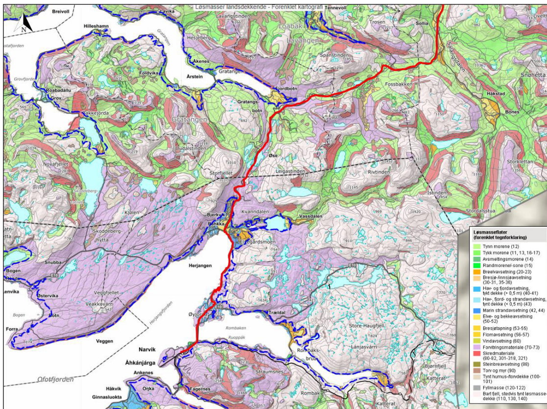
Figur 19: Utklipp av NGUs løsmassekart [5] som viser plasseringen av E6 Narvik til Tromsø, her strekningen Narvik - Sollia. Marin grense er vist med blå stiplede linje. Kartlagt målestokk 1:100 000.
