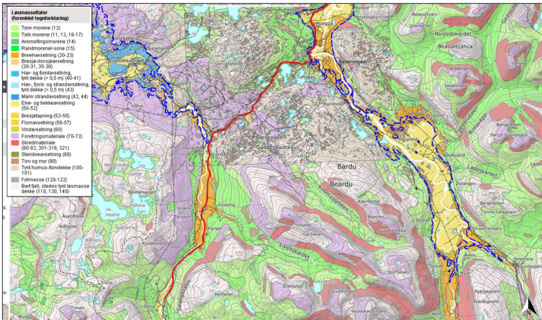
Figur 20: Utklipp av NGUs løsmassekart [5] som viser plasseringen av E6 Narvik til Tromsø, her strekningen Sollia – Setermoen. Marin grense er vist med blå stiplede linje. Kartlagt målestokk 1: 20 000 til 1:250 000.
