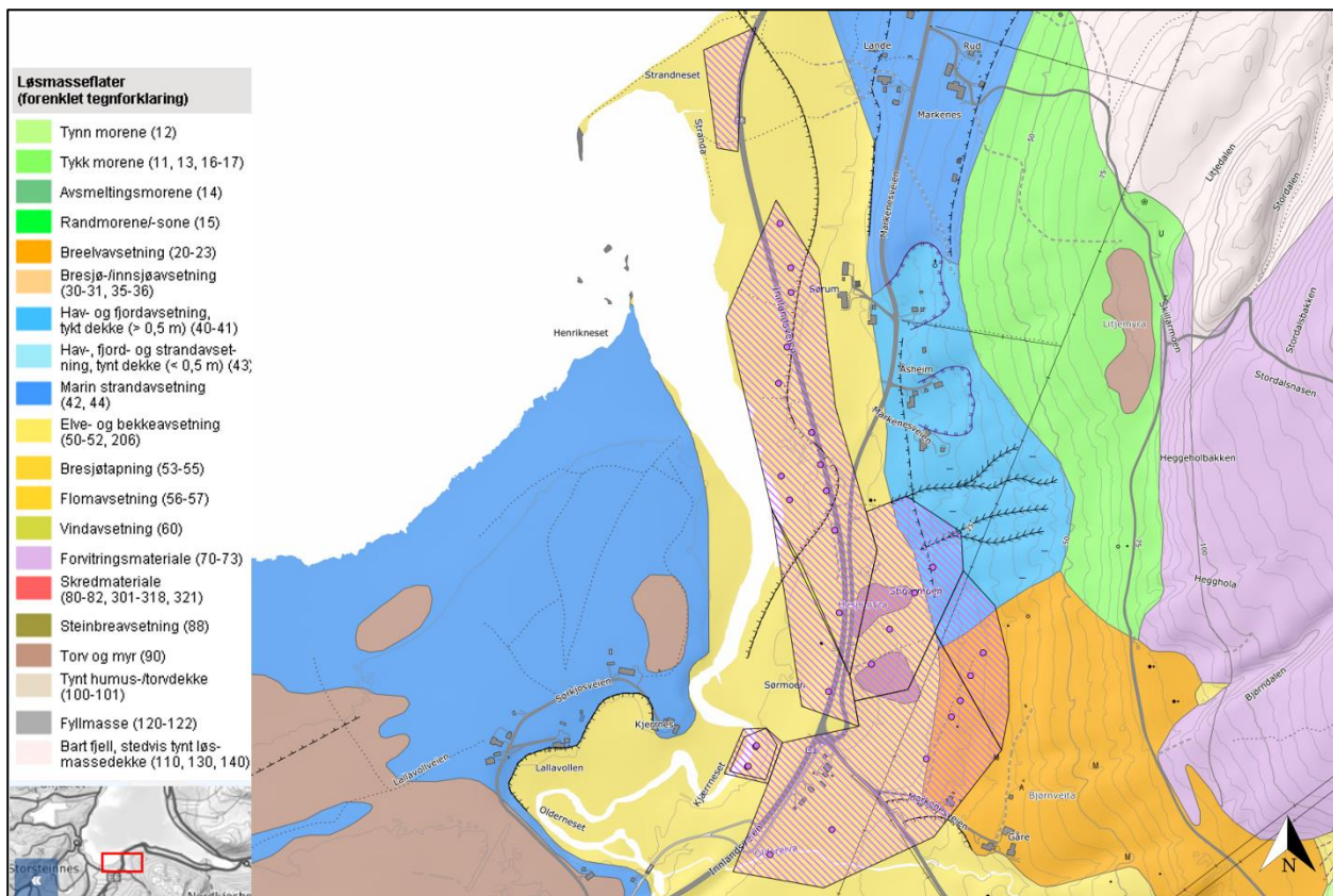
Figur 26: Utklipp fra NGU Løsmasser [5] som viser SVV-kvikkleirepunkter kartlagt ved Bjørnveita i Balsfjord kommune. Tømmerelv sone og Bjørnveita sone ligger i et område kartlagt i hovedsak som elve- og bekkeavsetninger (gul farge), marine strandavsetninger (mørkeblå farge) og breekvassetninger (oransje farge). Kartlagt målestokk: 1:20 000.
