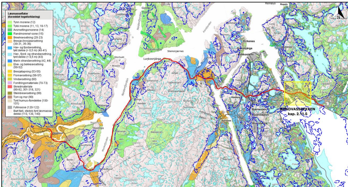
Figur 79: Utklipp av NGUs løsmassekart [5] som viser plasseringen av strekningen Bugøyfjord – Storskog, her strekningen Neiden – Storskog på E105. Marin grense er vist med blå stiplede linje. Kartlagt målestokk 1:50 000 til 1:500 000. Plassering av området Rundvassbekken er angitt med gult rektangel.
