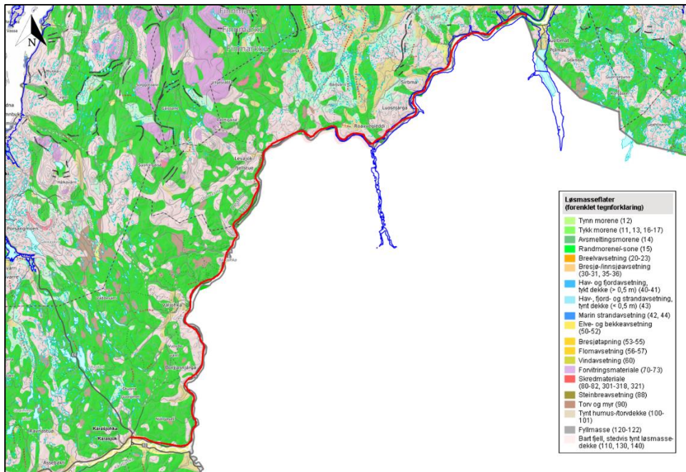
Figur 61: Utlipp av NGUs løsmassekart [5] som viser plasseringen av Karasjok-Bugøfjord, her strekningen Karasjok – Polmak på riksveg 92. Marin grense er vist med blå stiplet linje. Kartlagt målestokk 1: 250 000.
