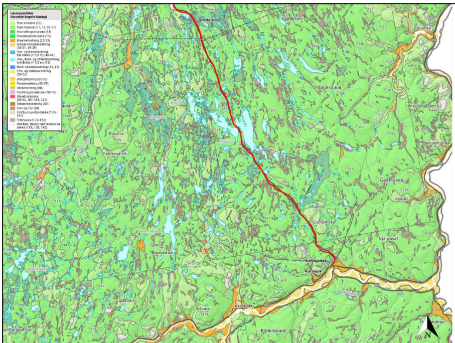
Figur 59: Utklipp av NGUs løsmassekart [5] som viser plasseringen av E6 Lakselv til Karasjok, her strekningen Grøtterud - Karasjok. Marin grense er vist med blå stiplede linje. Kartlagt målestokk 1: 250 000.
