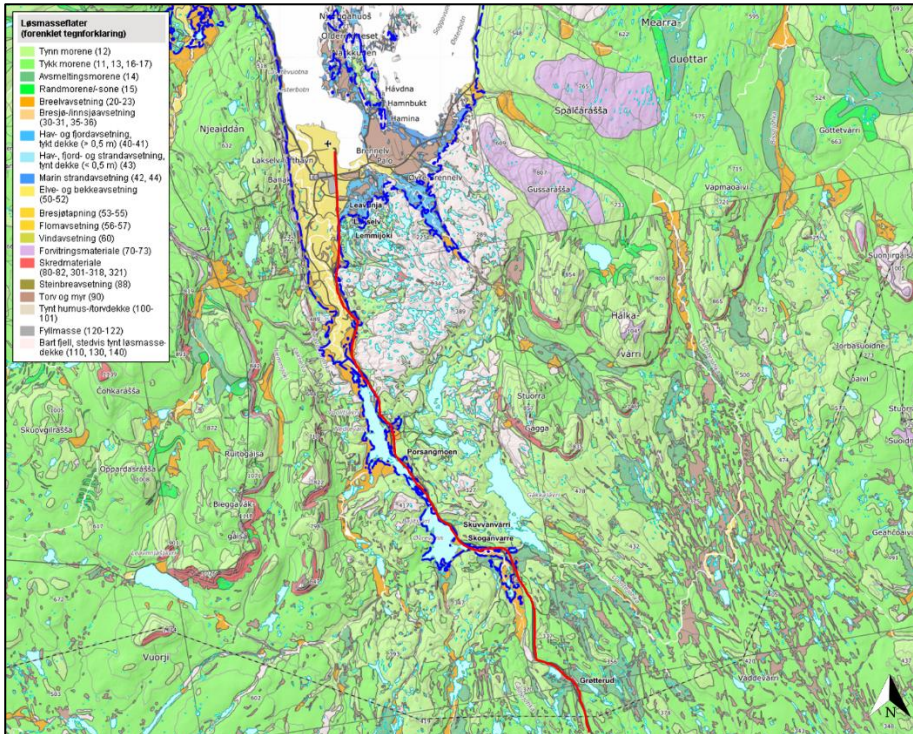
Figur 58: Utklipp av NGUs løsmassekart [5] som viser plasseringen av E6 Lakselv til Karasjok, her strekningen Lakselv - Grøtterud. Marin grense er vist med blå stiplede linje. Kartlagt målestokk 1: 250 000.
