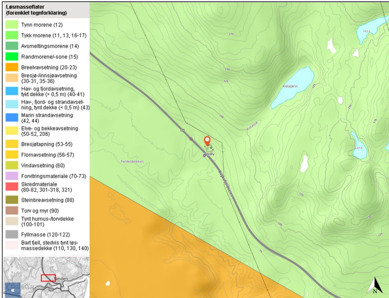
Figur 89: Utlipp fra NGU Løsmasser [5] som viser SVV-kvikkleirepunkter kartlagt ved Ferdly i Sør-Varanger kommune. Løsmassene i området er kartlagt som tynt morenemateriale over berggrunn (lysegrønn farge), og breelavsetninger (oransje farge). Kartlagt målestokk: 1:500 000.
