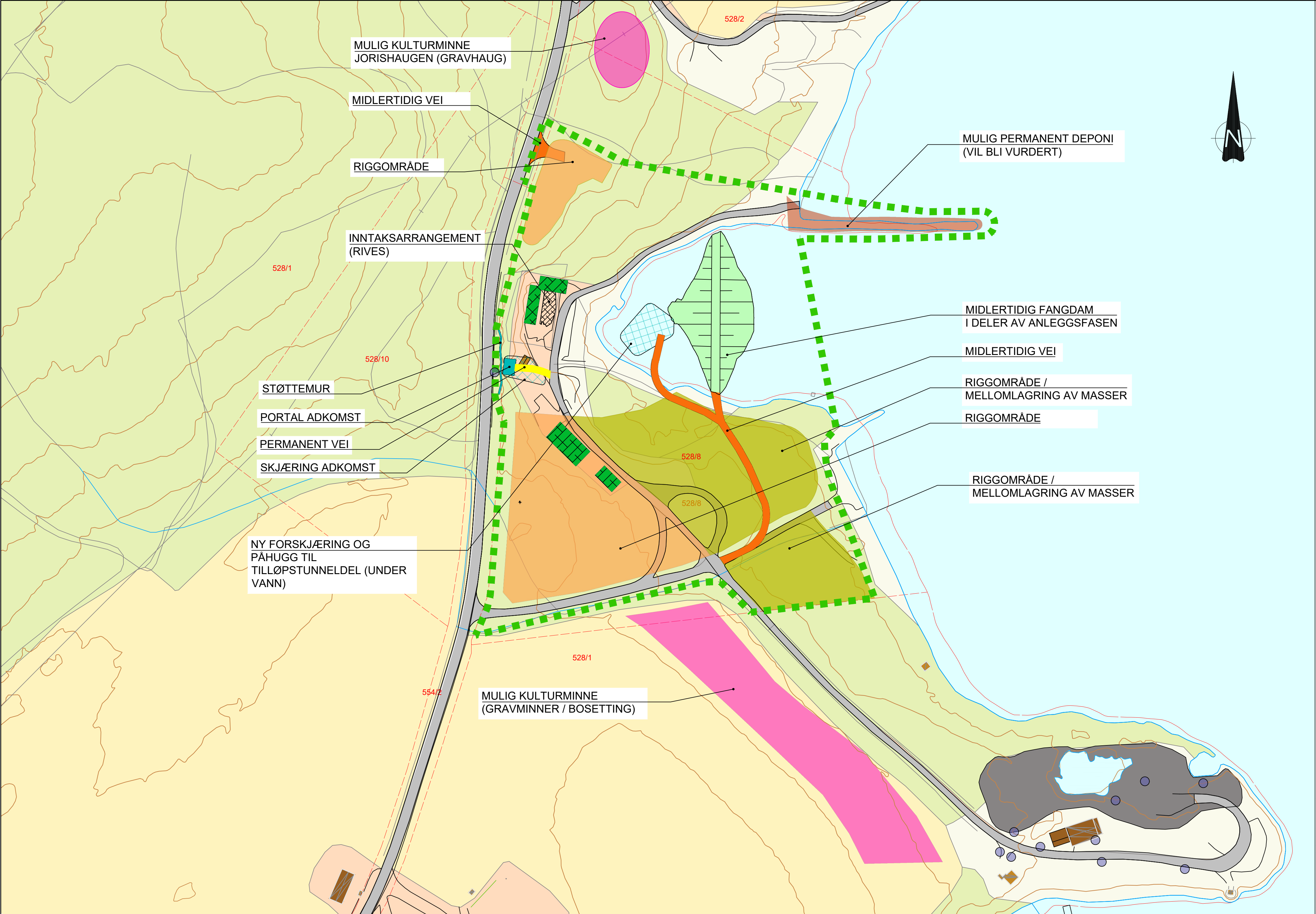
PLAN INNTAKSOMRÅDE 1:1000
