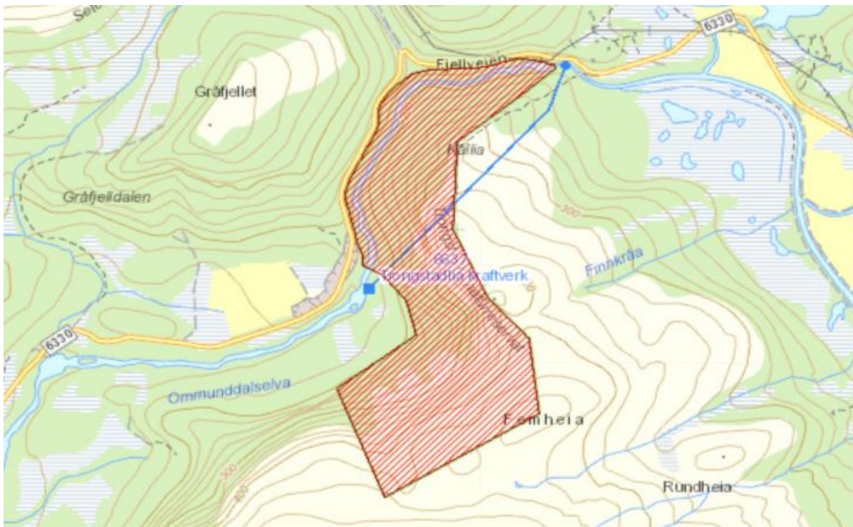
Figur 1: Kart over Trongstadlia naturreservat og planlagt inntak, vannvei og kraftverk (Kilde: NVE Atlas)
