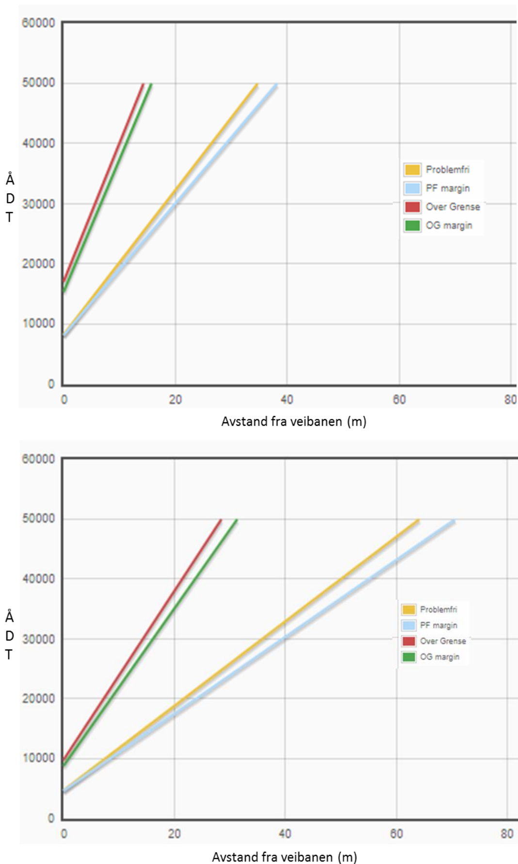
Figur 5.1. Trafikknomogram for PM10 beregnet for en tungtrafikkandel på 10%, piggdekkandel på 30% og kjørehastighet på 60 km/t (øverst) og 80 km/t (nederst). Oransje og rød linje viser grenseverdiene på hhv. 35 og 50 \mu\text{g}/\text{m}^3 for gul og rød sone etter T-1520, mens blå og grønn linje viser overskridelse av disse.
