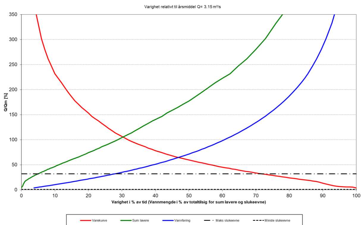
Varighetskurve, Voldafossen ved inntak, 1993 - 2022
