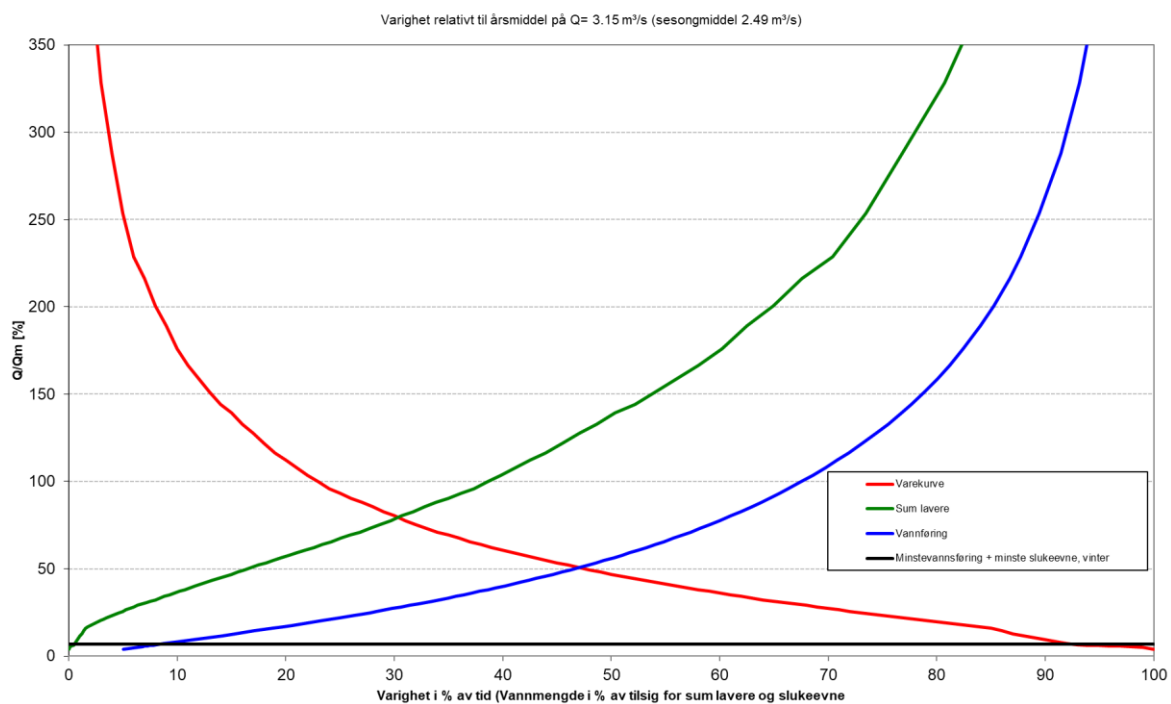
Varighetskurve vinter (1/10-30/4), Voldafossen ved inntak, 1993 - 2022
