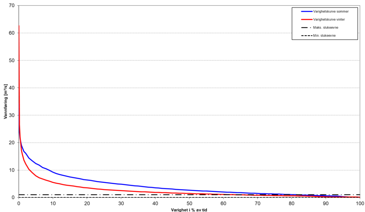
Varighetskurver, Voldafossen ved inntak, 1993 - 2022
