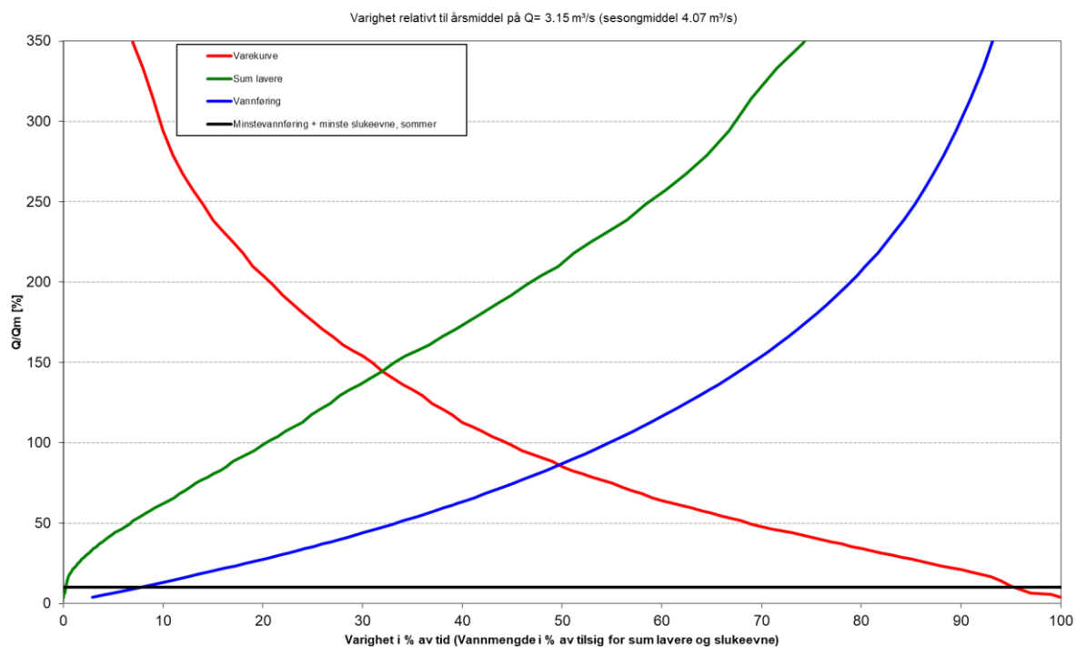
Varighetskurve sommer (1/5-30/9), Voldafossen ved inntak, 1993 - 2022
