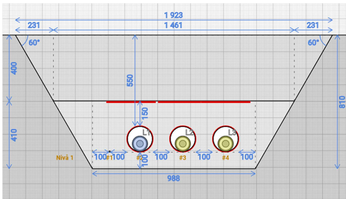
Figur 1. Standard grøftesnitt for kabeltrasé.
