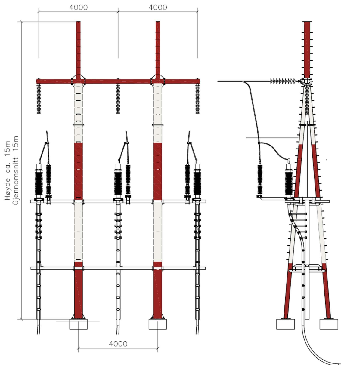
Figur 7. Kabelendemast sett forfra og fra siden. Kabelendemasten må merkes som luftfartshinder dersom den plasseres ved Tveitovegen. Plassert ved transformatorstasjonen blir kabelendemasten malt brun.
