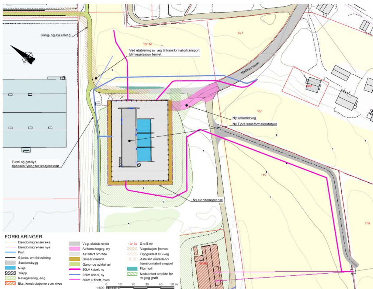
Figur 4-1 Utsnitt situasjonsplan
